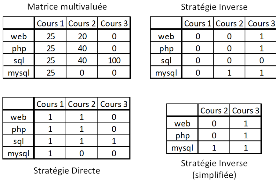
FIG. 2.5 – Exemple d’application des stratégies directe et inverse
