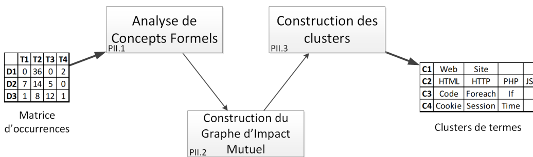
FIG. 3.10 – Les étapes de la phase d'analyse structurelle
