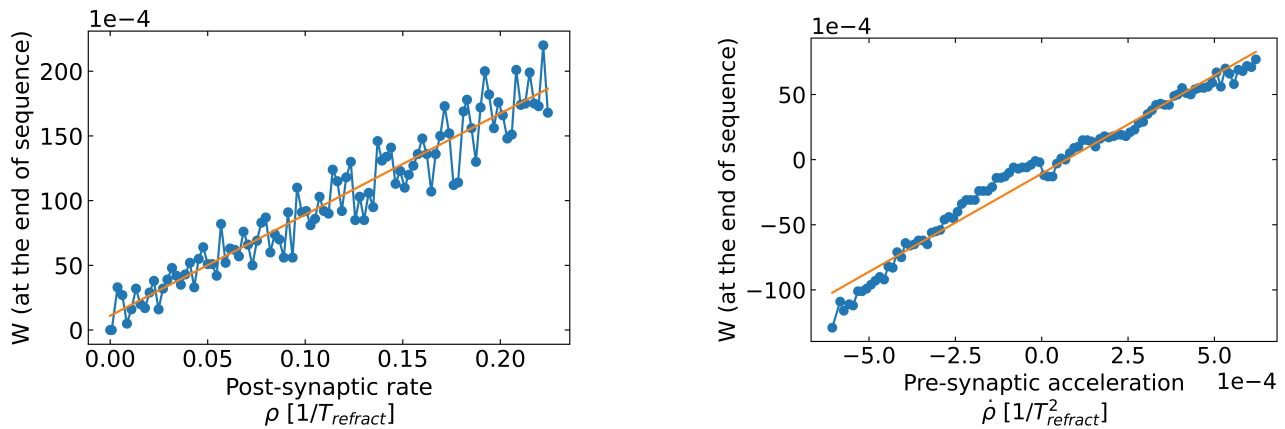
(a) Dépendance de la modification du poids synaptique à la fréquence avec une durée d'impulsion d'une durée de 100dt .
