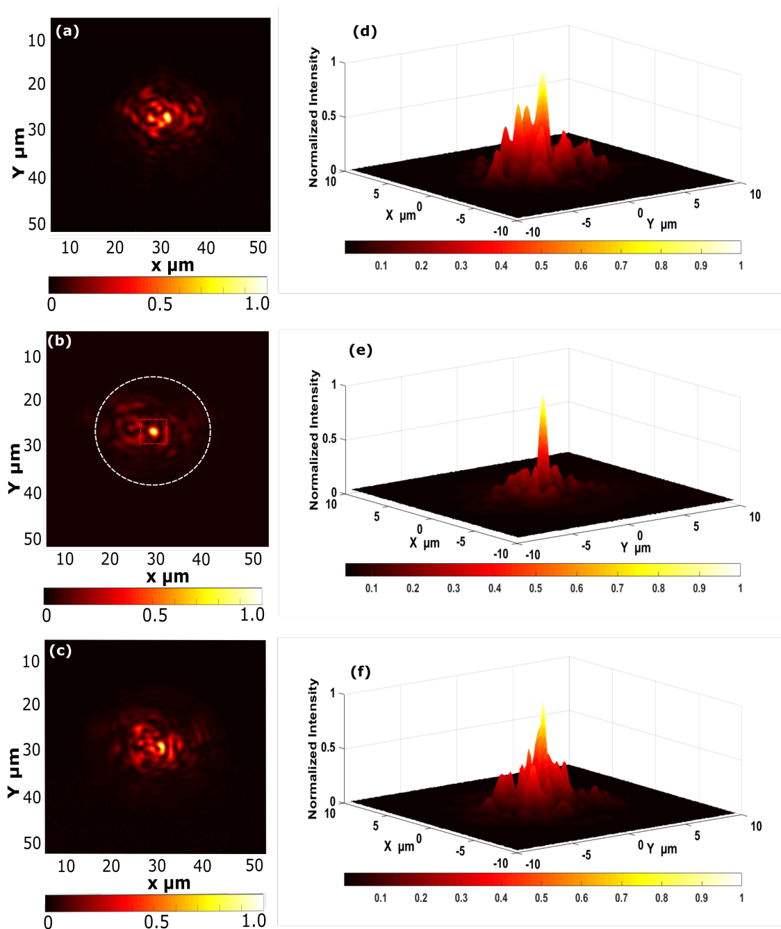
FIGURE 3.22 – Distribution d'intensité mesurée en sortie de la fibre 50/125 avec embout en (a)(d) Z = +8 \mu\text{m} ; (b)(e) Z = 0 et (c)(f) Z = -19 \mu\text{m} .
