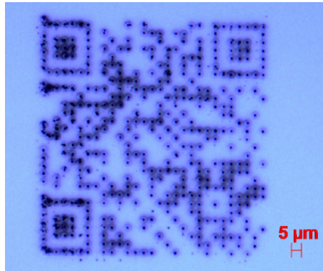
FIGURE 1.15 – Matrice de QR code ( 110 \times 110 \mu\text{m} ) sur silicium. Chaque marque gravée a un diamètre d'environ 1,3 \pm 0,6 \mu\text{m} . Une énergie d'impulsion de 17 \mu\text{J} . 35 impulsions pour chaque gravure par jet photonique en sortie d'une fibre 100/140 [68].
