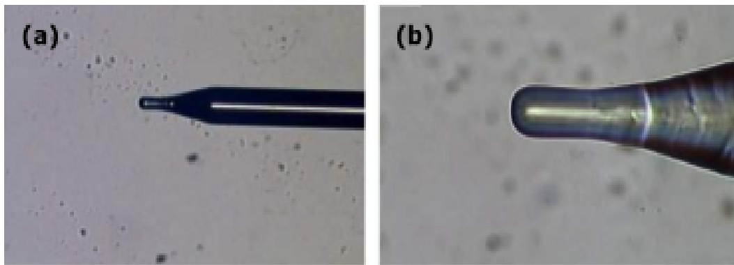
FIGURE 1.21 – Microlentilles avec des rayons de (a) 10µm et (b) 20µm réalisée par la méthode attaque chimique et fusion thermique [83].
