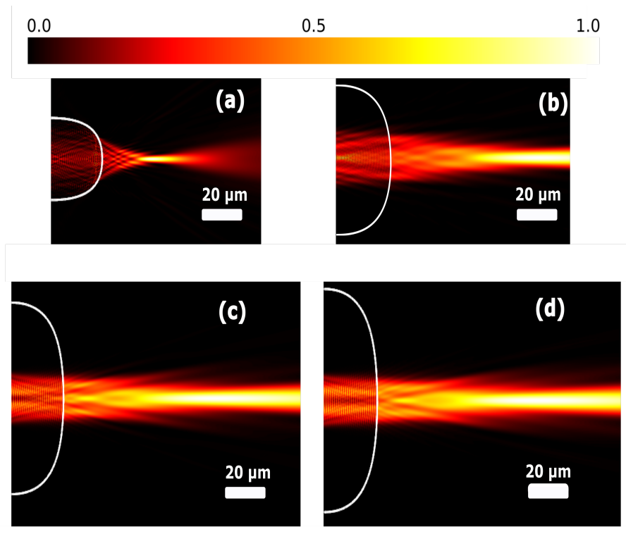
FIGURE 2.15 – Jet photonique (intensité |E^2| ) avec une fibre 20/125, ON de 0,22. Excitation par le mode fondamental. \lambda = 1064\text{nm} . h = 26 \mu\text{m} , W = 1,10 , (a) D = 30 \mu\text{m} , (b) D = 50 \mu\text{m} , (c) D = 70 \mu\text{m} , (d) D = 80 \mu\text{m} .
