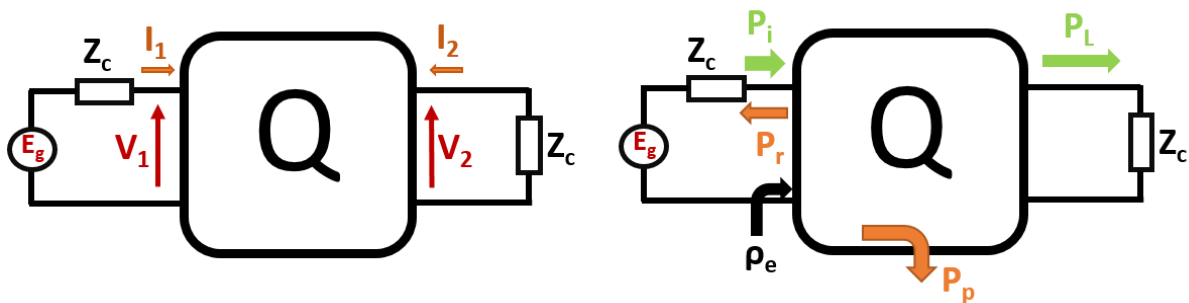
Figure 6: Représentation du filtre sous forme de quadripôle.
