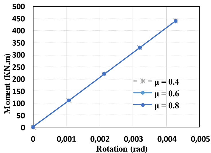
Figure 3.18 : Étude paramétrique sur le coefficient de frottement
