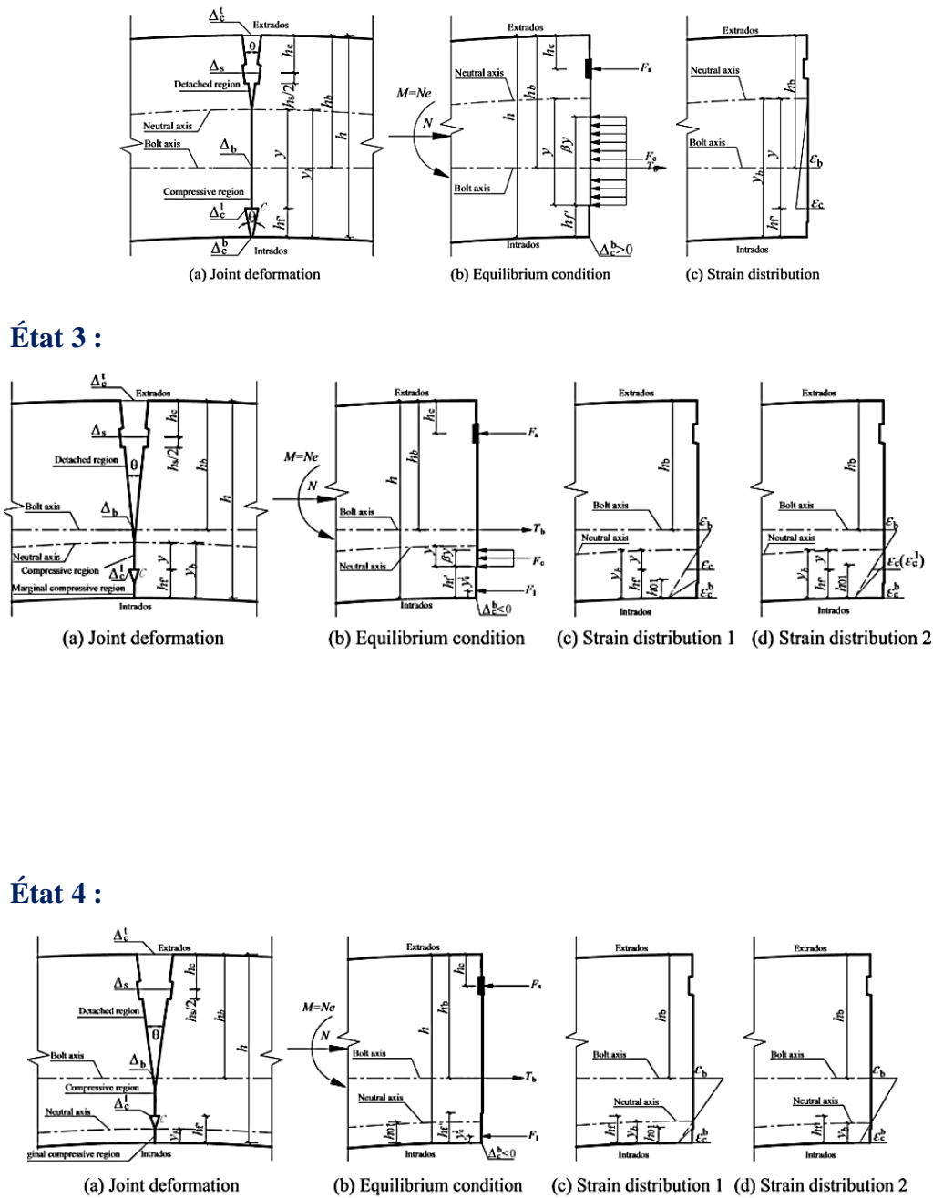
Figure 1.35: Différentes états de contrainte sous moment négatif lors des phases de chargement (Li et al. 2015).
