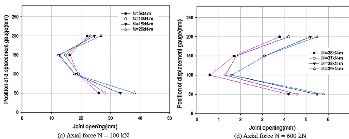
Figure 1.43: Relation entre l'ouverture du joint et le moment de flexion sous différentes forces axiales (Zuo et al. 2018).
