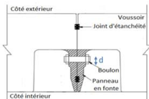
Figure 3.23 : Section de boulon.
