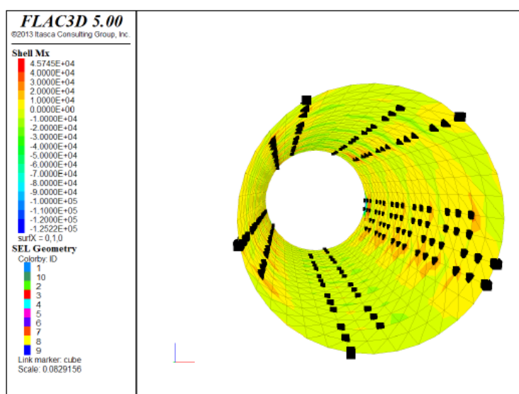
Figure 1.23: Joints segmentaires sous forme de liaison entre les éléments de coque
