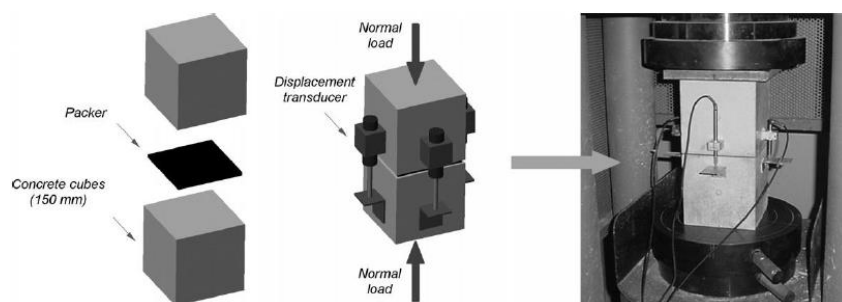
Figure 1.28: Configuration de l'essai à l'aide de blocs de béton (Cavalaro et al. 2011).
