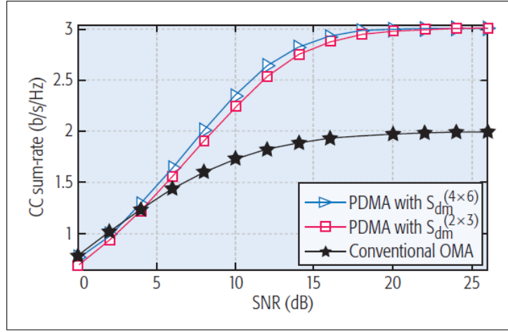
Figure 8 : Capacité « sum-rate » des schémas PDMA et comparaison avec les systèmes OMA
