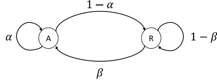
Figure 14: Diagramme de transition d'état du modèle de chaîne de Markov décrivant le comportement temporel du utilisateur.
