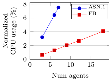
(a) Utilisation du CPU de FlexRIC.
