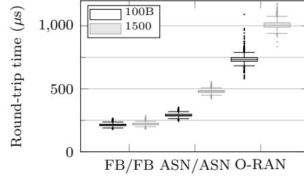
(b) RTT pour deux sauts vs. O-RAN RIC.
