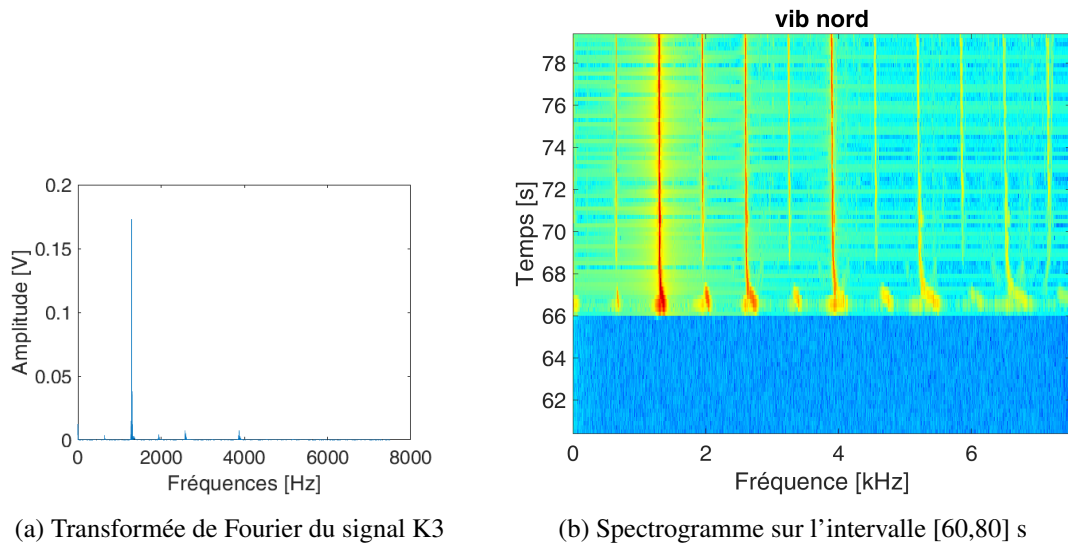
FIGURE 3.5 – Analyse fréquentielle du signal vibratoire pour un essai à 13 g/s
