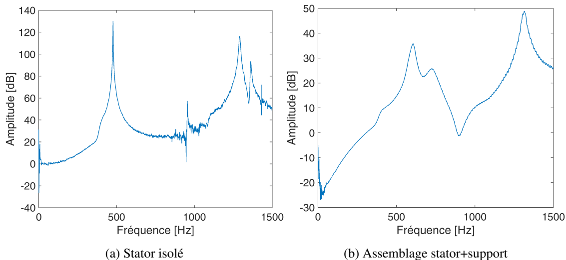
FIGURE 2.4 – Minotaur 1 : FRF des essais d'analyse modale en libre-libre
