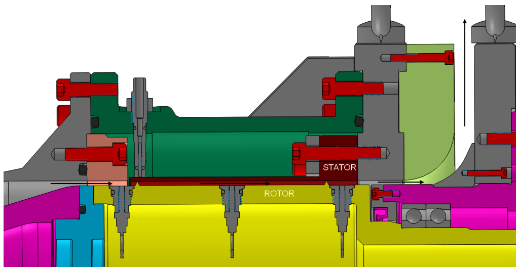
FIGURE 2.19 – Zoom sur le joint labyrinthe
