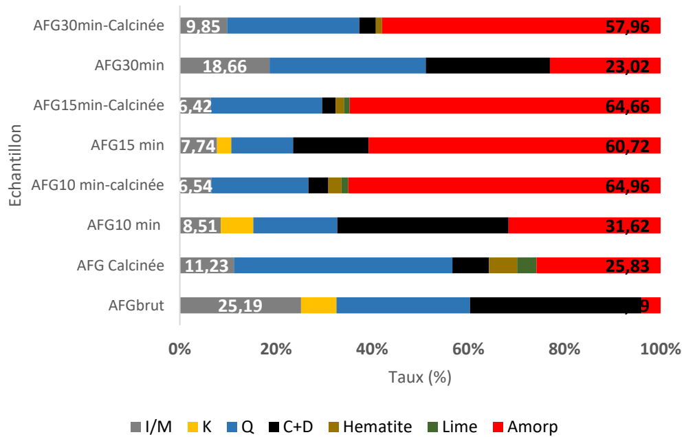
Figure III-11 : Quantification des phases cristallines et du taux d'amorphisation par la méthode de Rietveld.
