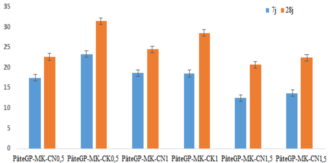
Figure IV-15 : Résistance à la compression des pâtes géopolymères à base de MK à 7 et 28 jours de séchage.
