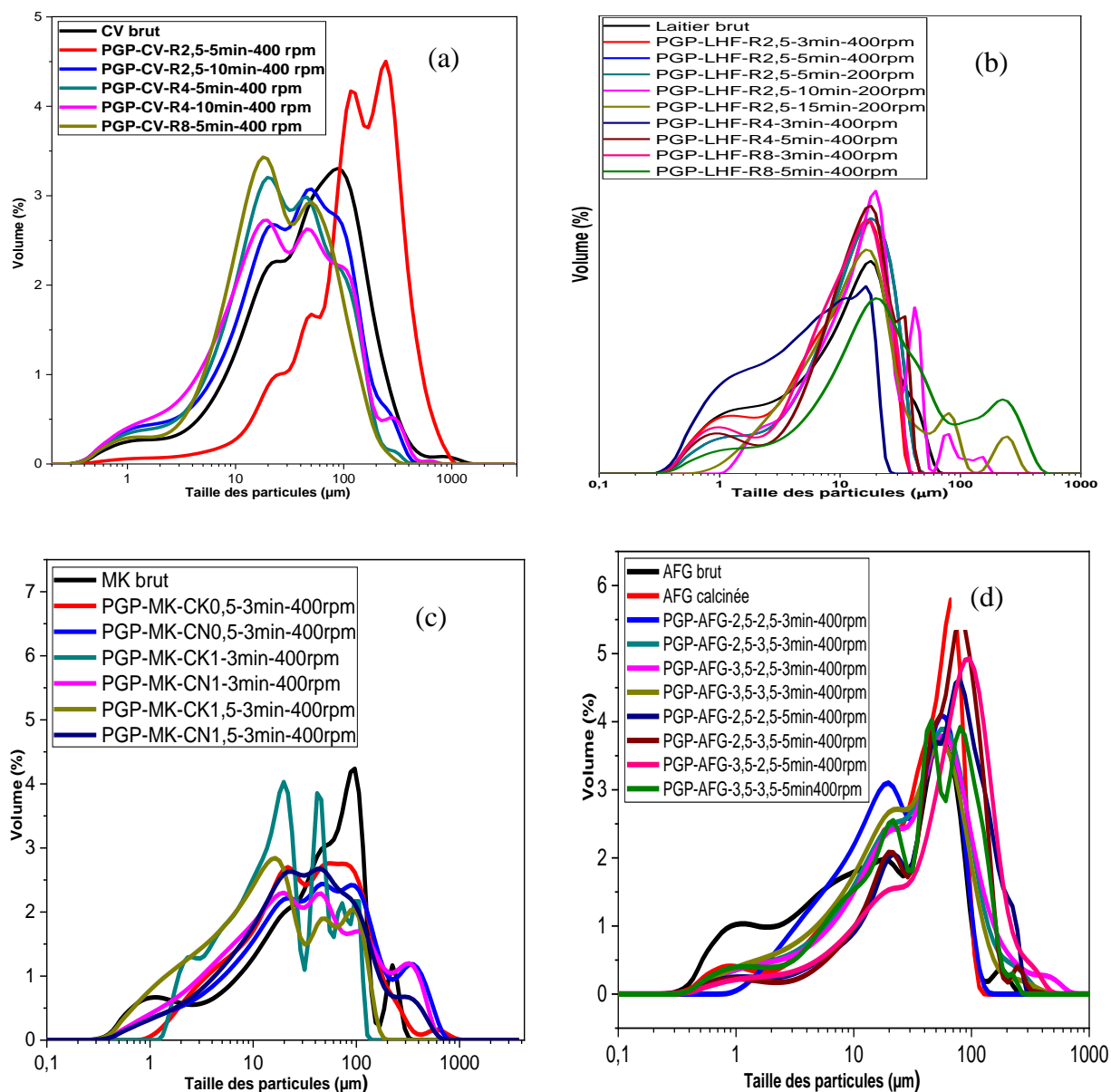
Figure III-1 : Granulométrie laser des poudres pré-géopolymères à base des différents précurseurs.
