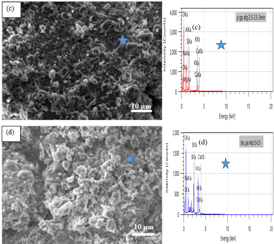
Figure IV-12 : Micrographies avec analyse EDX des échantillons (a) AFG brute, (b) AFG brute calcinée, (c) PâteGP-AFG-R2,5-2,5-3min-400rpm, (d) PâteGP-AFG-R 3,5-2,5-3min-400rpm.
