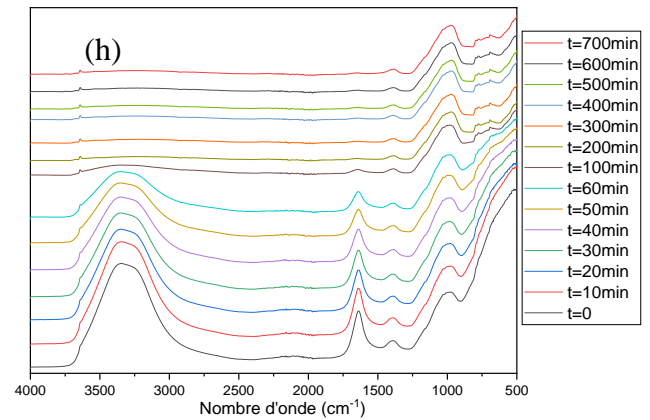
PâteGP-MK-CK0,5-3min-400rpm
