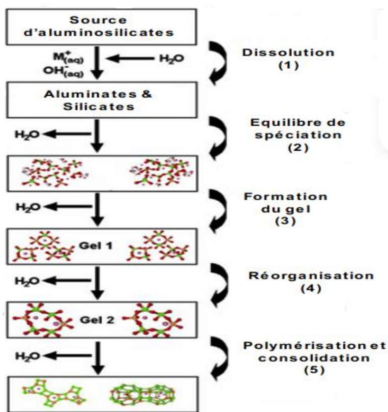
Figure I-4 : Modèle de géopolymérisation proposé par Duxson et al. [15].
