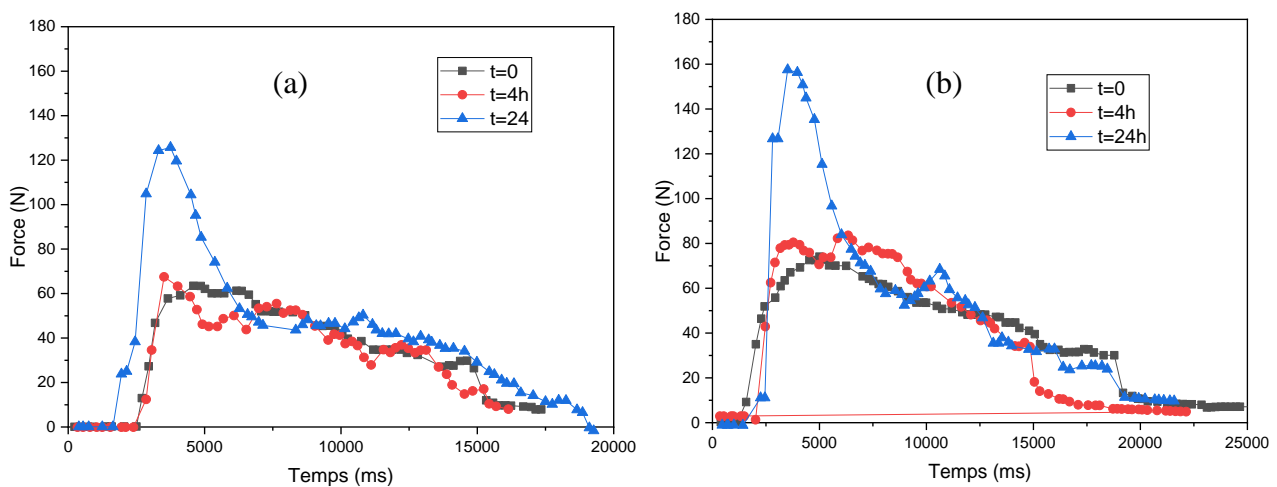
Figure V-8 : Résultats des essais de maniabilité pour les enrobés à l'émulsion avec le filler (a) calcaire et (b) PGP-LHF.
