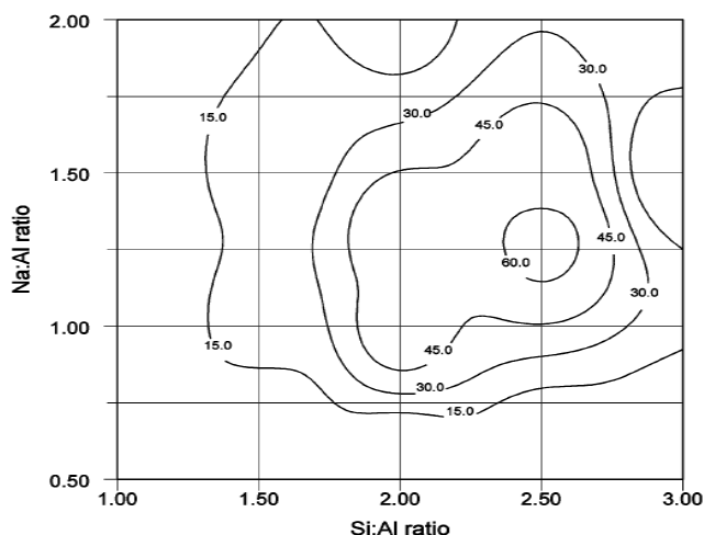
Figure I-18 : Contours de résistance à la compression pour les Na-géopolymères [100].
