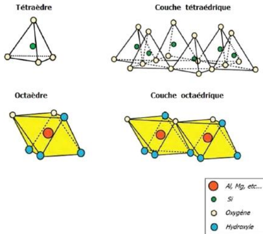
Figure I-10 : Structures octaédrique et tétraédrique des couches d'argiles [54].
