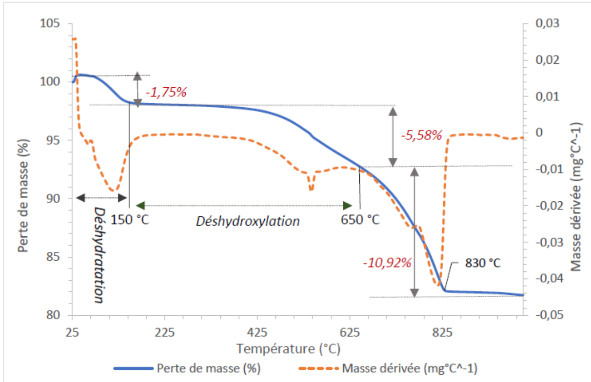
Figure A4 : Analyse thermogravimétrique de l'argile de Fès.
