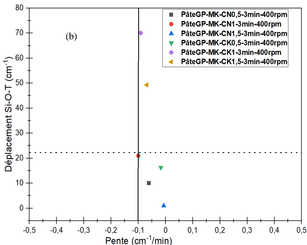
Figure IV-7 : Zones géopolymères pour les géopolymères à base de CV (a) et MK (b).
