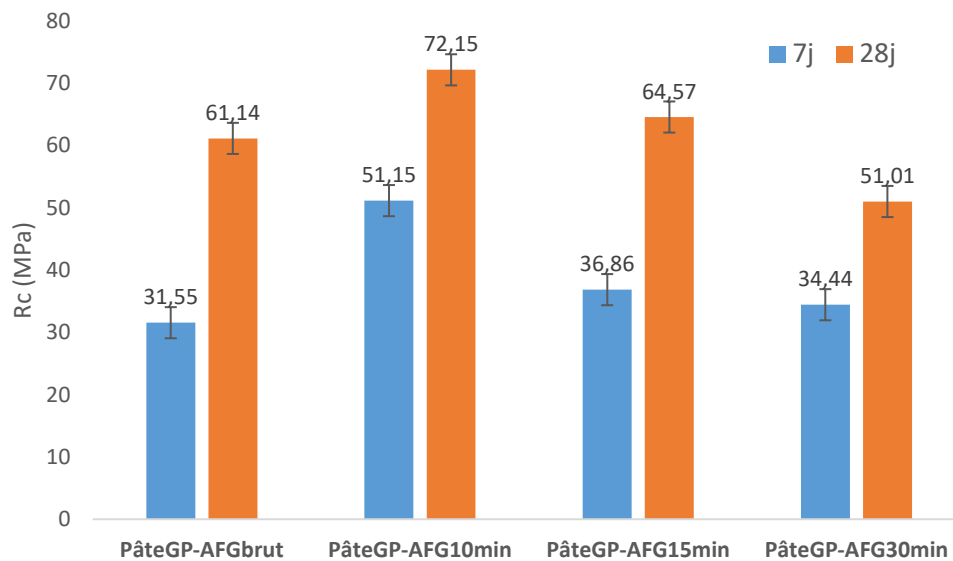
Figure IV-20 : Résistances à la compression des pâtes géopolymères produites par mécanosynthèse indirecte à 7 et 28 jours de séchage.
