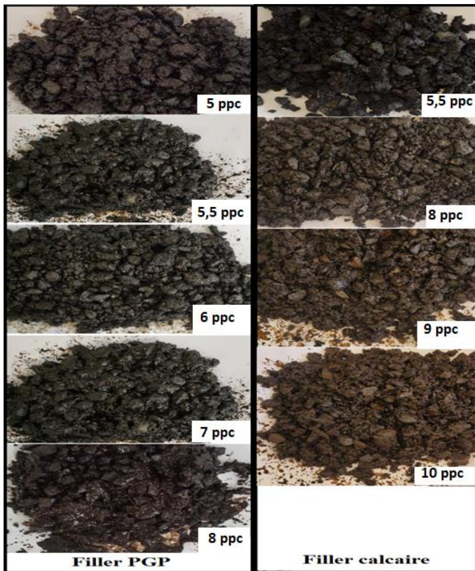
Figure V-7 : Formulations d'enrobés à l'émulsion avec différentes teneurs en eau totale.
