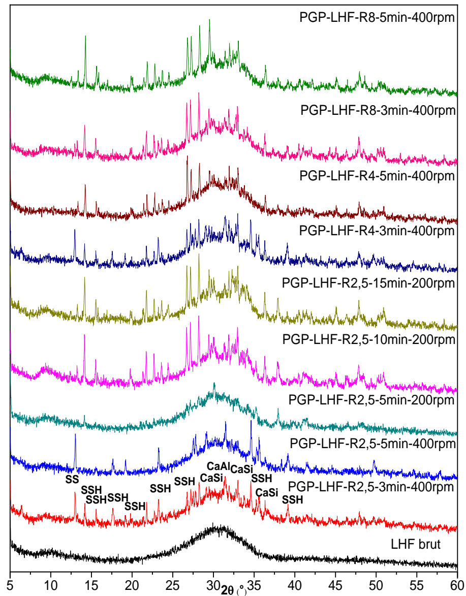
Figure III-4 : Diffractogrammes du LHF brut et des PGP à base du LHF SSH : Sodium Silicate Hydrate (PDF 00-022-0892), SS : Sodium Silicate (PDF 00-035-0344), CaSi : Calcium Silicate (PDF 00-017-0449), CaAl : Calcium aluminide (PDF 01-078-3541).
