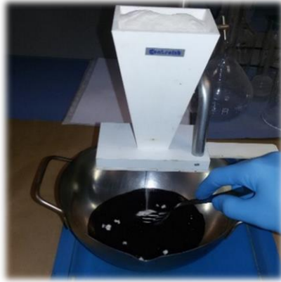
Figure II-17 : Dispositif utilisé pour la détermination de l'IREC.
