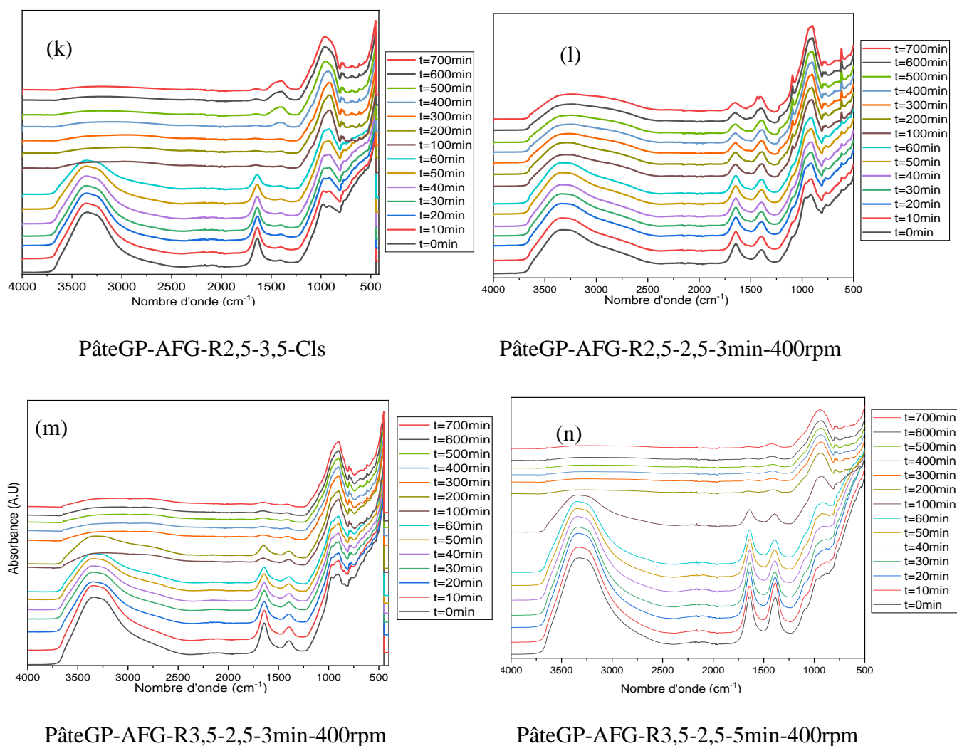
Figure IV-5 : Spectres de suivi infrarouge des pâtes géopolymères à base de CV (a-c), LHF (d-g), MK (h-j) et AFG (k-n).
