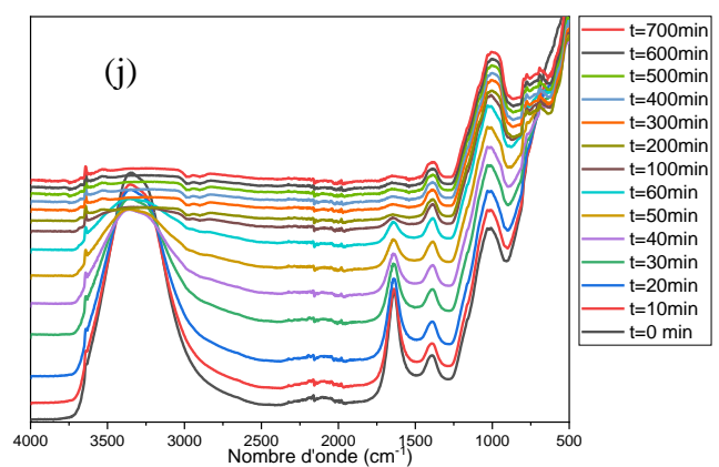
PâteGP-MK-CK1,5-3min-400rpm
