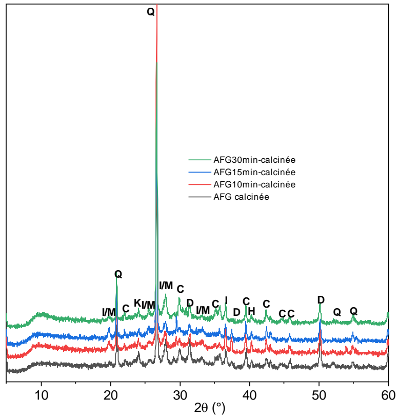
Figure III-10 : Diffractogrammes des poudres d'AFG brutes calcinées et activées par mécanosynthèse indirecte.
