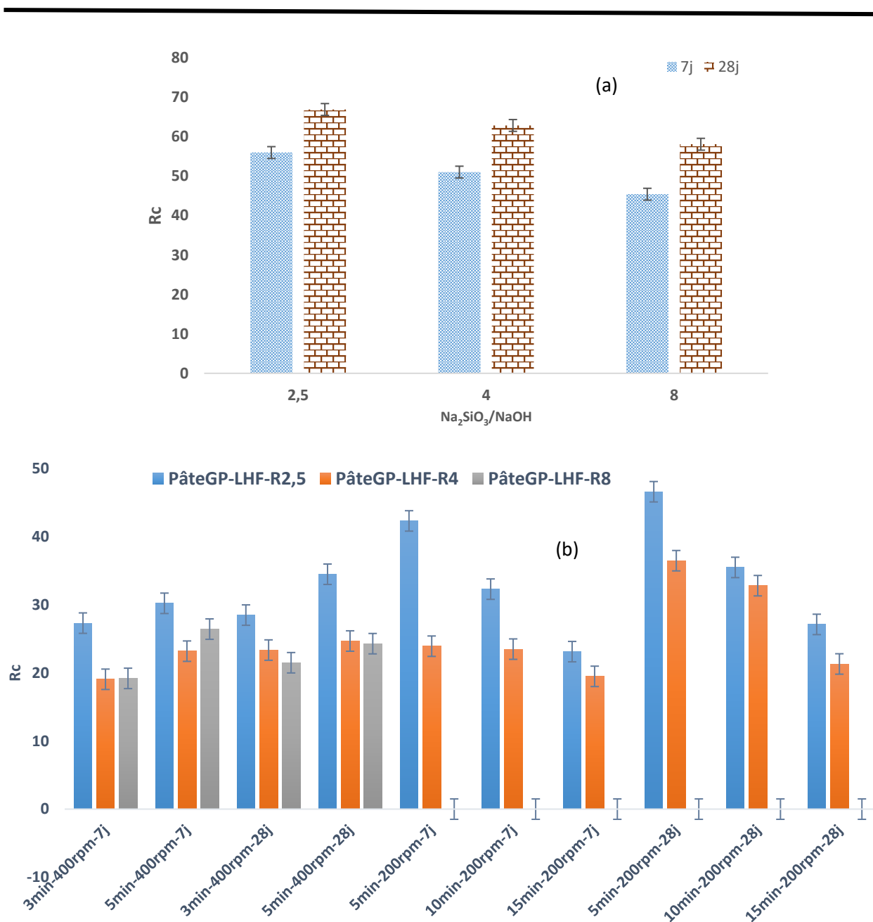
Figure IV-14 : Résistance à la compression des pâtes géopolymères à base de LHF obtenues par la méthode (a) classique et (b) par mécanosynthèse à 7 et 28 jours de séchage.
