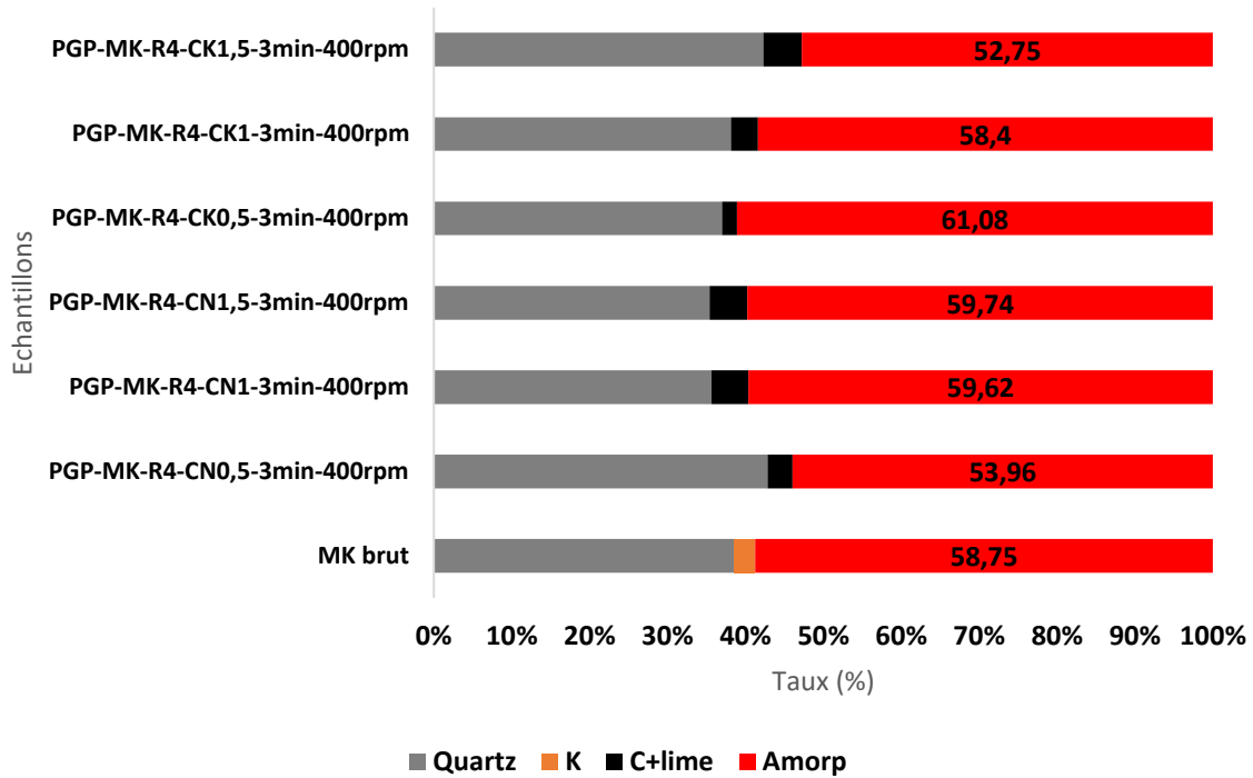
Figure III-6 : Quantification des phases cristallines et du taux d'amorphisation du MK et PGP à base de MK.
