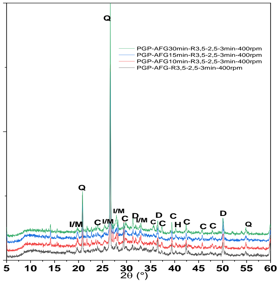
Figure III-12 : Diffractogrammes des poudres pré-géopolymères à base d'AFG produites par mécanosynthèse indirecte.
