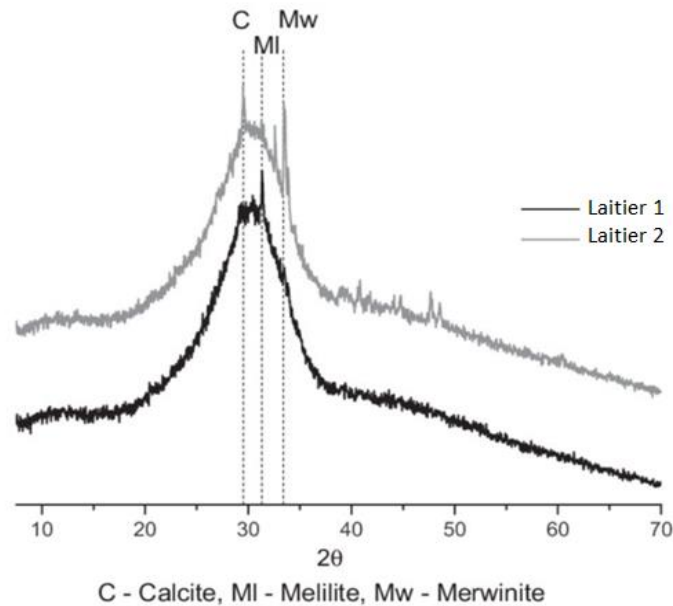
Figure I-9 : Exemple de diffractogrammes de deux laitiers de haut fourneau [52].
