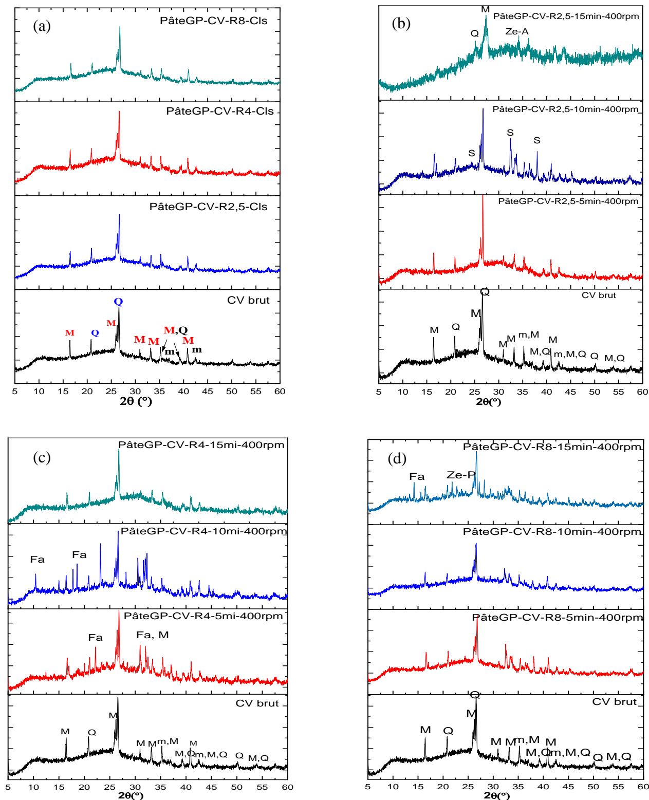
Figure IV-1 : Diffractogrammes des pâtes géopolymères à base de CV classique (a) et mécanosynthèse pour les rapports \text{Na}_2\text{SiO}_3/\text{NaOH} de 2,5 (b), 4(c) et 8(d). Fa : Faujasite-Na-Syn PDF 00-039-1380, S : Sodalite (PDF 00-024-1045), Q : Quartz (PDF 00-005-0490), m: magnétite (00-025-1376), M : Mullite (PDF 00-015-0776), Ze-P: Zéolite P (PDF 01-089-6322).
