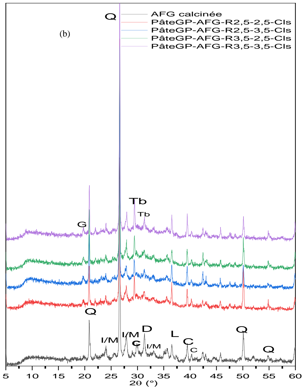
Figure IV-4 : Diffractogrammes des pâtes géopolymères à base d'AFG de poudres obtenues par mécanosynthèse (a) et classique (b). I/M : Illite/Muscovite (PDF 01-078-5136) / (PDF 00-074-4856), D : Dolomite (PDF 00-036-0426), K : Kaolinite (PDF 01-078-2110), C : Calcite (PDF 00-003-0526), L : Lime (PDF 00-002-1088), C-S-H : Calcium silicate hydrate (PDF 00-003-0548), Tb : Tobermorite (PDF 00-011-073), G : Gehlénite (PDF 00-019-0210), C-A-S-H : Calcium Aluminum Silicate hydrate (PDF 00-015-0171).
