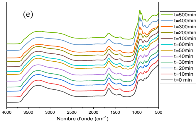
PâteGP-LHF-R2,5-5min-400rpm
