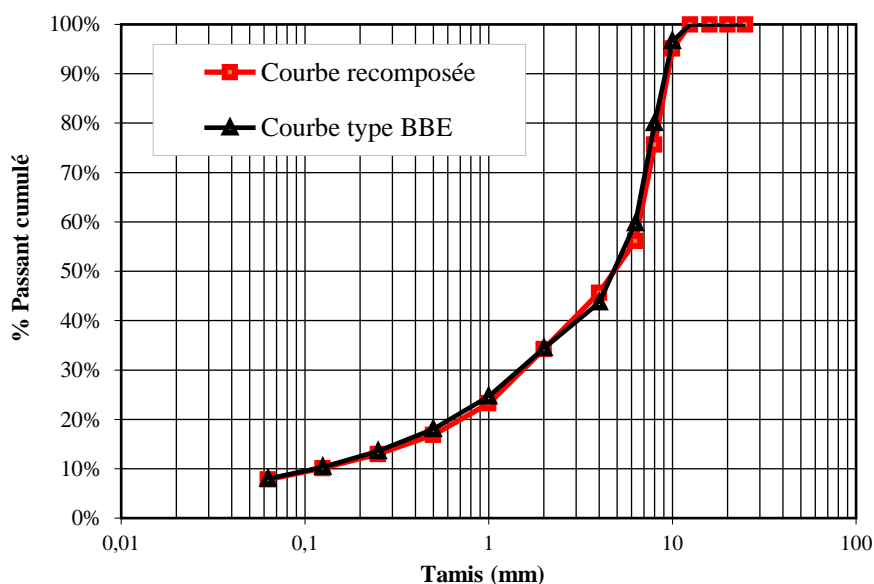
Figure II-19 : Recomposition granulométrique pour la formule de l'enrobé bitumineux.
