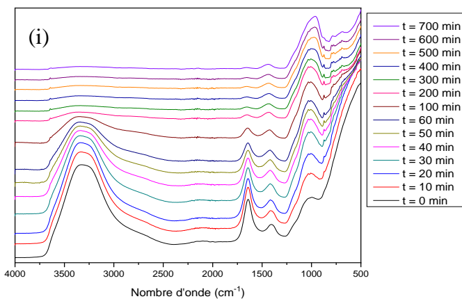
PâteGP-MK-CN1-3min-400rpm
