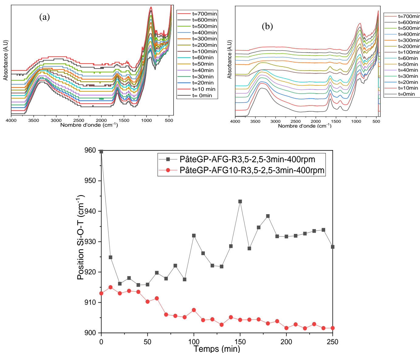
Figure IV-18 : Spectres des suivis infrarouges et suivi de la position Si-O-T en fonction du temps des échantillons (a) PâteGP-AFG10min-R3,5-2,5-3mi-400rpm et (b) PâteGP-AFG-R3,5-2,5-3min-400rpm.
