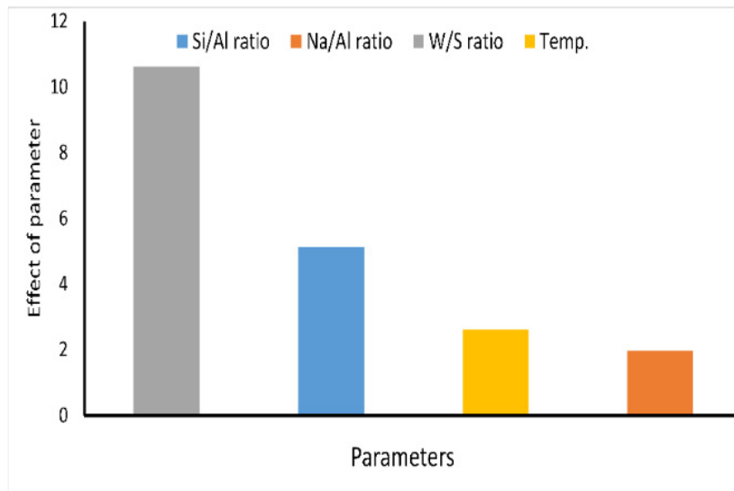
Figure I-16 : Effet de différents facteurs sur le temps de prise des matériaux géopolymères, d'après Siyal et al. [73].
