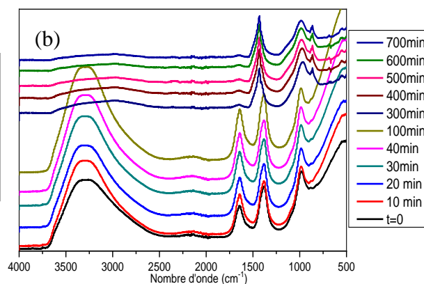
PâteGP-CV-R2,5-5min-400rpm
