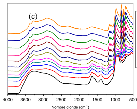
PâteGP-CV-R8-15min-400rpm
