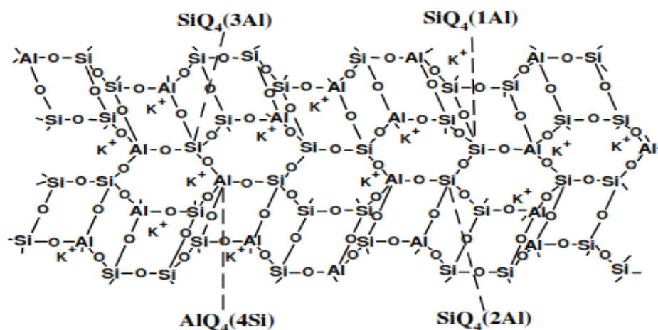
Figure I-14 : Structure proposée par Davidovits pour le géopolymère K-Poly(sialate-siloxo) [6].
