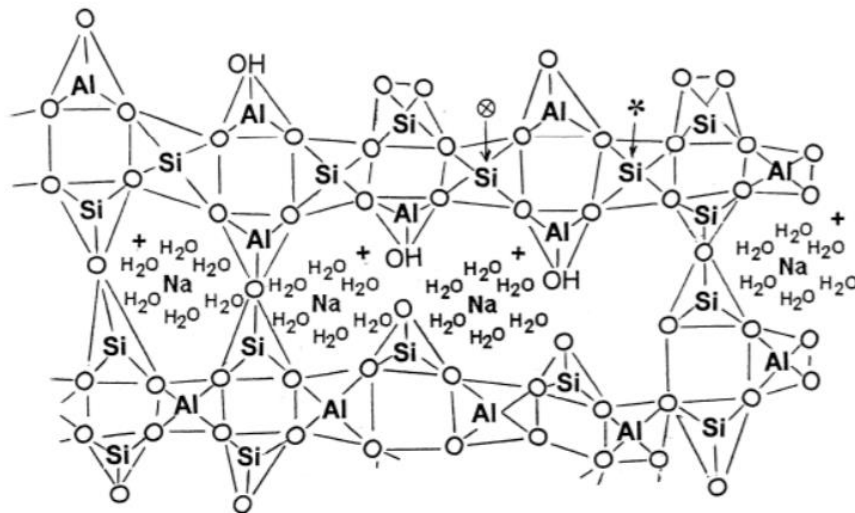
Figure I-15 : Modèle de structure d'un géopolymère Na-polysialate proposé par Barbosa et al. [93].
