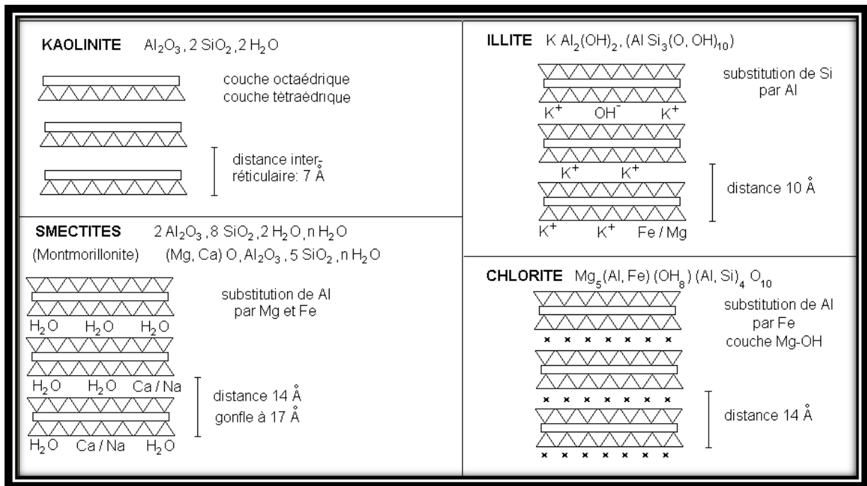
Figure I-11 : Structures des argiles phylliteuses [58].
