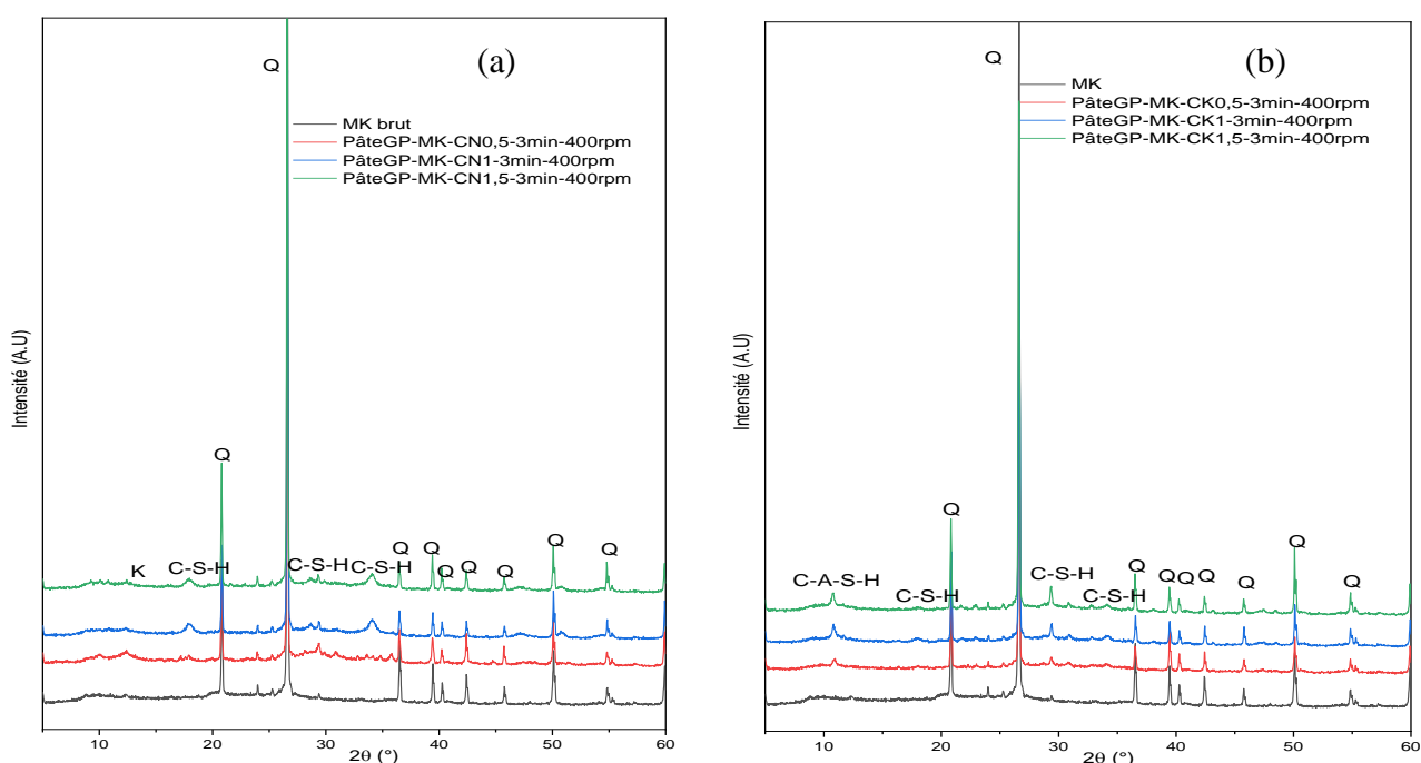
Figure IV-3 : Diffractogrammes des pâtes géopolymères à base de MK activé par CaO et NaOH (a) et KOH (b). K : Kaolinite (PDF 01-078-2110), Q : Quartz (PDF 00-005-0490), C-S-H : Calcium silicate hydrate (PDF 00-003-0548), C-A-S-H : Calcium Aluminum Silicate Hydrate (PDF 00-015-0171).
