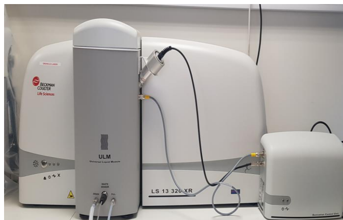
Figure II-8 : Granulomètre laser.
