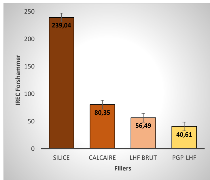
Figure V-4 : IREC « modifié » pour le filler calcaire, le LHF brut et la PGP-LHF.
