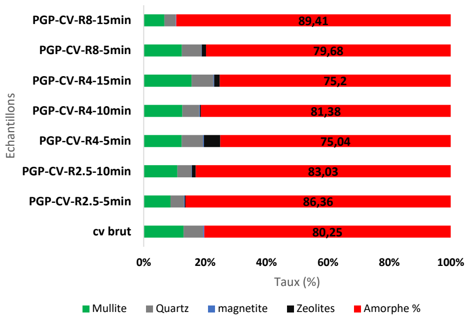
Figure III-3 : Quantification des phases cristallines et du taux d'amorphisation des CV et PGP à base de CV.
