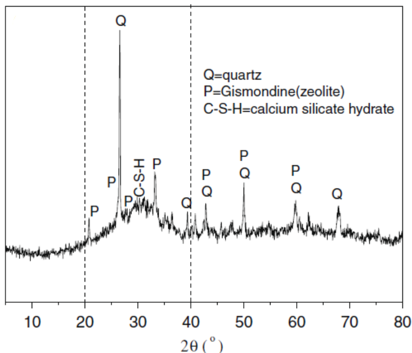
Figure I-13 : Diffractogramme d'un matériau géopolymère étudié par Guo et al. [88].
