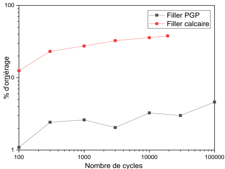
Figure V-11 : Résultats d'orniérage des enrobés à l'émulsion.
