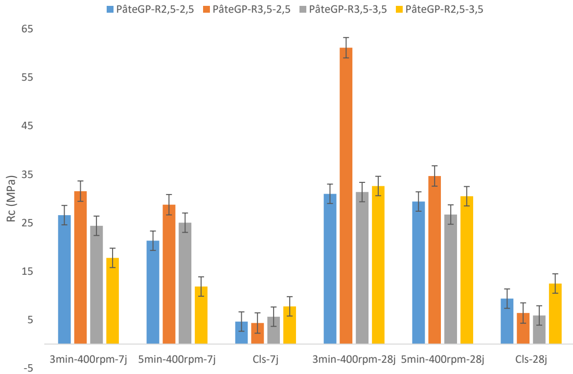
Figure IV-16 : Résistance à la compression des pâtes géopolymères à base d'AFG à 7 et 28 jours de séchage.
