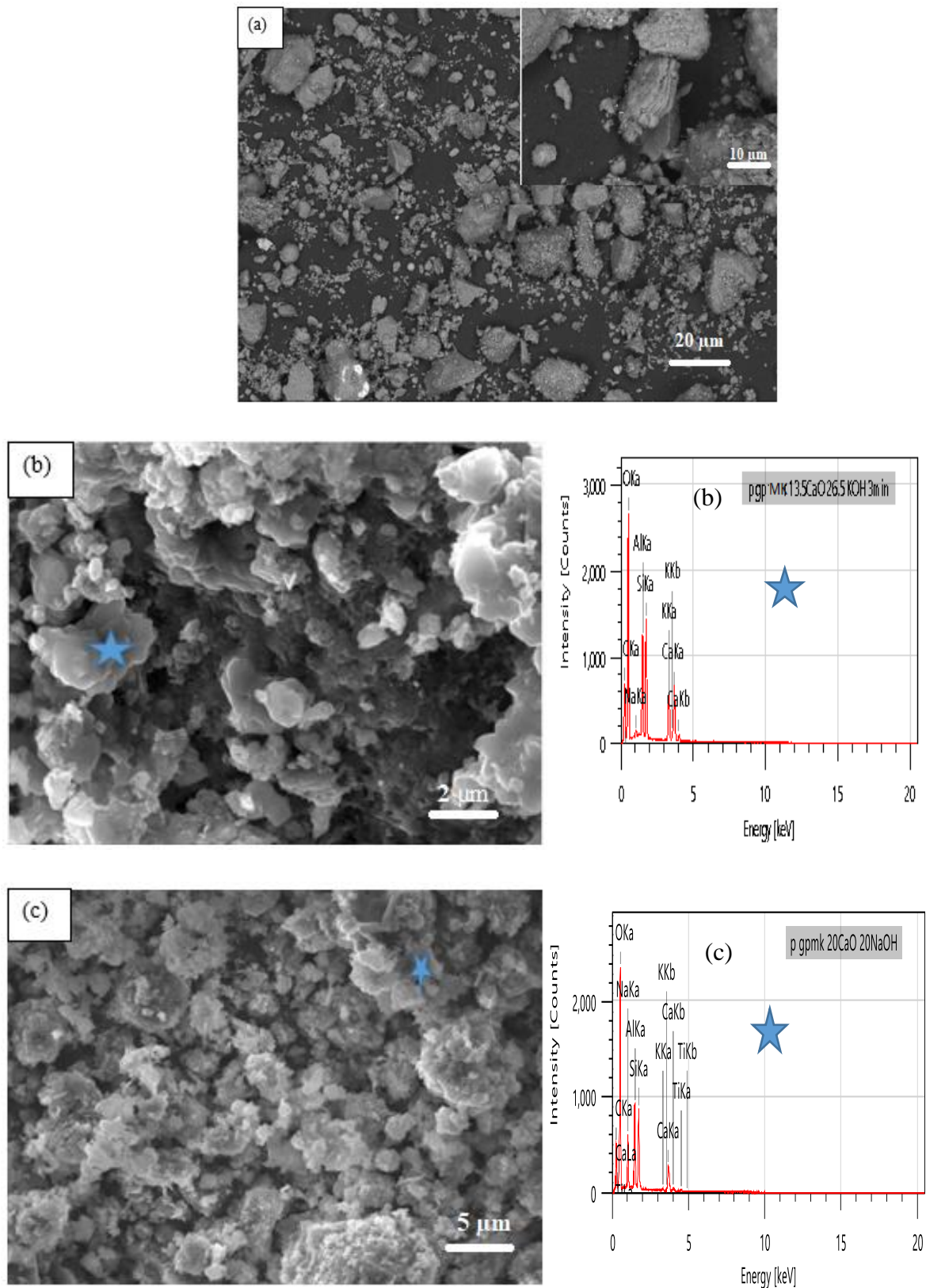
Figure IV-11 : Micrographies avec analyse EDX des échantillons (a) MK brut, (b) PâteGPGP-MK-CK0,5-3min-400rpm et (c) PâteGPGP-MK-CN1-3min-400rpm.
