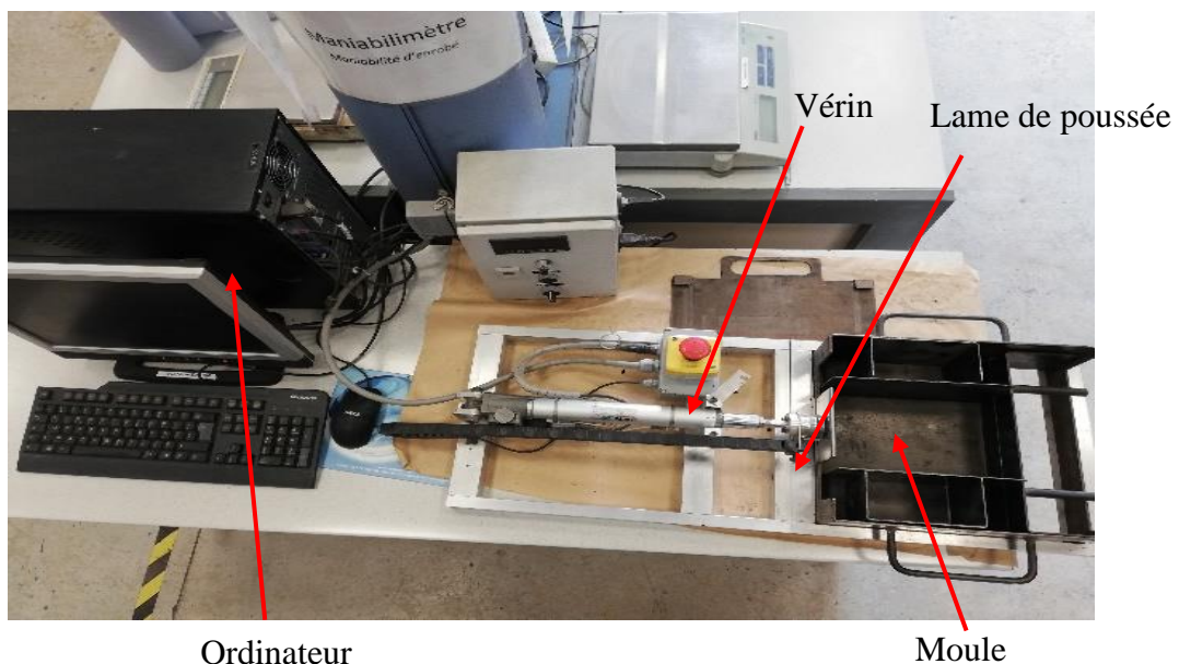
Figure II-22 : Maniabilimètre utilisé à l'IRC-ESTP Paris.
