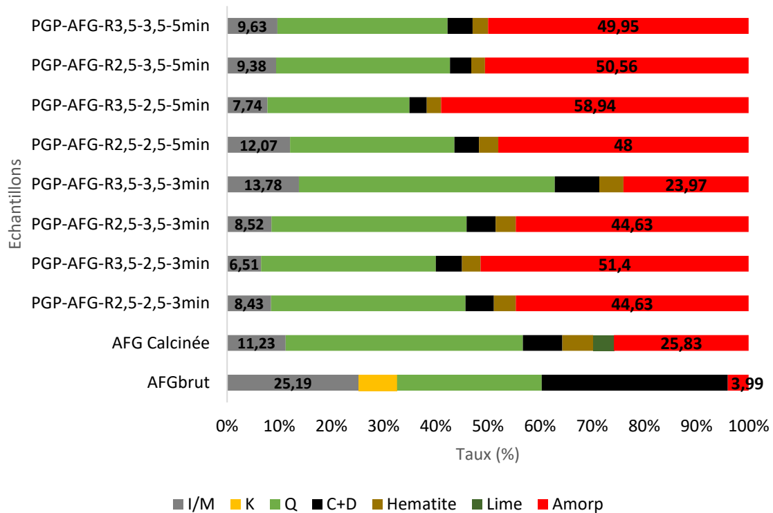
Figure III-8 : Quantification des phases cristallines et du taux d'amorphisation par la méthode Rietveld pour l'AFG brute et les PGP à base d'AFG (b).
