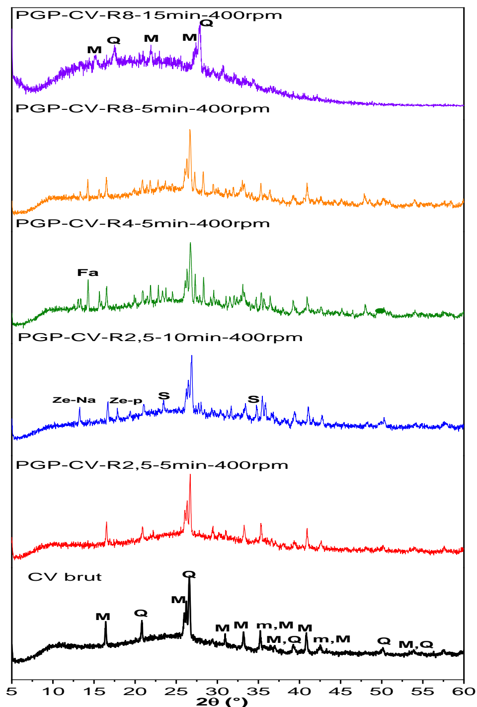
Figure III-2 : Diffractogrammes des PGP à base de CV.
