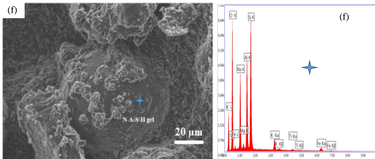
Figure IV-9 : Micrographies avec analyse EDX des échantillons (a) CV brutes, (b) PâteGPGP-CV-R2,5-5-Cl, (c) PâteGP-CV-R2,5-5min-400rpm, (d) PâteGP-CV-R2,5-10min-400rpm, (e) PâteGP-CV-R4-10min-400rpm ET (f) PâteGP-CV-R8-15min-400rpm.
