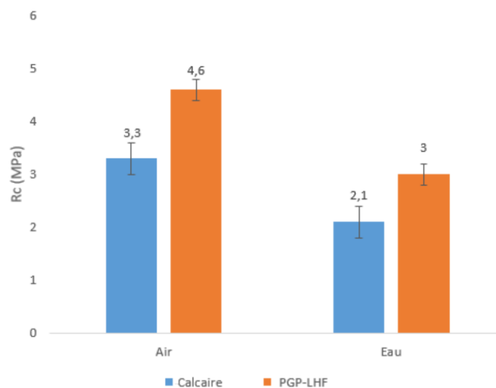
Figure V-9 : Résistance à la compression dans l'air et dans l'eau des enrobés de référence et géopolymère.
