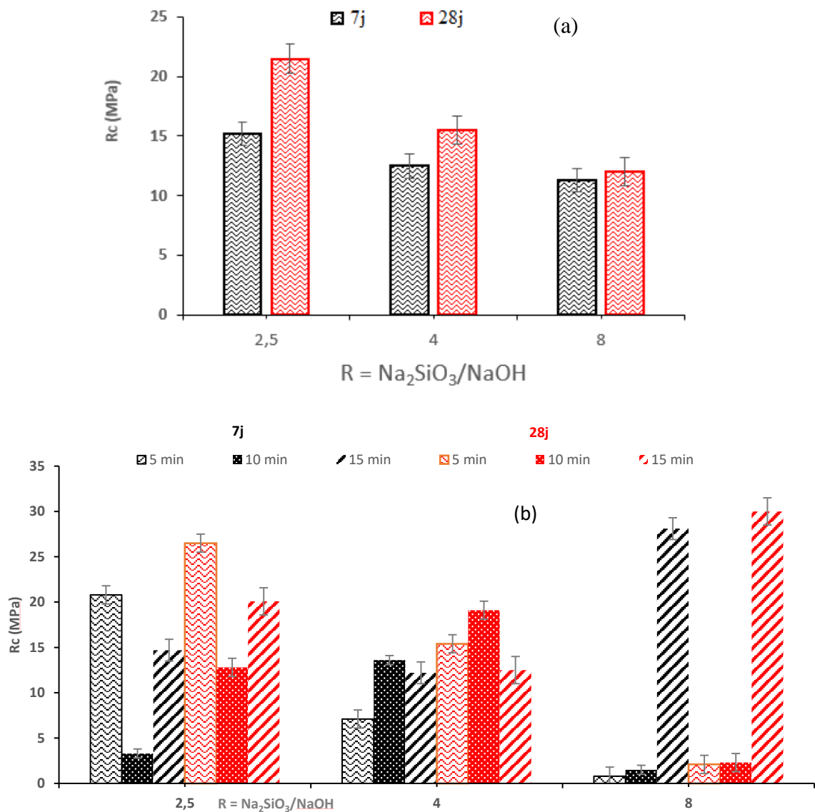
Figure IV-13 : Résistance à la compression des pâtes géopolymères à base de CV obtenues par la méthode (a) classique et (b) par mécanosynthèse à 7 et 28 jours de séchage.
