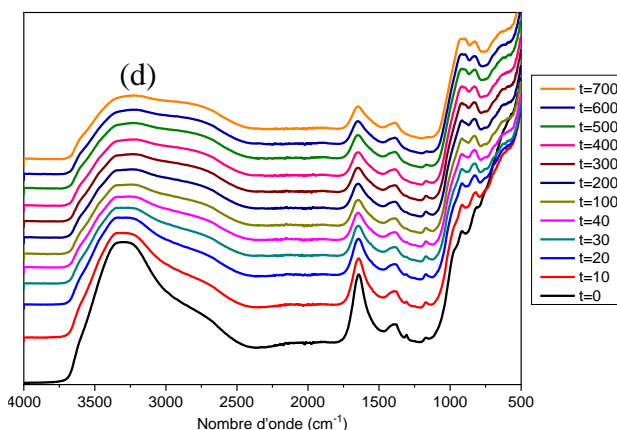
PâteGP-LHF-R2,5-3min-400rpm
