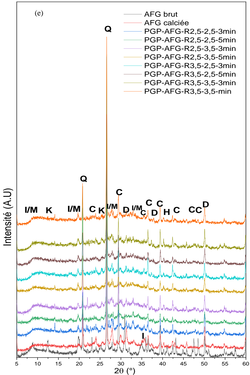
Figure III-7: Diffractogrammes de l'AFG et des poudres pré-géopolymères à base d'AFG (e). Q : Quartz (PDF 00-005-0490), C : Calcite (PDF 00-003-0526), I/M : Illite/Muscovite (PDF 01-078-5136) / (PDF 00-074-4856), D : Dolomite (PDF 00-036-0426), K : Kaolinite (PDF 01-078-2110), H Hématite.
