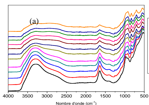
PâteGP-CV-R2,5-ClS
