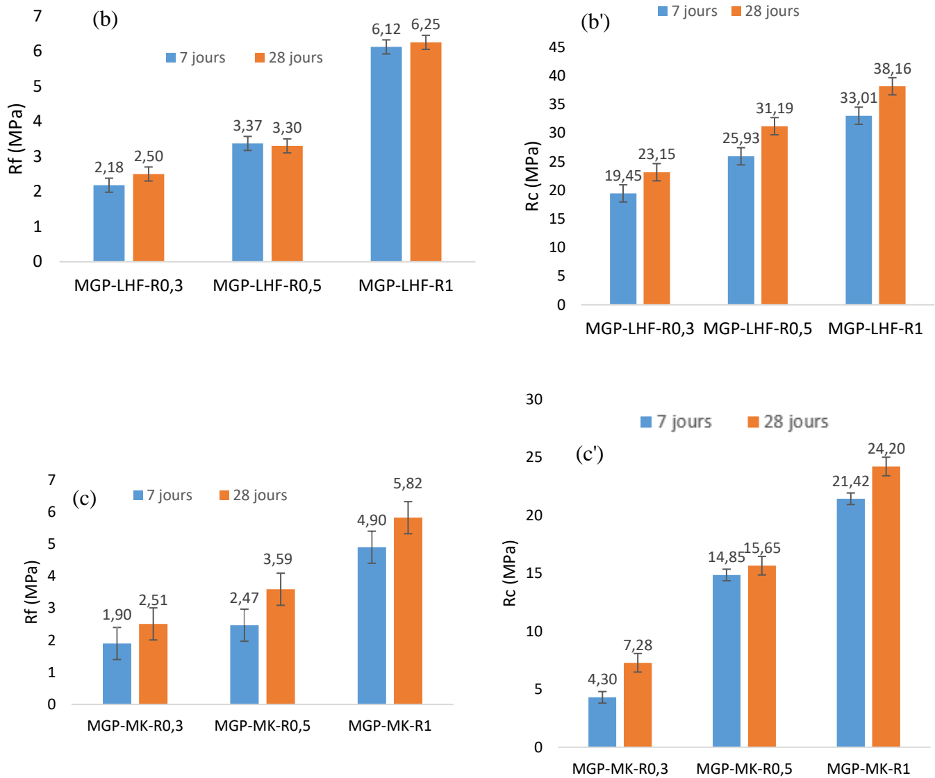
Figure V-3 : Résistances mécaniques des mortiers géopolymères à base de CV (a), LHF (b) et MK (c).
