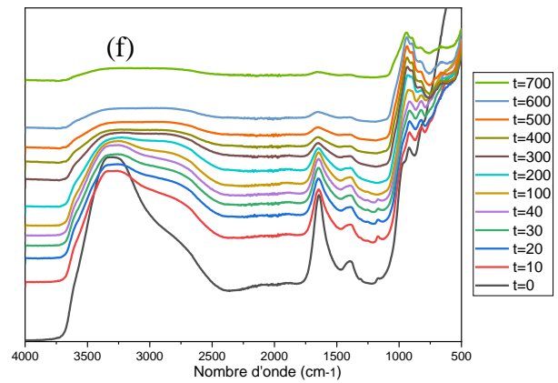
PâteGP-LHF-R2,5-5min-200rpm
