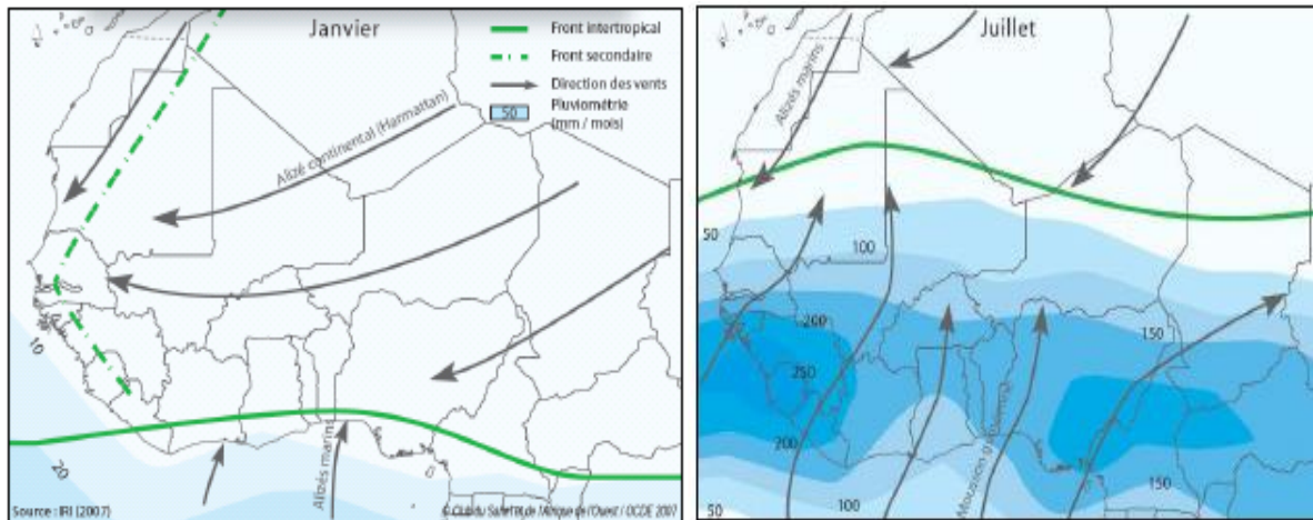
Figure 12 : Cycle de la mousson en Afrique de l'Ouest Source : Totin, 2010 et Akindélé, 2014
