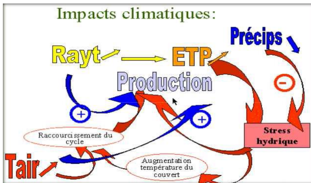
Figure 3 : Schéma synthétique des impacts climatiques sur la production agricole : augmentation de la température de l'air, du rayonnement solaire, diminution des précipitations et de l'ETP
