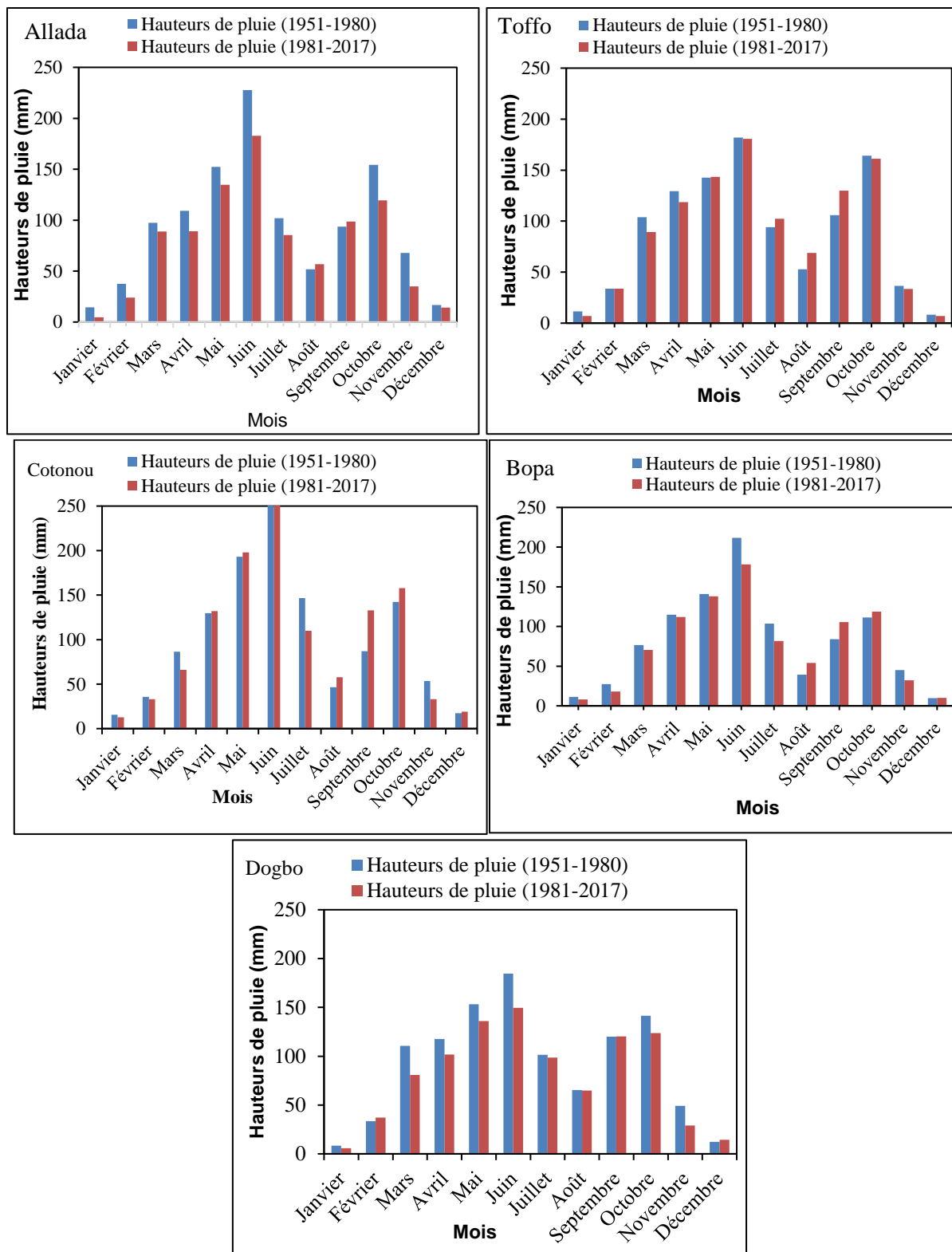
Figure 23 : Variation inter-mensuelle des précipitations entre 1951 et 1980 et entre 1981 et 2017
