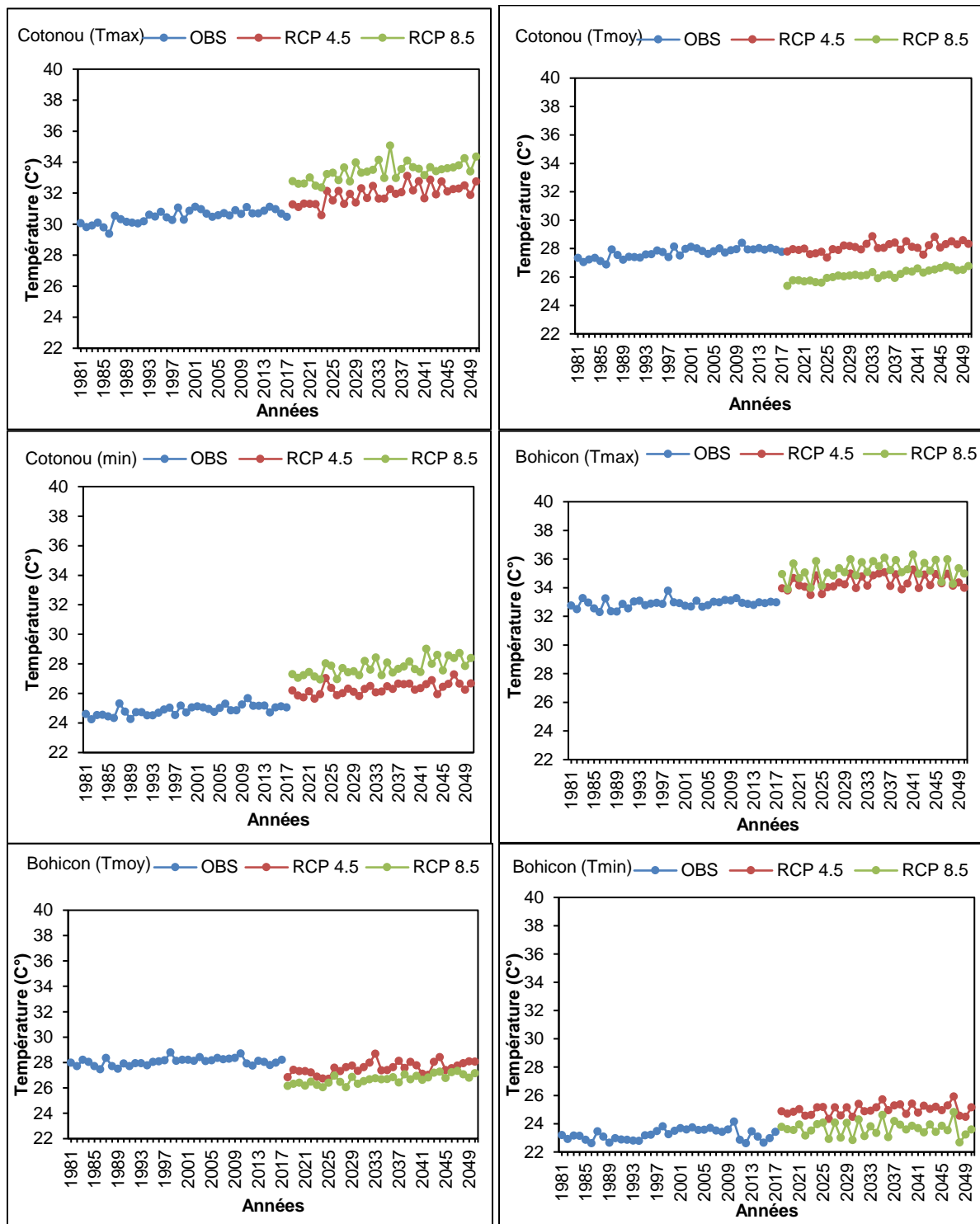
Figure 41 : Projection des températures annuelles dans la dépression médiane Source des données : Météo-Bénin, avril 2019
