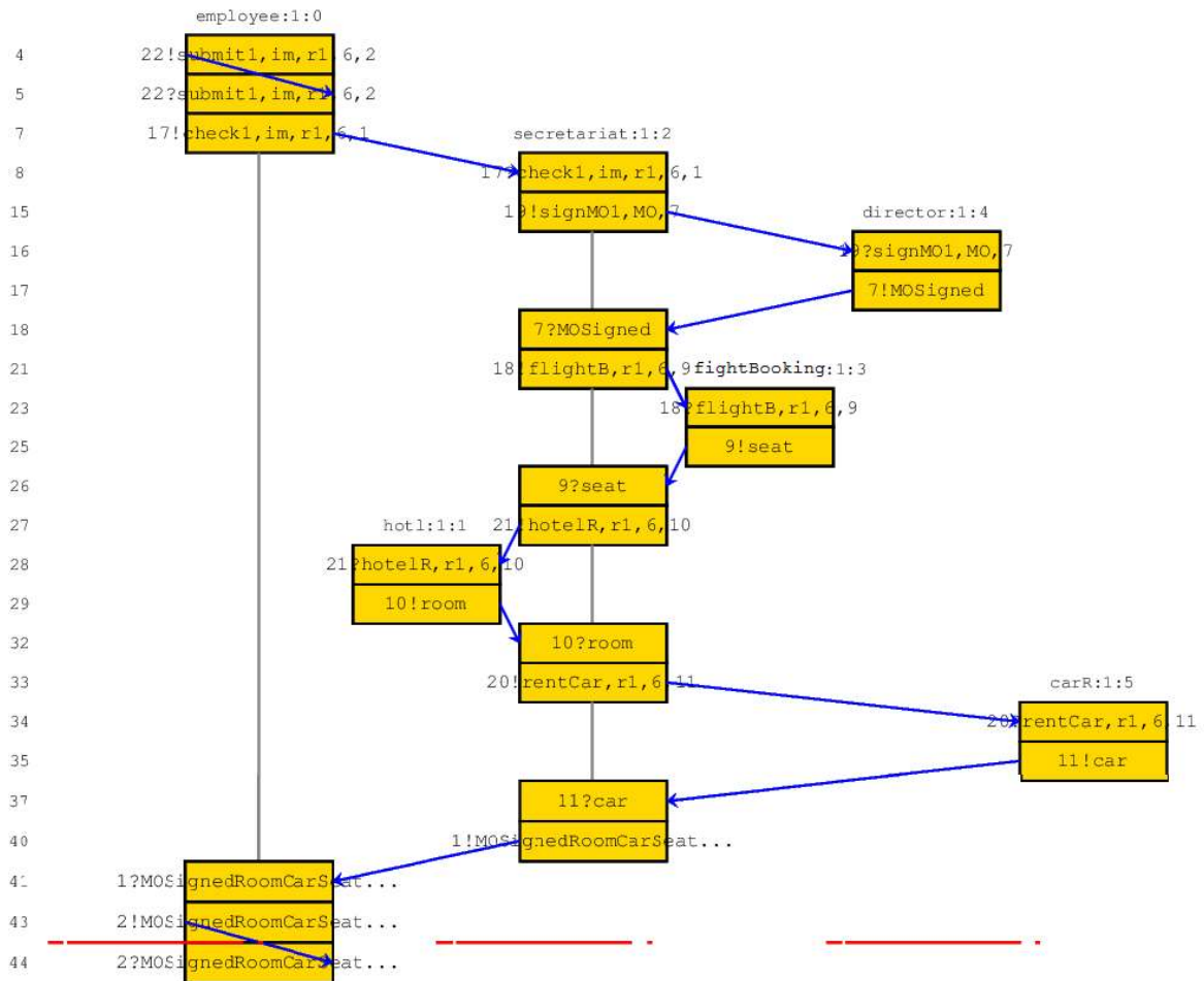
FIGURE 4.9: Une exécution possible
