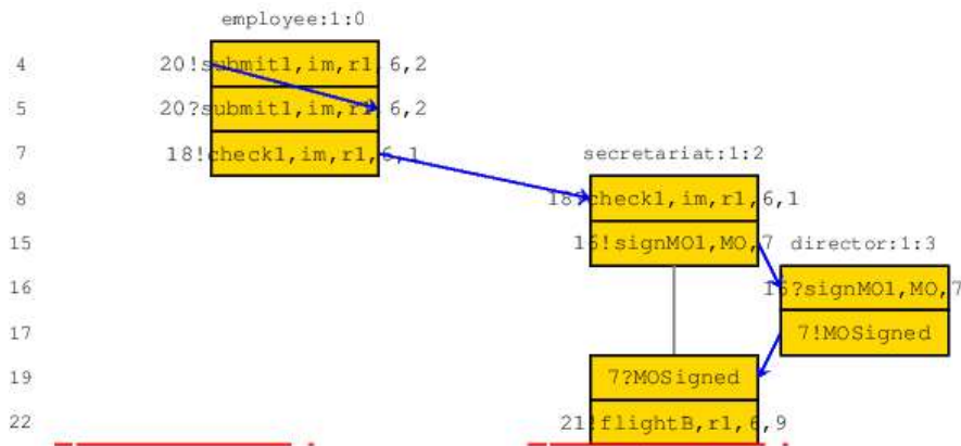
FIGURE 4.11: Le processus flightBooking n'est pas disponible
