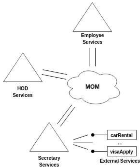
FIGURE 4.12: Le style architectural du moteur d'exécution
