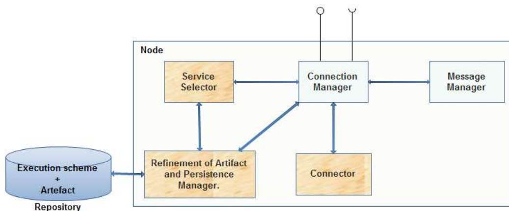
FIGURE 4.5: Les éléments du Backend
