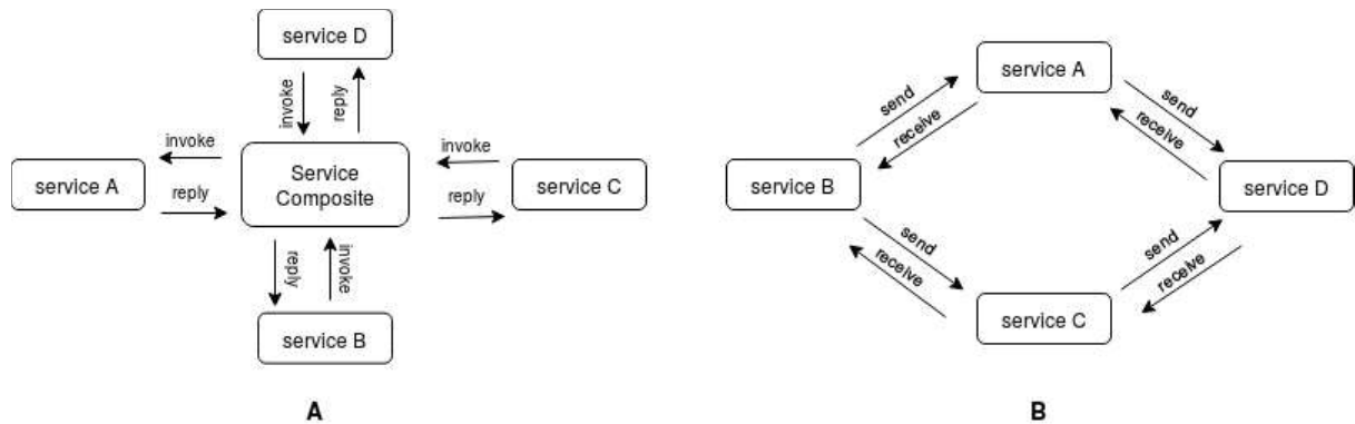
FIGURE 1.2: Orchestration vs Chorégraphie [19]
