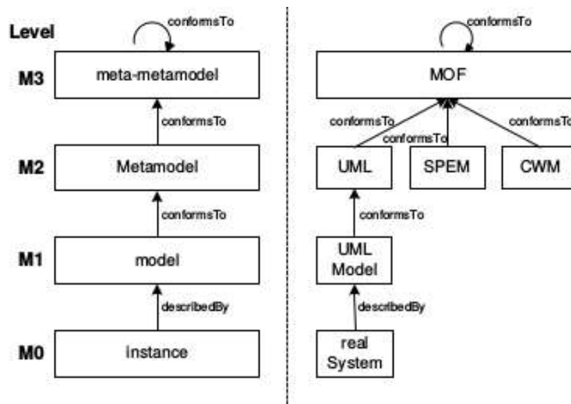
FIGURE 3.2: L'architecture de métamodélisation à quatre couches [74]
