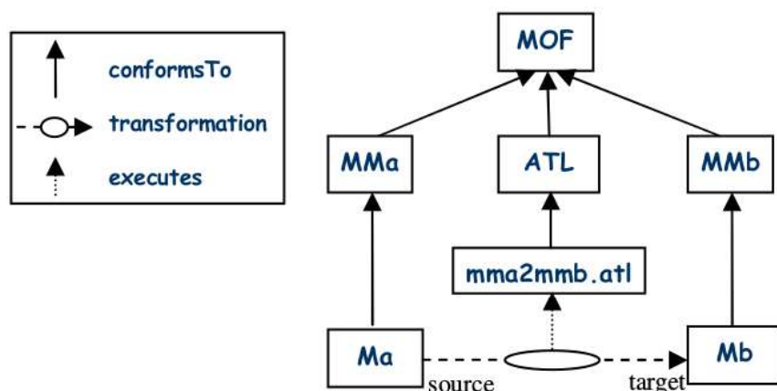
FIGURE 4.1: Aperçu de l'approche transformationnelle ATL [89]
