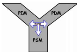
FIGURE 3.3: Étapes de l'approche MDA [75]
