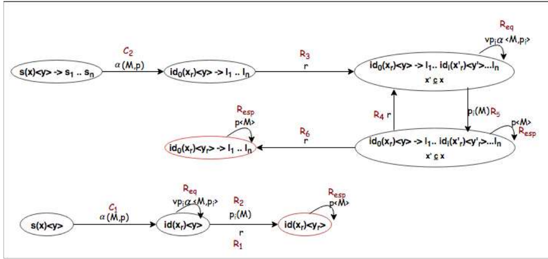
FIGURE 2.1: Progression d'un service instancié
