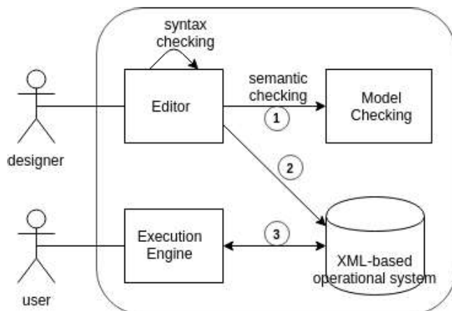
FIGURE 4.3: Framework de vérification et de validation
