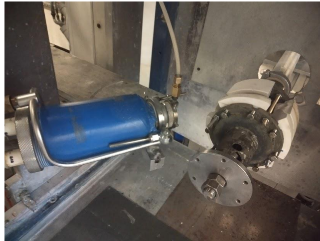
Figure II-31. Essai préliminaire de scellement par projection thermique de pièces cylindriques.
