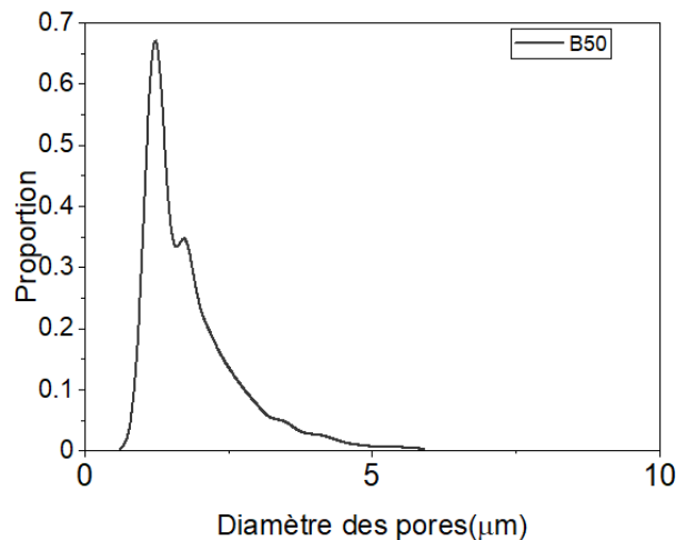
Figure III-5. Distribution en taille des pores de la céramique B50.
