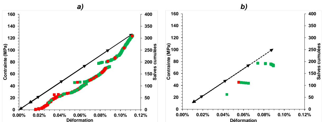
Figure IV-11. Contrainde et salves cumulés en fonction de la déformation pour le fritté B50 pendant les cycles de chargement a) et déchargement b) lors du test de flexion 4 points. Les salves cumulés sont classés en fonction de la gamme de fréquence (MF rouge, HF vert).
