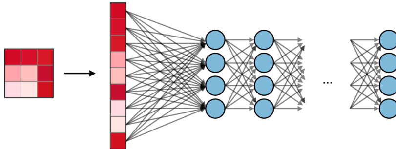
FIGURE 3.8 – Couche totalement connectée (FC), où chaque neurone d'une couche est connecté à tous les neurones de la couche suivante. Source : CS230 , avec l'autorisation de Afshine Amidi et Shervine Amidi, 2018
