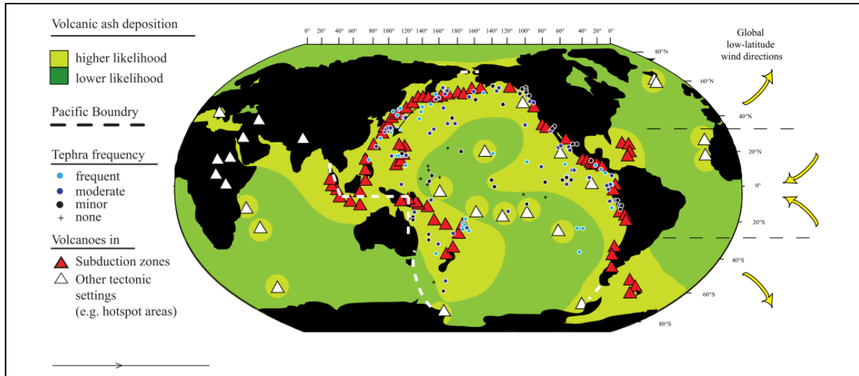
Figure I-4: Probabilité de dépôt de cendres volcaniques au-dessus de l’océan, avec distinction entre forte (vert clair) et faible (vert foncé) probabilité. Ces zones ont été estimées en fonction de la localisation de volcans historiquement actifs, de la direction du vent et de la proportion de téphra dans des sédiments marins du Quaternaire. Figure issue de Olgun et al. (2011) et basée sur les travaux de Straub and Schmincke (1998).
