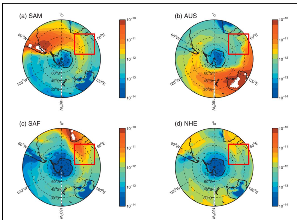
Figure I-5: Dépôt moyen annuel de poussières (kg.m -2 .s -1 ) sur l'Océan Austral et en Antarctique venant de quatre sources individuelles : (a) Amérique du Sud (SAM) ; (b) Australie (AUS) ; (c) Afrique du Sud (SAF) et (d) l'hémisphère Nord (NHE). Les points blancs symbolisent les régions sources de l'hémisphère Sud et les carrés rouges localisent la zone d'étude de la partie B de ce manuscrit. Figure modifiée depuis Li et al. (2008).
