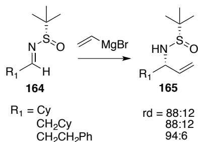
Schéma 47 : Premières additions décrites par Ellman
