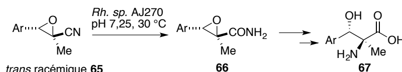
Schéma 19 : Formation d'acides aminés par biotransformation d'un nitrile
