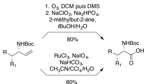
Schéma 125 : Synthèse d'acides \alpha -aminés \beta -substitués
