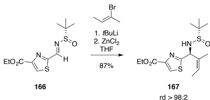
Schéma 48 : Addition de vinylzinc sur une hétéroarylimine
