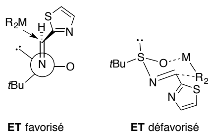
Figure 15 : Etat de transition pouvant justifier la sélectivité
