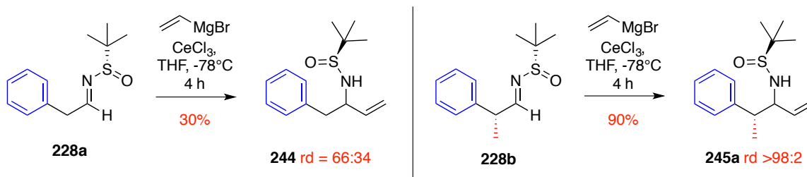
Schéma 93 : Addition de bromure de vinylmagnésium en présence de \text{CeCl}_3
