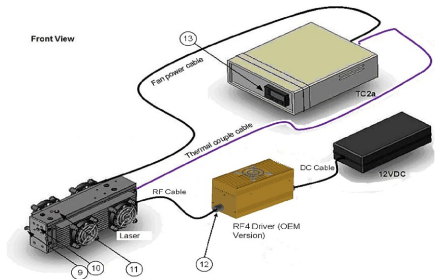
Figure 4.10 : Schéma de la connexion du système laser.
