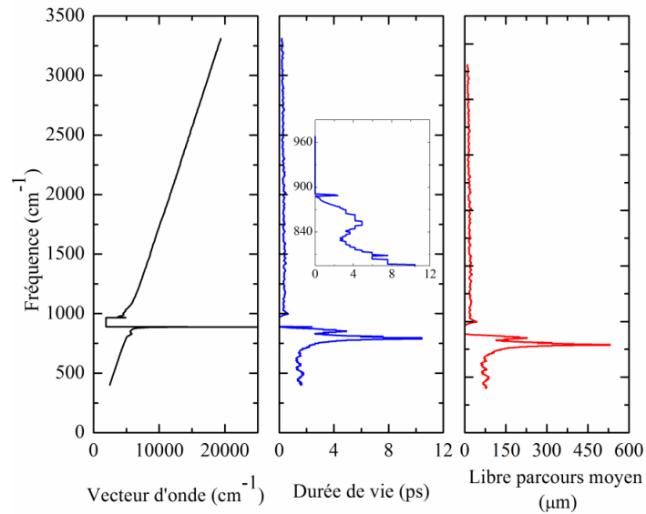
Figure 1.11 : La dispersion, la durée de vie, et le libre parcours moyen des phonons-polaritons de surface en fonction de l'énergie de ces modes.
