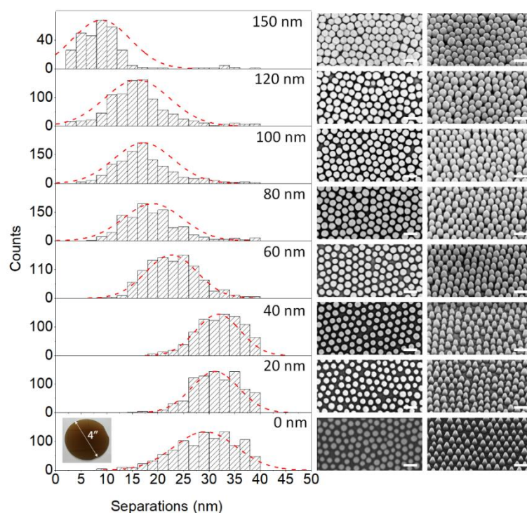
Illustration A.21. Histogrammes des distances entre les piliers en fonction de l'épaisseur des films d'or pulvérisés, et les images SEM des réseaux de nanopiliers acquis, vue de haut et inclinée (inclinaison de 30^\circ ). Les barres de mesure indiquent 200 nm. L'image des réseaux de nanopiliers uniformes de 4" sur des plaquettes de 4"Si est présentée dans l'encadré.
