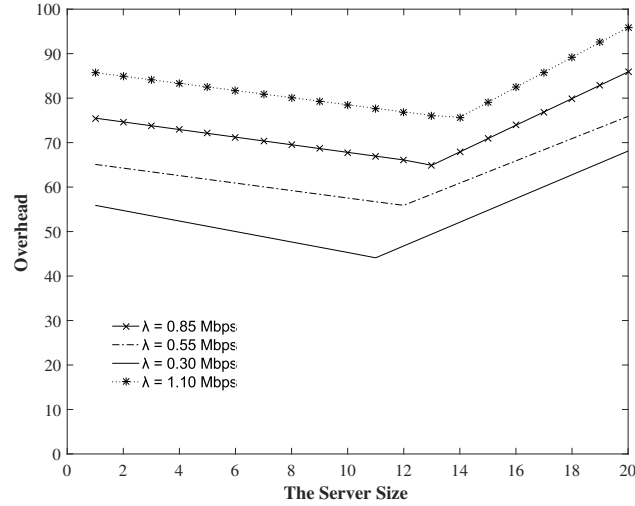
FIGURE 5.4 – La surcharge d'un nœud fog versus n et \lambda
