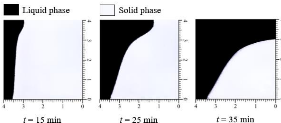
Fig. 6.7. Évolution de l'interface de fusion de la paraffine pure en fonction du temps
