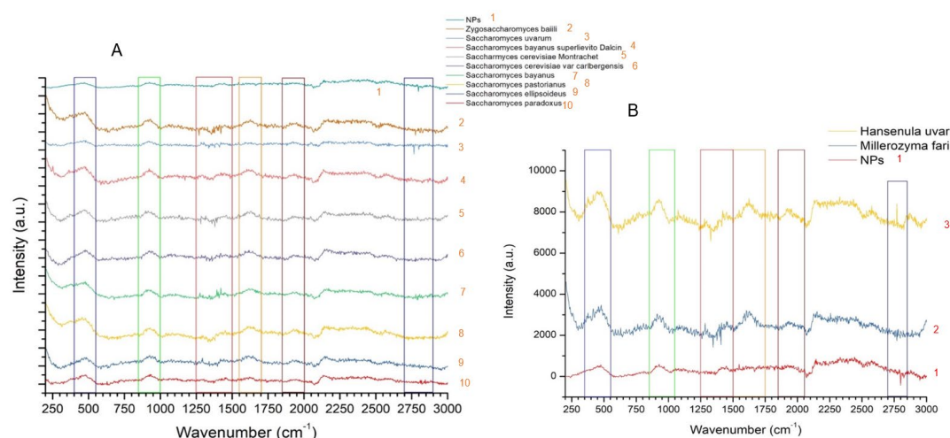
Figure 6. 8 Spectres SERS de différents microorganismes de Saccharomycetales (A), et Debaryomycetaceae ( Millerozyma farinosa ) et Saccharomycodaceae ( Hansenula uvarum ) (B), en utilisant un temps d'acquisition de 10 sec x 3 fois avec le filtre D0.
