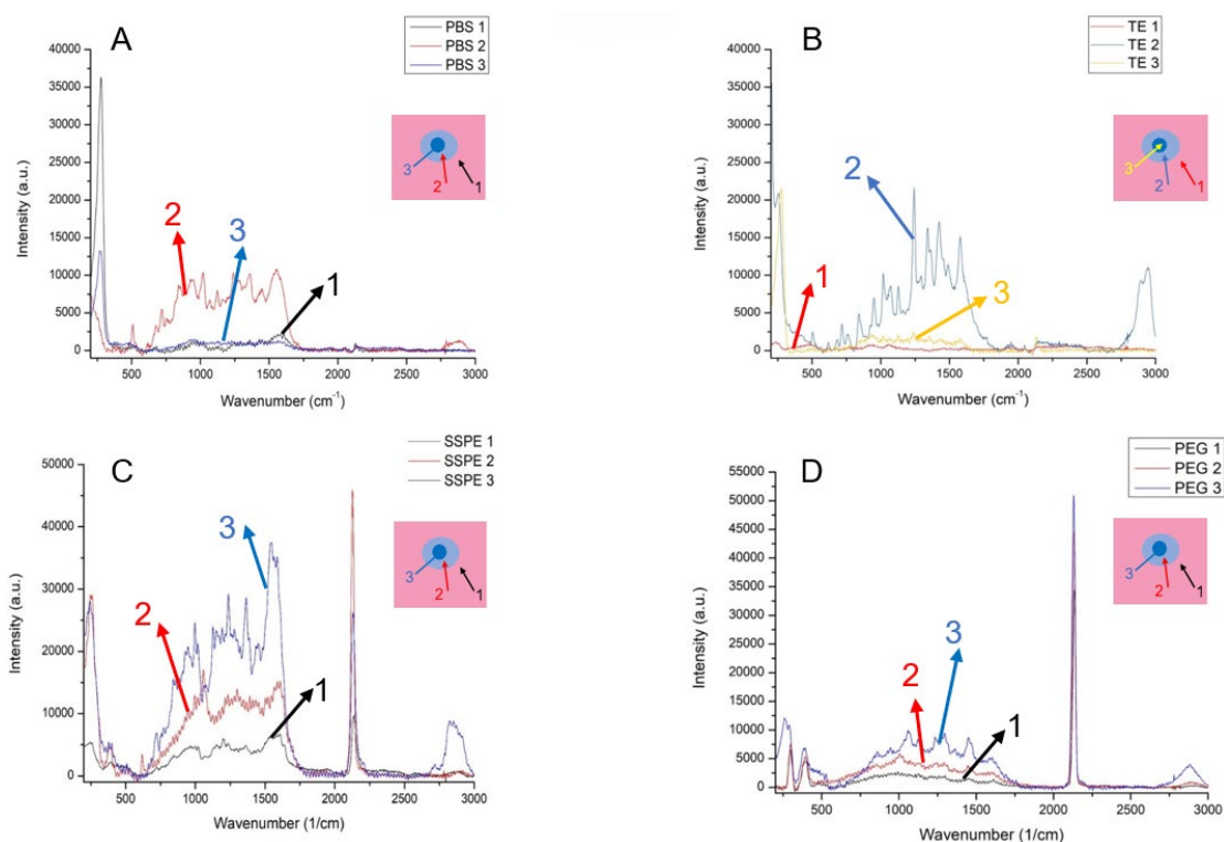
Figure 6. 7 Spectres SERS de 2 \mu\text{L} de gouttes de tampon PBS (A), de tampon TE (B), de 1 x SSPE (C), de tampon PEG (D) sur la surface active. Le temps d'acquisition était de 10 sec x 3 fois avec le filtre D0.3.
