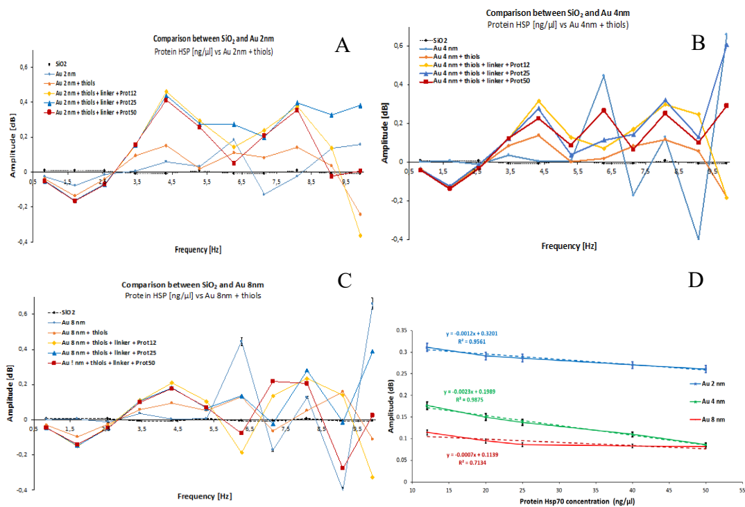
Figure 6.3 Caractérisation spectrale de matériaux ayant une épaisseur de film d'or de A) 2 nm, B) 4 nm et C) 8 nm pour différentes concentrations de protéines Hsp70 (12, 25 et 50 ng/μL/cm 2 ) ; D) Courbes d'étalonnage du Hsp70 déposé sur des nanostructures d'or (2nm, 4nm et 8 nm, respectivement) à 4,33 GHz.
