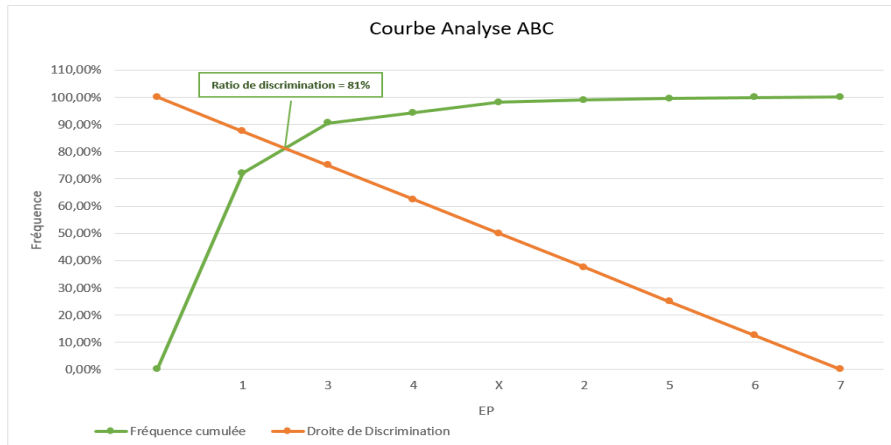
FIGURE 3.2 – Courbe d’analyse ABC pour les catégorise EP à simuler
