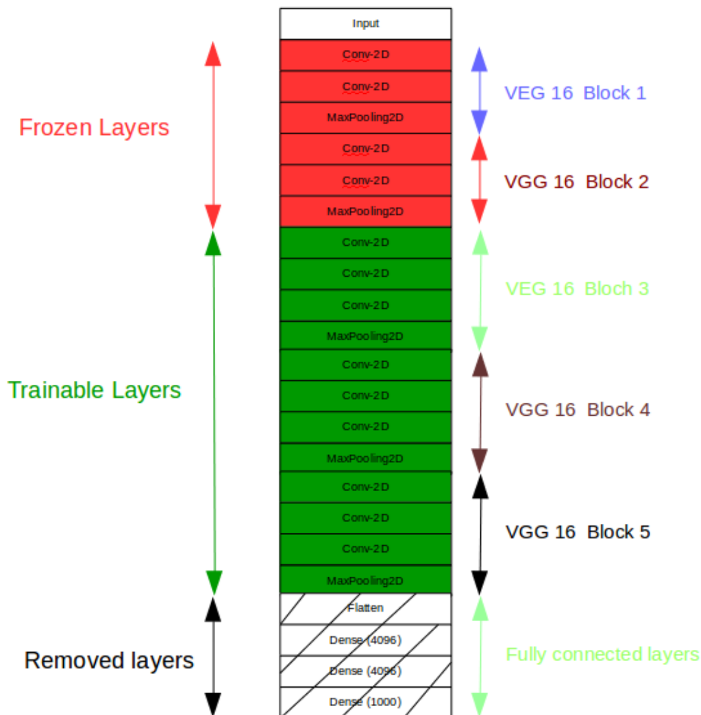
FIGURE 6.3: Architecture VGG 16 utilisée pour le réglage fin de l'objectif d'une classe unique
