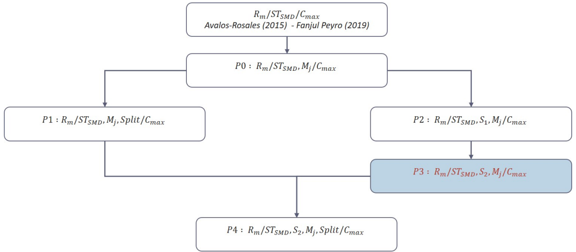
FIGURE 4.8 – Construction du modèles mathématique qui correspond au problème Petit Bateau
