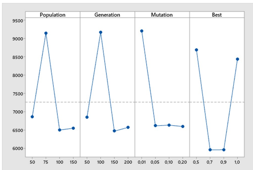
FIGURE 4.22 – Méthode Taguchi - résultats des paramètres
