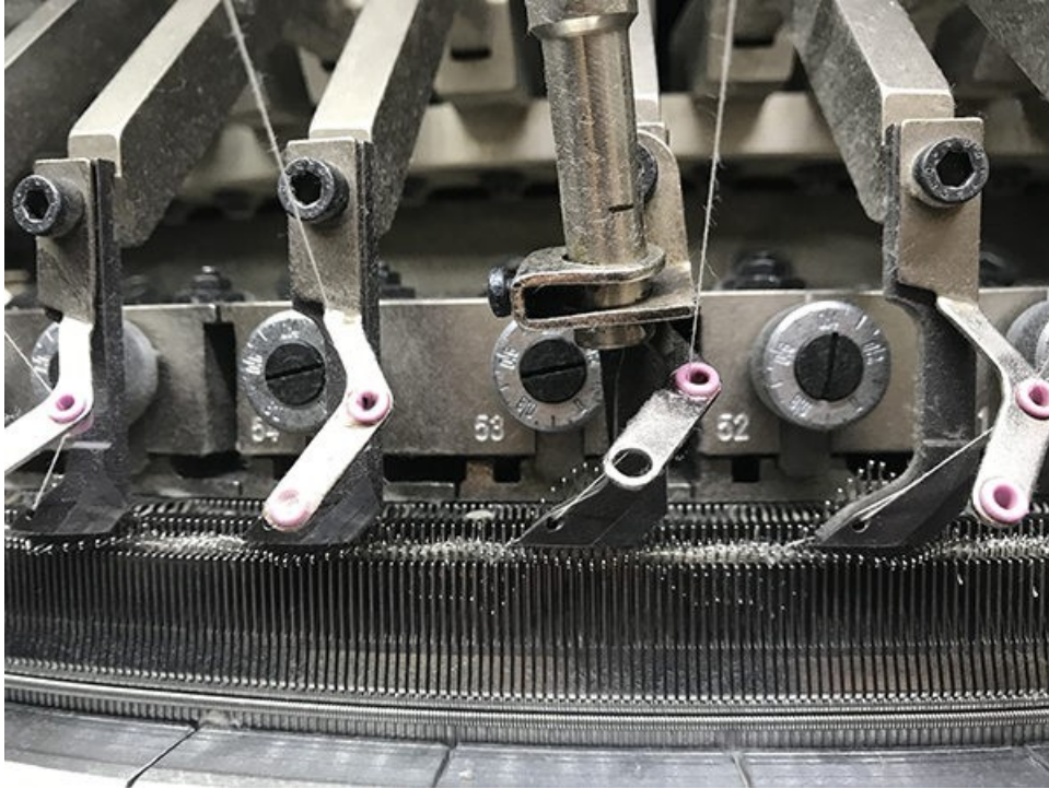
FIGURE 3.2 – Les machines rotatives tricotent grâce à leurs quelques 3 000 aiguilles
