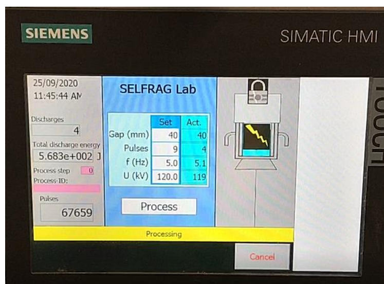
Figure 3-33 : Ecran de contrôle du dispositif SELFRAG Lab
