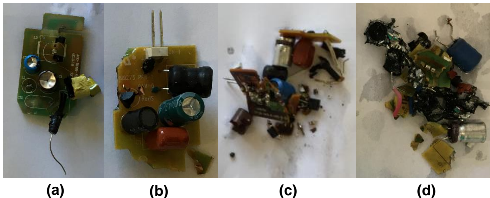
Figure 3-50 : Exemples des états de drivers des E27 : Très bon (a), bon (b), mauvais (c) et très mauvais (d)
