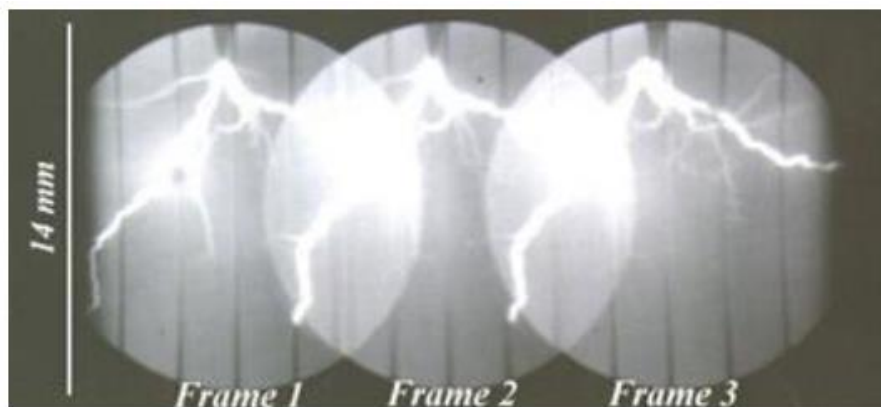
Figure 3-5 : Convertisseur d'images d'une décharge électrique supersonique dans l'eau (polarité positive) \sigma = 200 \mu\text{S/cm} et temps d'exposition 200 ns [32]
