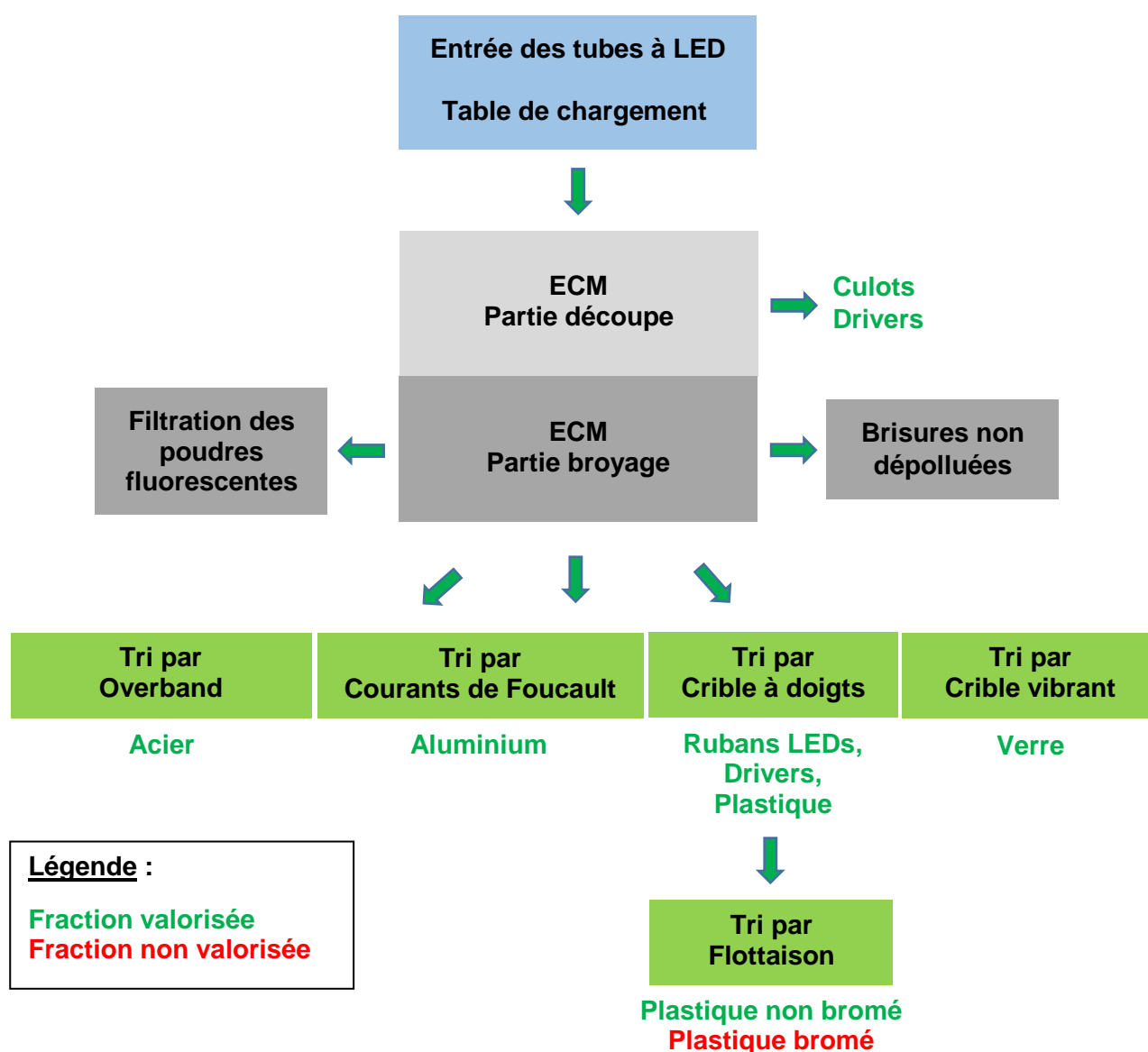
Figure 1 : Synoptique de l'outil ECM pour le traitement en fin de vie des tubes à LED en aluminium, plastique et verre
