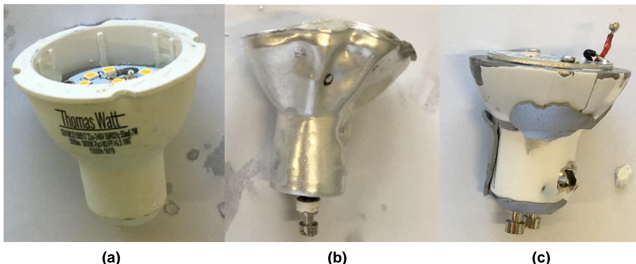
Figure 3-58 : Exemples de photographies de l'état des corps par la fragmentation sélective des GU10 : Corps non détérioré (a), corps enfoncé-non percé (b) et corps enfoncé-percé (c)
