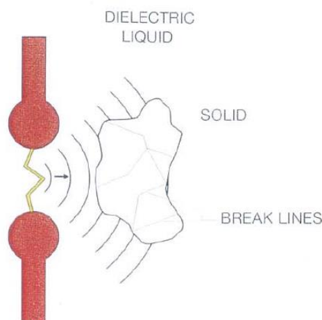
Figure 3-13 : Schématisation du principe de la fragmentation par compression à travers l'onde de choc : IMPULSTEC (lower voltages) [17] [18]
