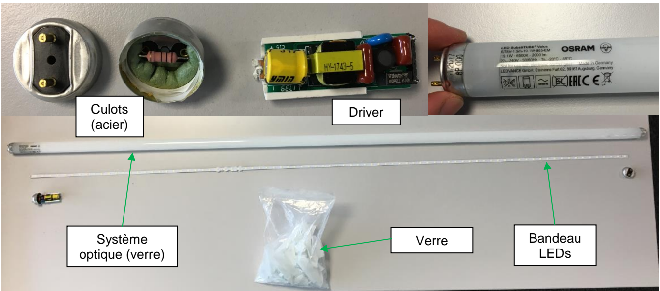
Figure 5 : Désassemblage manuel d'un tube à LED verre OSRAM, 19,1 W, 150 cm, 6500 K, masse 236 g et 84 puces LEDs (fabrication 2014)
