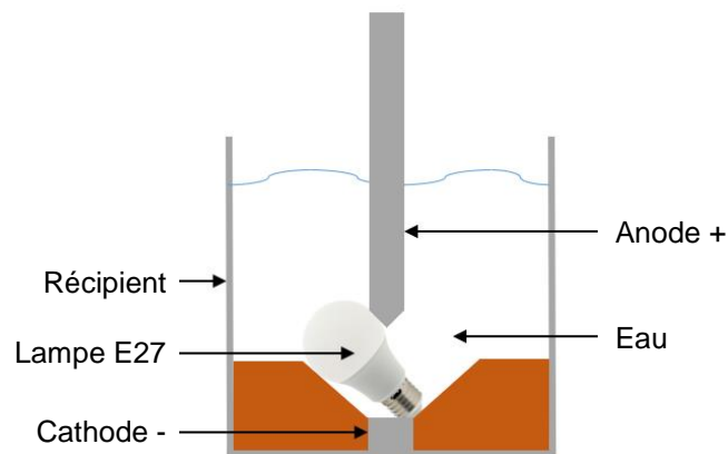
Figure 3-32 : Schéma de la disposition de la lampe E27 dans le récipient
