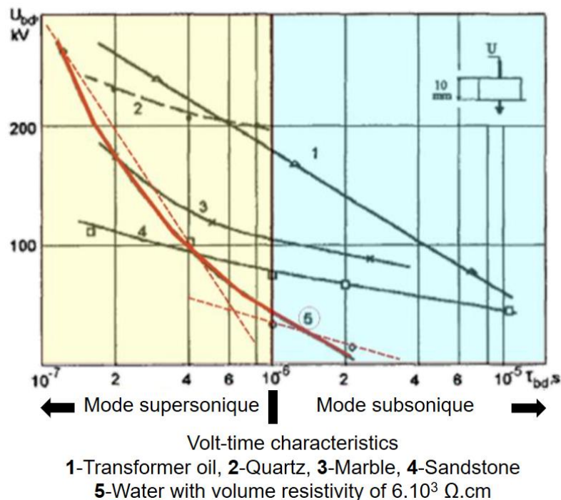
Figure 3-2 : Evolution de la tension de claquage en fonction de la durée d'application [29]
