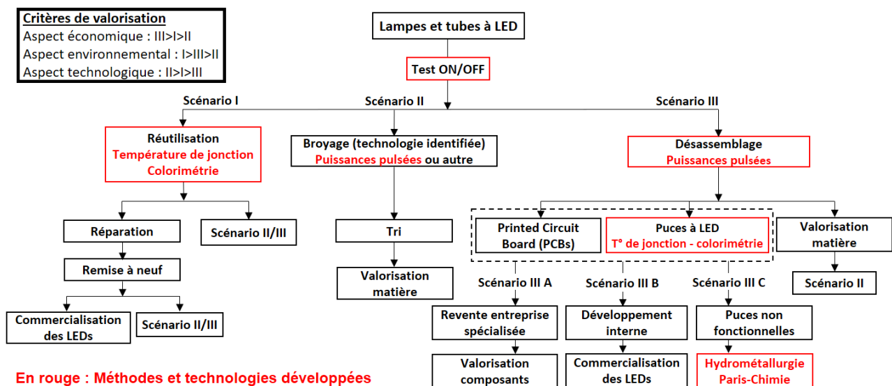
Figure 1-11 : Différents scénarii envisagés et procédés associés pour le recyclage des lampes à LED [13]
