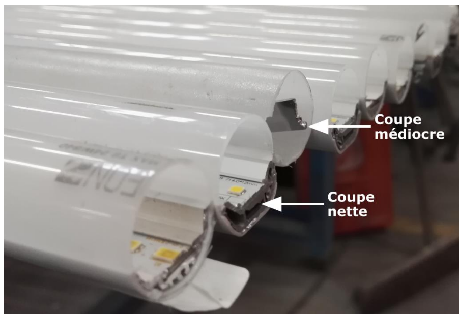
Figure 3-72 : Photographie d'illustration des découpes des tubes à LED en plastique à l'ECM [55]
