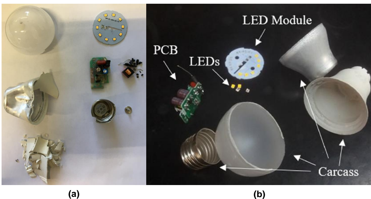
Figure 4-28 : Exemples de lampes E27 en plastique désassemblées : Sélectivement au SELFRAG Lab (a) et manuellement (b) [30]
