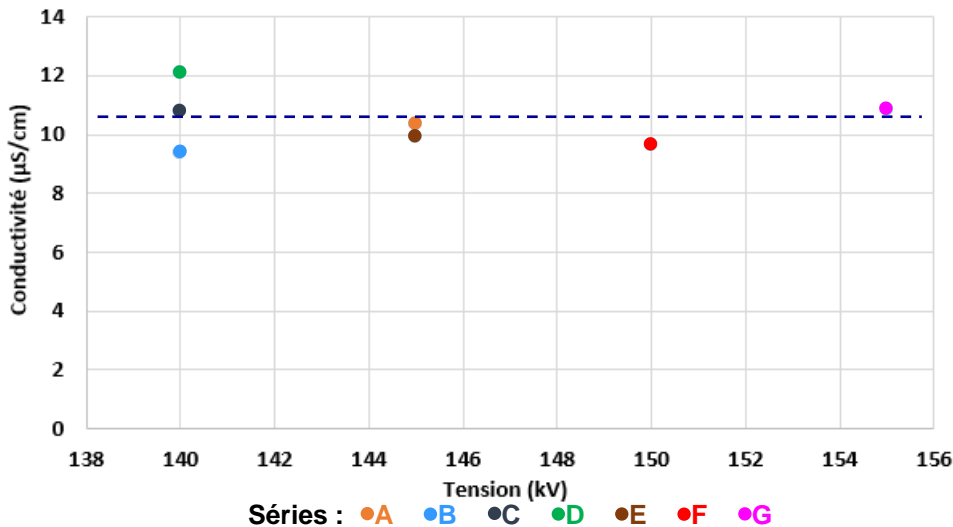
Figure 3-39 : Conductivité en fonction de la tension, pour les 7 séries favorables des couples tension-nombre de pulses
