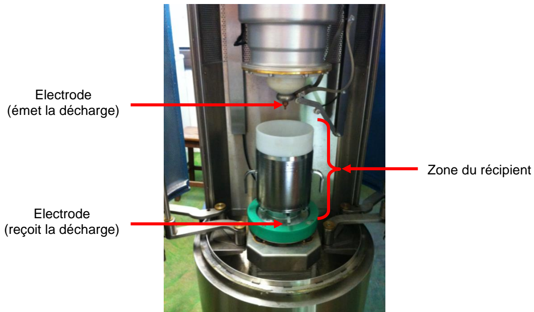
Figure 3-31 : Photographie du récipient dans le SELFRAG Lab
