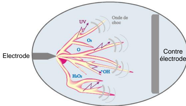
Figure 3-1 : Illustration des différents effets produits par une décharge « streamer » dans l'eau [28]
