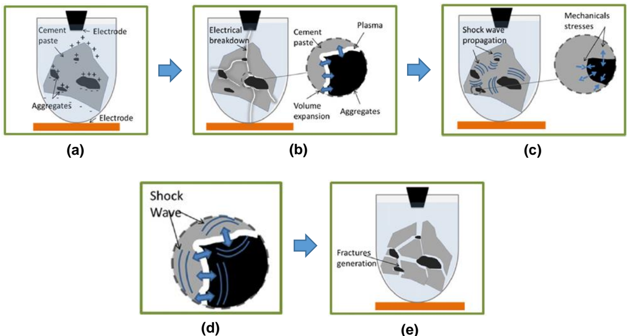
Figure 3-12 : Schématisation du principe de la comminution par EDF du SELFRAG Lab [6]
