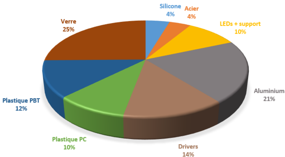
Figure 2-28 : Composition moyenne d'une lampe à LED commercialisée en 2020 (lampes E27, E14, E40 et spots GU10)
