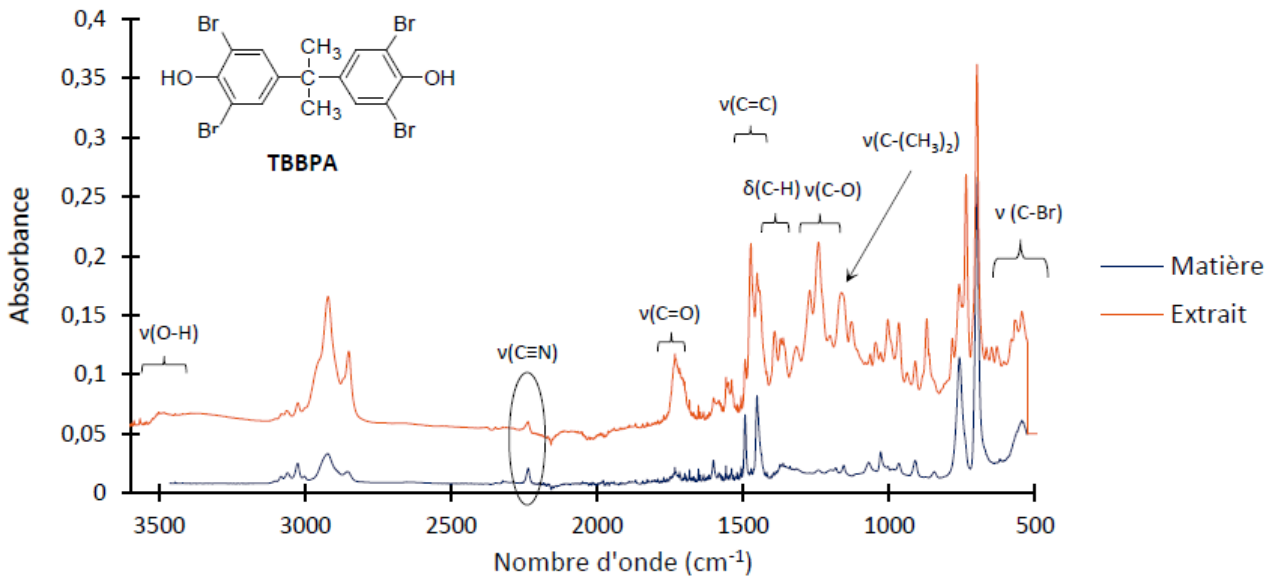
Figure 4-10 : Spectres IR du TBBPA extrait et dans la matière (ABS) après dissolution-précipitation [21]
