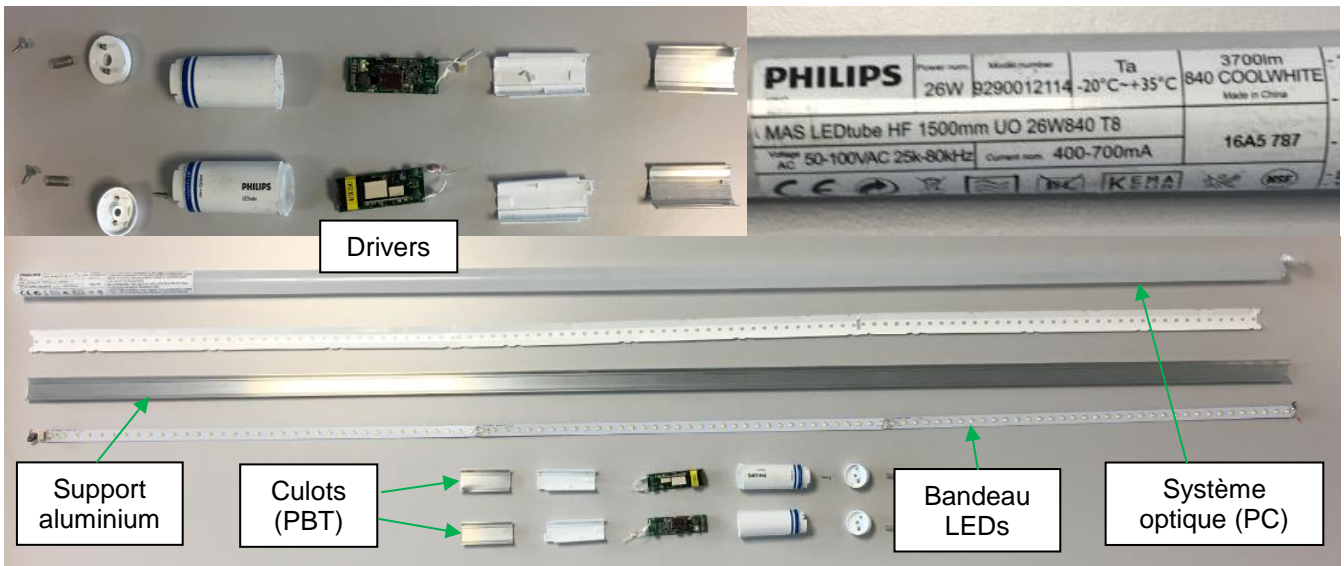
Figure 4 : Désassemblage manuel d'un tube à LED plastique Philips, 26 W, 150 cm, masse 310 g et 108 puces LEDs
