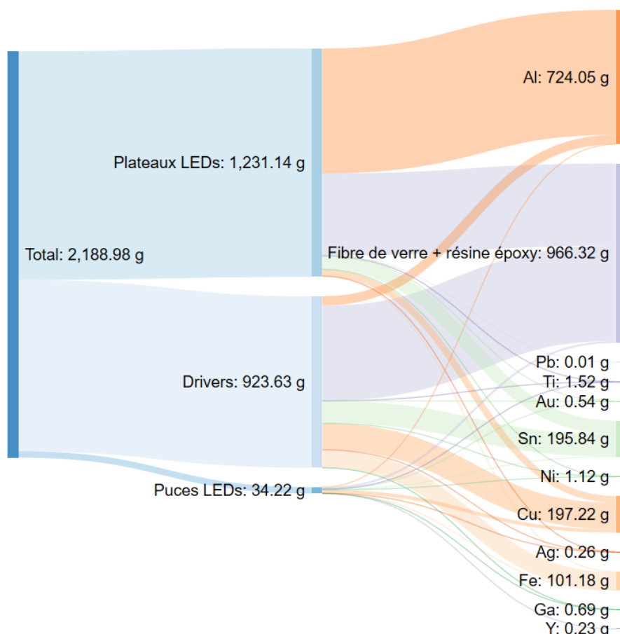
Figure 3-36 : Diagramme de Sankey des métaux précieux et stratégiques récupérés dans les plateaux LEDs, les drivers et les puces LEDs des lampes E27 en plastique, pour la totalité des essais
