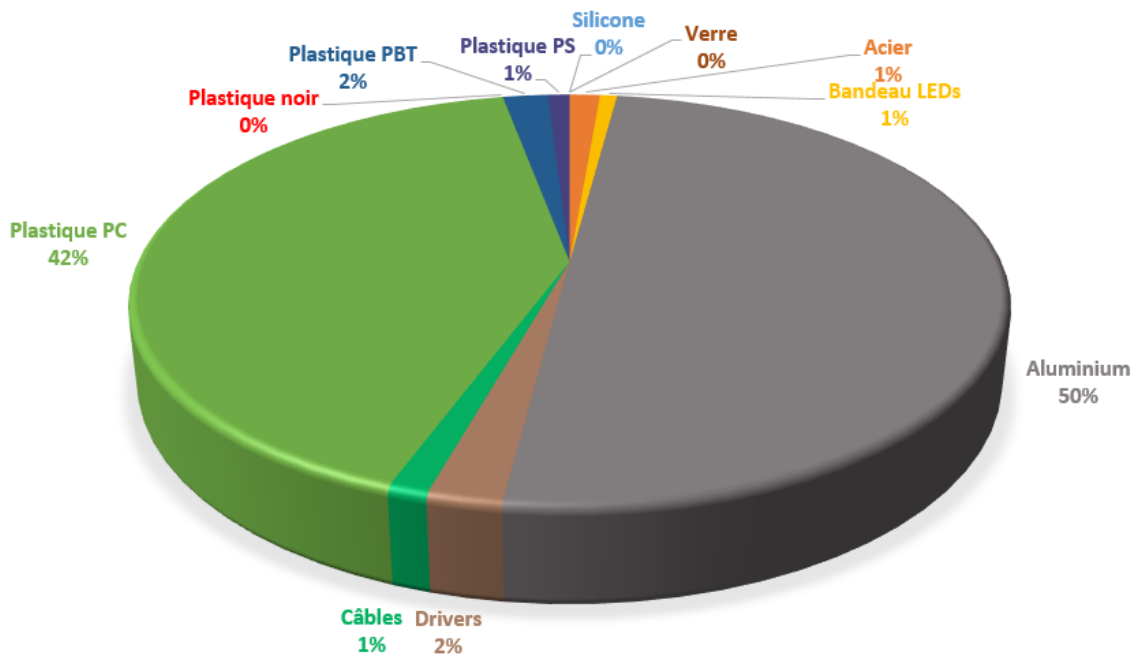
Figure 2 : Composition moyenne d'une dalle à LED 120 x 30 (technologie 2020)
