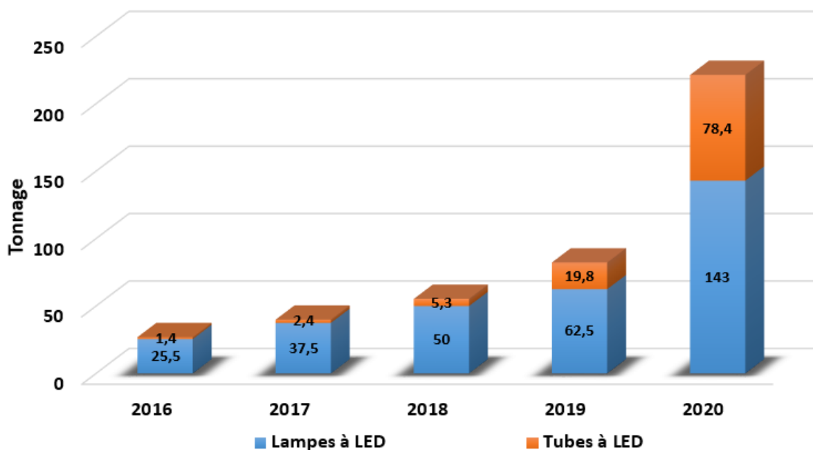
Figure C : Tonnages des systèmes d'éclairage à LED stockés chez ARTEMISE
