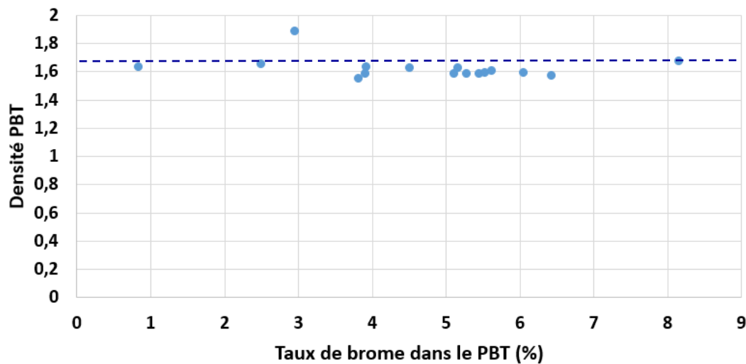
Figure 4-8 : Densité de la matrice PBT en fonction de la concentration de brome
