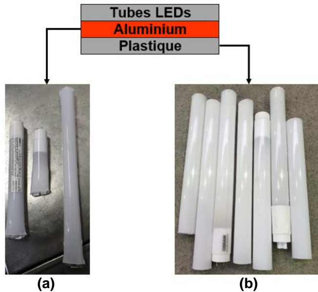
Figure 3-24 : Tubes à LED avec socles en aluminium (a) et en plastique (b)
