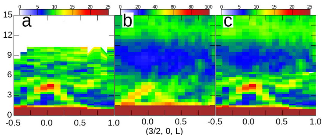
Figure 5.2 – Dispersion mesurées le long de la direction (1.5,0,L) pour k_f=2 \text{ \AA}^{-1} (2T@LLB) fig. a) et k_f=2.5 \text{ \AA}^{-1} (4F@LLB) fig. b. La figure c montre la synthèse des deux, en conservant les mesures à petit k_f pour les basses énergies et à grand k_f pour les hautes.
