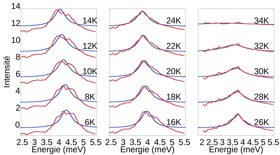
Figure 4.6 – Spectres d'absorption (en rouge) dans la configuration E||b||H||a pour différentes températures de 6 à 40 K, en prenant comme référence ( I_0 ) le spectre obtenu à 45 K. Les courbes en bleu correspondent à un fit par une Lorentzienne unique.
