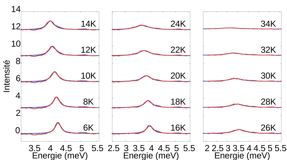
Figure 4.4 – Spectres d'absorption (en rouge) dans la configuration E a H b pour différentes températures de 6 à 40 K par pas de 2 K, en prenant comme spectre référence ( I_0 ) le spectre obtenu à 45 K. Les courbes en bleu correspondent à un fit par une Lorentzienne unique.
