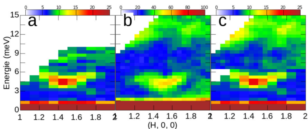
Figure 5.3 – Dispersion mesurées le long de la direction (H,0,0) pour k_f=2.667 \text{ \AA}^{-1} (2T@LLB) fig. a) et k_f=1.97 \text{ \AA}^{-1} (4F@LLB) fig. b. La figure c montre la synthèse des deux, en conservant les mesures à petit k_f pour les basses énergies et à grand k_f pour les hautes.
