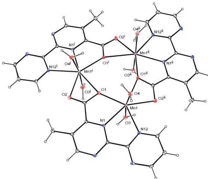
Figure 22. Structure moléculaire de la brique cationique [\text{Mn}_3(\text{bpymca})_3(\text{H}_2\text{O})_6]^{3+} . [125]
