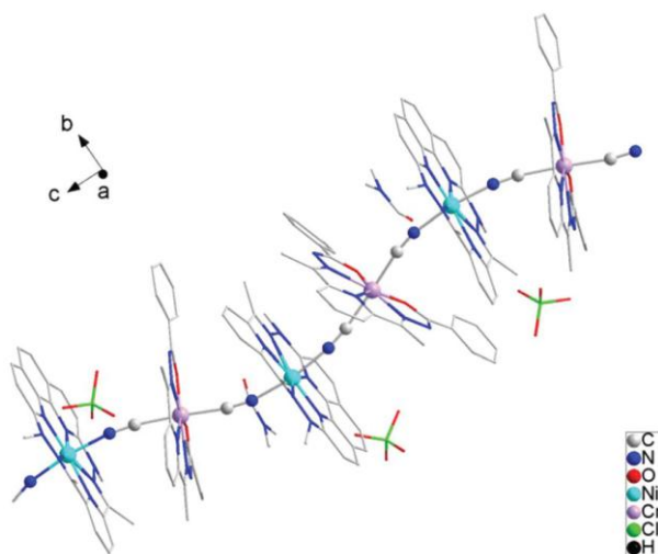
Figure 11. Arrangement moléculaire de la chaîne-aimant 1D- [\text{Ni}(\text{L}^{\text{N}5\text{PhenMe}})\{\text{Cr}(\text{L}^{\text{N}3\text{O}2\text{Ph}})(\text{CN})_2\}]\cdot\text{ClO}_4 . [63]
