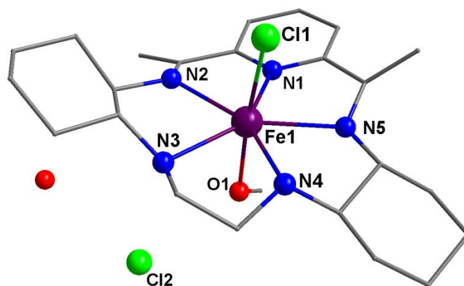
Figure 7. Structure moléculaire du complexe [Fe(L^{N5RR/SS})(MeOH)Cl]Cl.H_2O ( 5^R )
