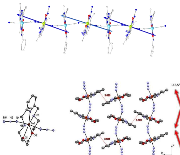
Figure 12. SCMs impliquant des centres PBP Fe^{II} comme source d'anisotropie magnétique. (haut) 1D-[\{Fe(H_2L^{N3O2NH2})\}_2CrL^{(N3O2Ph)}(CN)_2].PF_6 avec l'axe de facile aimantation des Fe^{II} représenté sous forme de flèches bleues ( Fe en vert, Cr en bleu clair, à partir de Ref.97), (en bas) 1D-[FeL^{N3O2H}(N_3)]ClO_4 , les flèches rouges matérialisent l'axe de facile aimantation d'un centre Fe^{II} positionné le long de l'axe N_{azido}-Fe-N_{azido} , mettant ainsi en évidence l'angle d'inclinaison à l'origine d'un faible ferromagnétisme et d'un comportement de SCM [98] .
