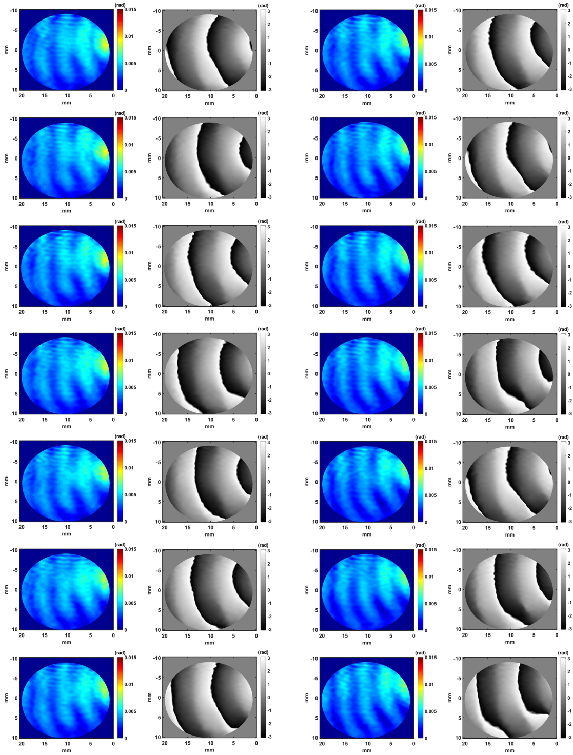
FIGURE 3.18 – Amplitude et phase du champ acoustique à 0 mm selon la vue R, 14 projections de 70^\circ à 135^\circ avec un incrément de 5^\circ .
