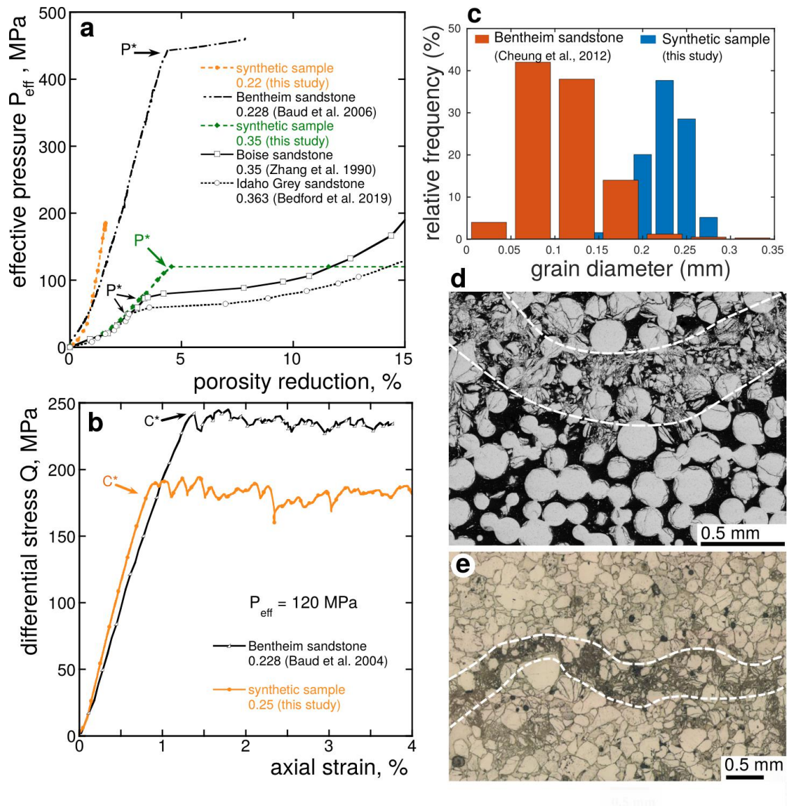
Figure 4 Résultats d'expériences de déformation sur des échantillons de synthèse comparés à des résultats d'expériences de déformation sur un grès naturel, le grès de Bentheim. (a) Comparaison des résultats de la compression hydrostatique d'un échantillon synthétique monodisperse (vert pointillé) avec une porosité de 0.35 et un diamètre de grains de 0.5 mm et
