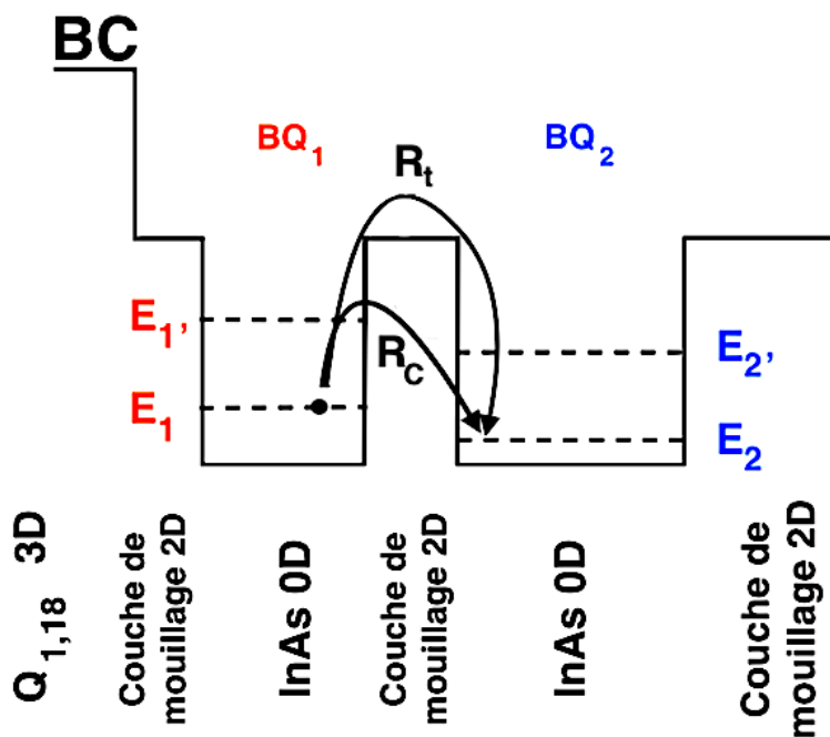
Figure 4-1: Représentation schématique du diagramme en énergie de la bande de conduction BC pour deux boîtes quantiques adjacentes couplées appartenant à deux familles différentes notés 1 et 2.
