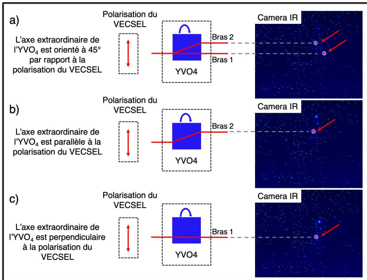
Figure 2-28: Orientation du cristal biréfringent \text{YVO}_4 en dehors de la cavité laser à l'aide d'une caméra infrarouge. a) Polarisation linéaire en sortie du VECSEL orientée à 45^\circ par rapport à l'axe extraordinaire du cristal biréfringent. b) Polarisation en sortie du VECSEL parallèle à l'axe extraordinianire du cristal \text{YVO}_4 . c) Polarisation en sortie du VECSEL perpendiculaire à l'axe extraordinaire du cristal \text{YVO}_4 .
