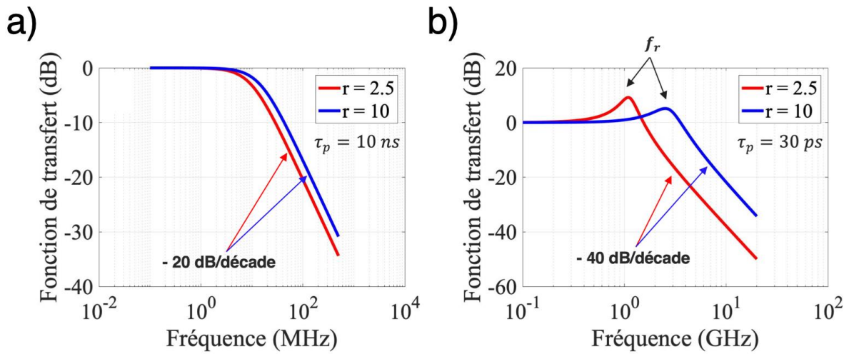
Figure 3-1: Fonctions de transfert d'un laser classe A (a) et classe B (b) pour deux valeurs de taux de pompage r = 2.5 et r = 10 . \tau_c = 1 \text{ ns} .
