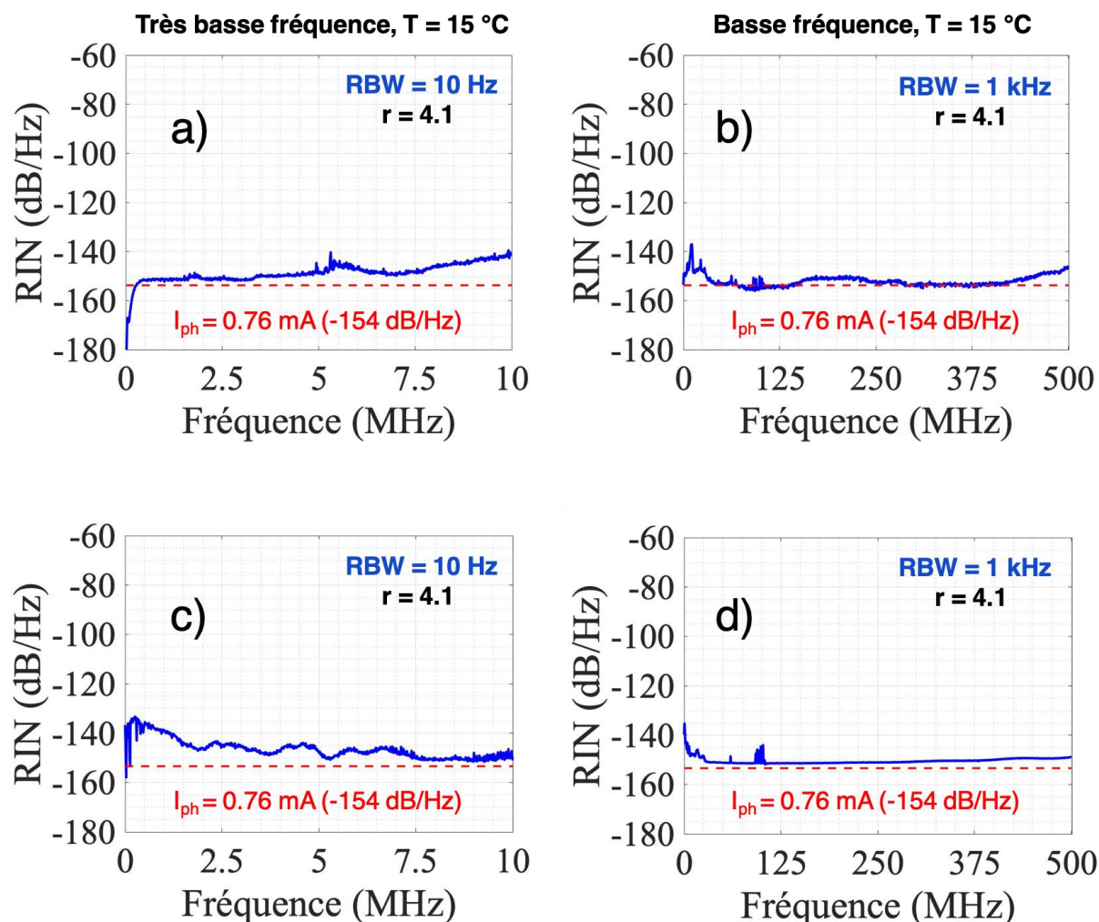
Figure 5-5: a) et c) Spectres de RIN à très basse fréquence, RBW = 10 Hz. b) et d) Spectres de RIN à basse fréquence, RBW = 1 kHz. Les traits en pointillée rouge représentent le bruit de grenaille pour un photocourant détecté de 0.76 mA.
