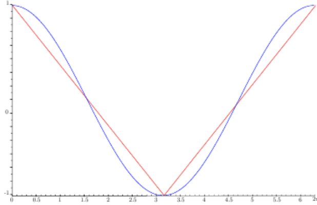
FIGURE 1 – En bleu, \cos , en rouge le signal triangulaire qui l’interpole.
