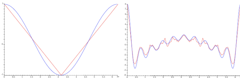
FIGURE 2.2 – À gauche, les fonctions cosinus (en bleu) et triangle (en rouge), à droite deux réalisations des signaux S_{10} associés pour des coefficients de loi de Rademacher.
