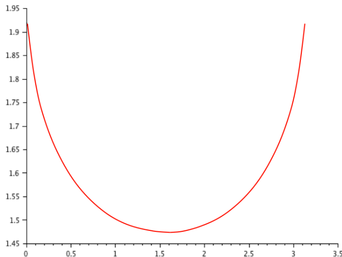
FIGURE 2.1 – Graphe de la fonction x \mapsto \ell^{1/2}(x)
