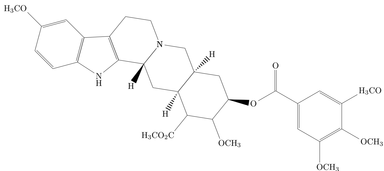
FIGURE 3 – Représentation plane de la réserpine (C 33 H 40 N 2 O 9 )
