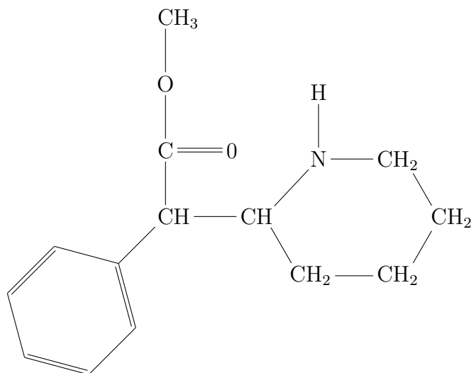
FIGURE 20 – Méthylphénidate (C 14 H 19 NO 2 )
