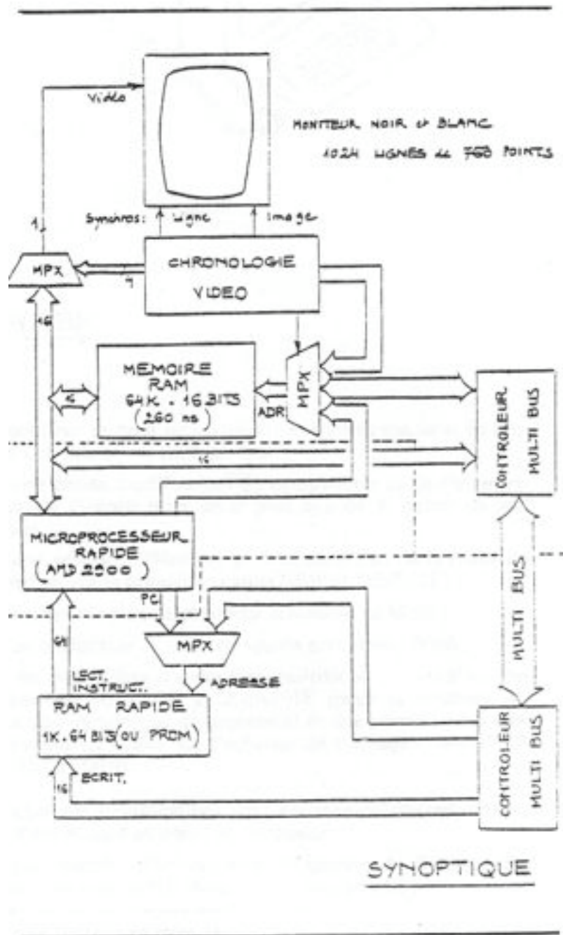
Figure 31. Synoptique du système Kayak 29
