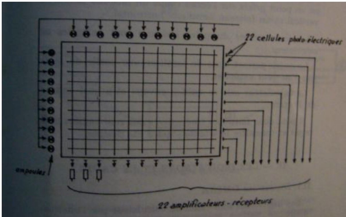
Figure 16. Schéma de fonctionnement du Digitatron 15 .
