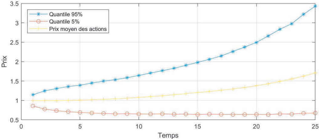
Figure III.23 : courbe de volatilités du modèle actions diffusé avec le modèle HW 2
