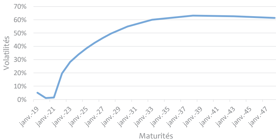
Figure III.8 : volatilité log-normale du cap ATM observé au 02 janvier 2018
