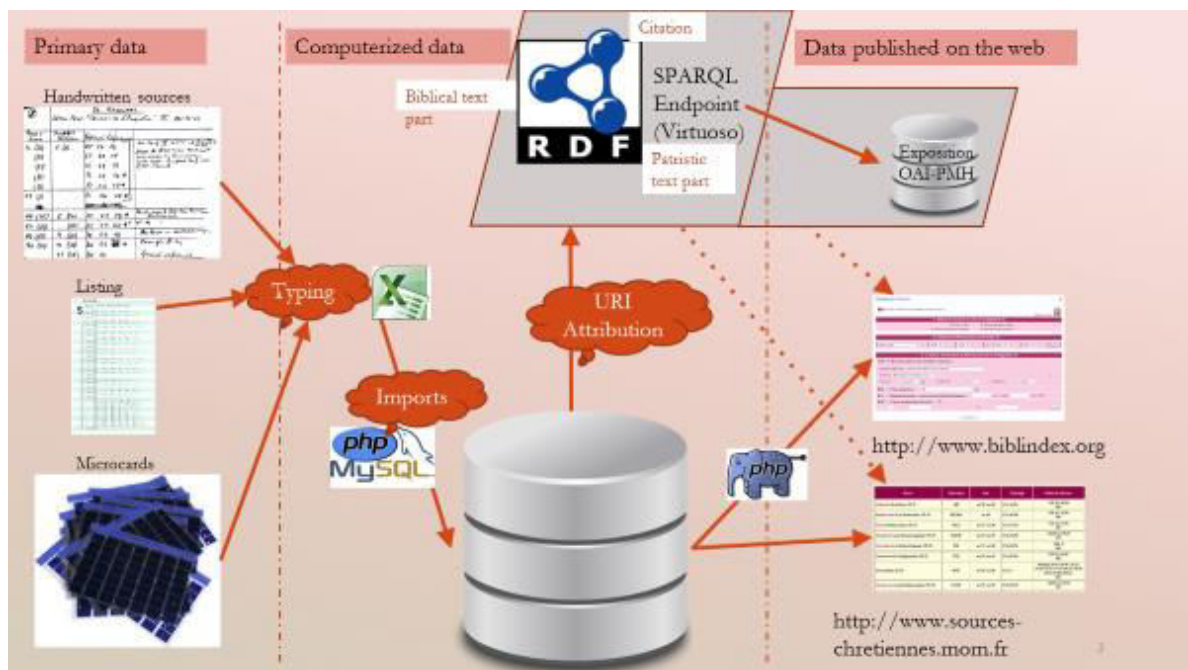
Image 4. Architecture du projet BIBLINDEX.
