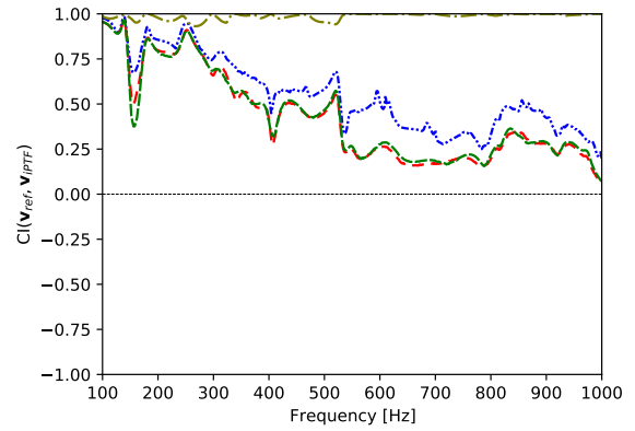
(d) u-iPTF CI fp = 480
