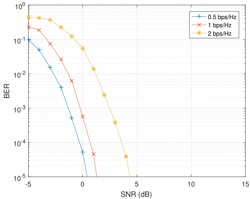
FIGURE 4 – Performance TEB du système DSTM MIMO 8 \times 8 pour différentes efficacités spectrales utilisant \mathcal{G}_{wee8}
