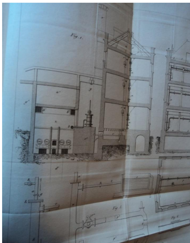
Figure 10 : « Coupe d'une machine à vapeur », Grouvelle et Jaunez, Guide du chauffeur et du propriétaire de machine à vapeur, op. cit. , planches additives.
