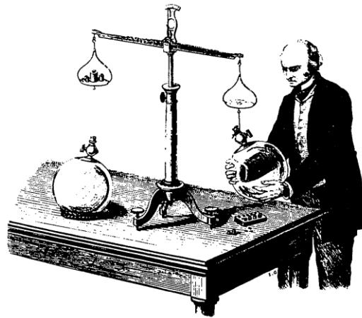
Démonstration du poids des gaz.
