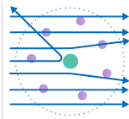
Figure 16 : Modèle de Rutherford.
