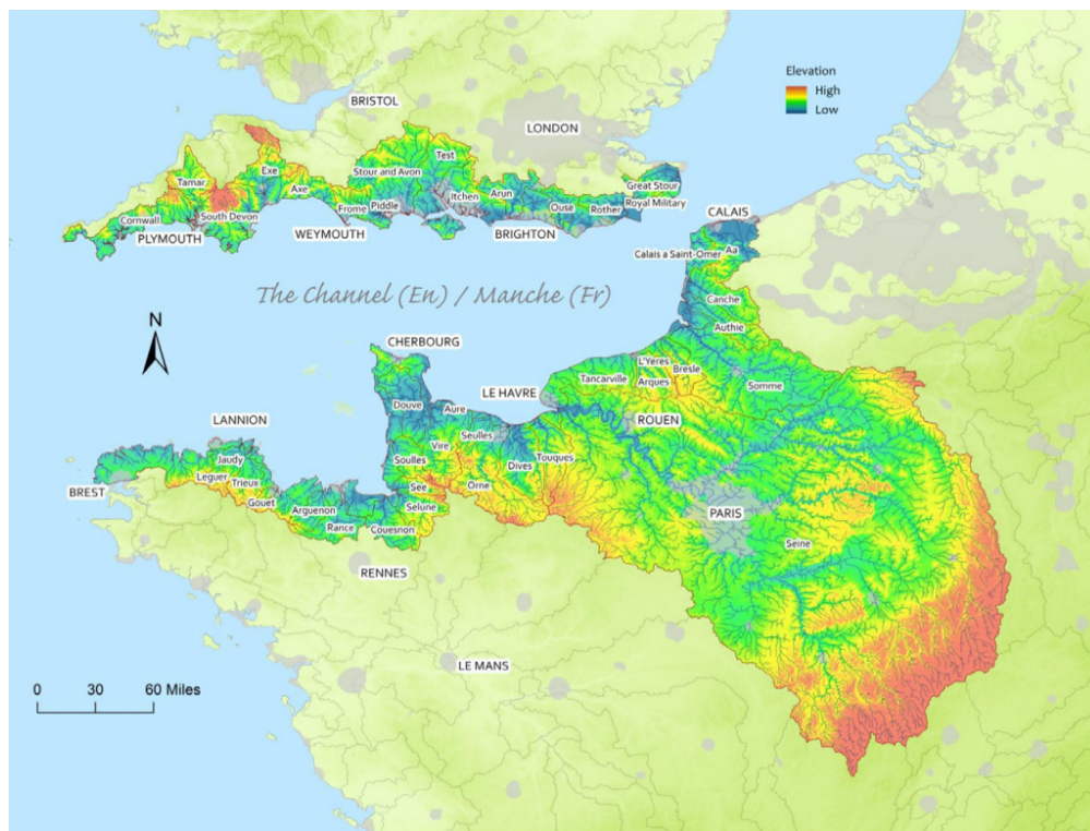
FIGURE 1.14 – Carte des différents bassins versants anglais et français se déversant dans la Manche (extrait de Millward et al. (2015)).
