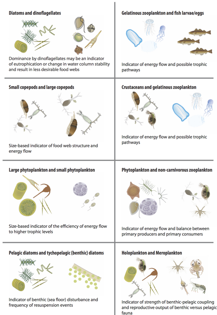
FIGURE 9.5 – Illustration des paires de formes de vies et des stratégies écologiques derrière leur sélection (extrait du rapport OSPAR 2017 ; Changes in Phytoplankton and Zooplankton Communities, décrit dans la publication de McQuatters-Gollop et al. (2019)).
