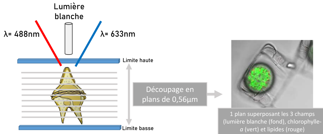
FIGURE 2.7 – Illustration du processus d’acquisition des images par microscopie confocale (gauche) et du résultat obtenu sur un plan (le dessin de Protoperidinium sp. est extraite de la Société Japonaise de Plancton (2011), l’image de Trigonium alternans est issue de l’analyse.)
