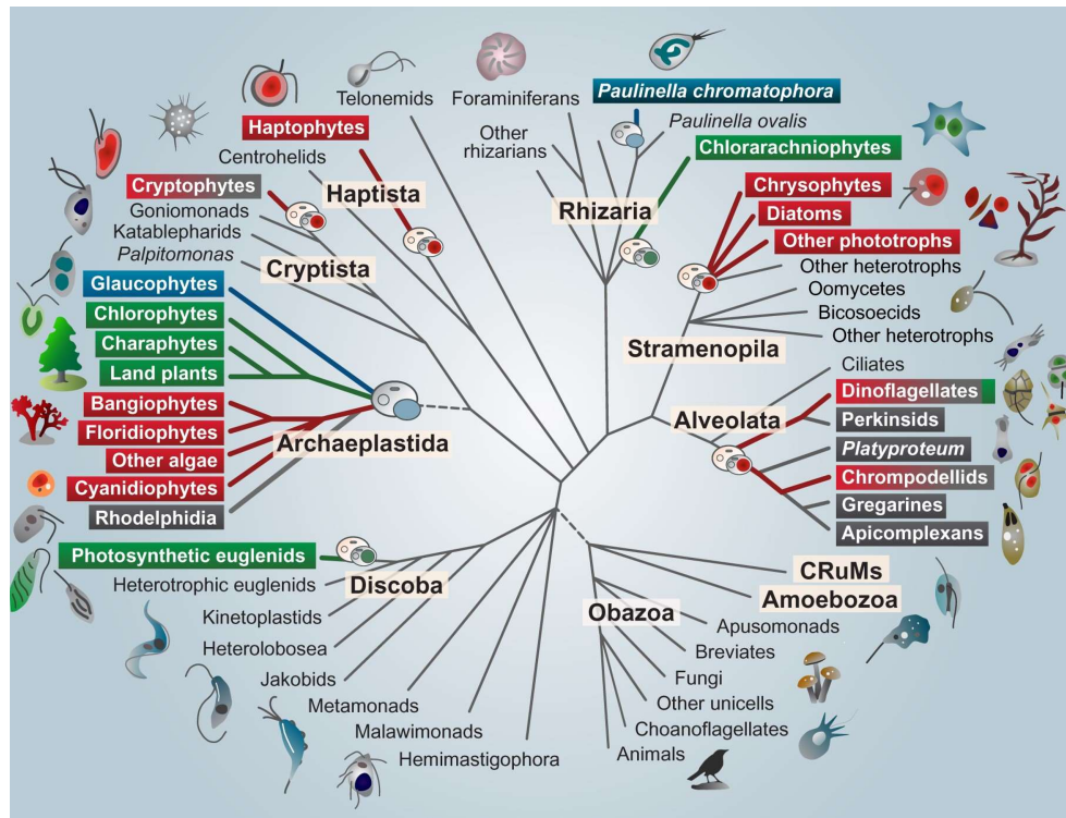
FIGURE 1.2 – Arbre schématique des lignées eucaryotes (organismes photosynthétiques colorés) (McGrath, 2020). Les membres des Archaeplastides ont des plastes primaires provenant directement de cyanobactéries. Les plastes primaires des algues rouges et vertes se sont propagés des Archaeplastides à d'autres branches de l'arbre, notamment celles des Rhizaires, Discoba et Stramenopiles. Les noms de taxons colorés dans ces lignées reflètent l'origine endosymbiotique secondaire ou tertiaire des algues vertes ou rouges de leurs plastes. Les noms de taxons surlignés en gris indiquent la présence d'un ou plusieurs membres secondairement non photosynthétiques.
