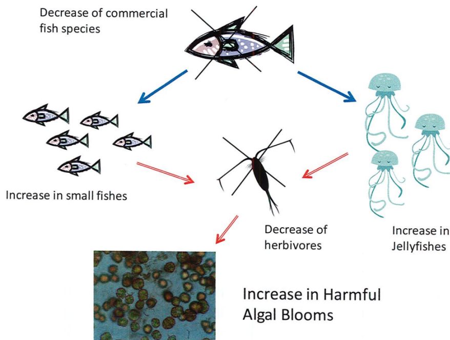
FIGURE 1.11 – Explication possible de l'effet de pêche sur la formation de blooms algaux toxiques, la modification du contrôle 'top-down' des herbivores (repris de Lassus et al. (2016)).
