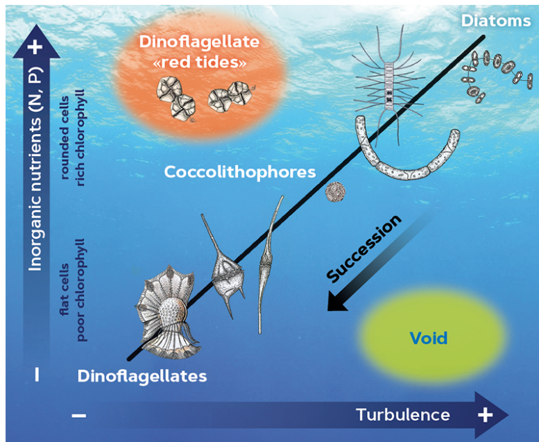
FIGURE 9.2 – Principe du Mandala de Margalef ; représentation schématique de la succession saisonnière des principaux groupes phytoplanctonique selon des axes de turbulences ou de concentrations en nutriments (illustration extraite de Villa et al. (2020)).
