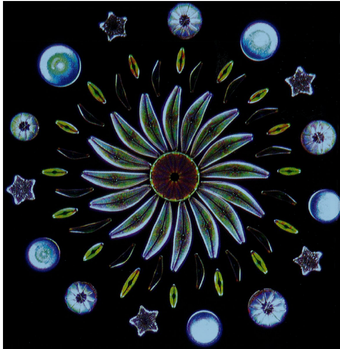
FIGURE 1.4 – Oeuvre du Docteur Osamu Oku, illustrant la diversité morphologique des diatomées (Société Japonaise de Plancton, 2011).
