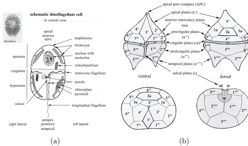
FIGURE 1.6 – (a) Représentation schématique d'un dinoflagellé en vue ventrale. (b) Système Kofoidian pour la désignation des plaques qui forment la thèque des dinoflagellés. (Hoppenrath et al., 2009)
