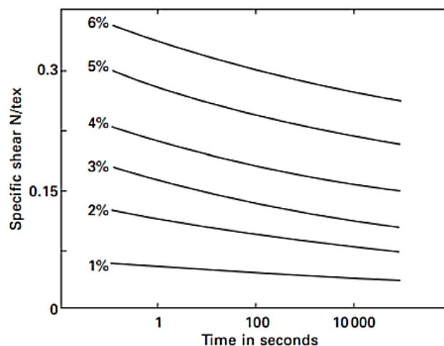
Figure 1. 30 Courbes de relaxation de contrainte du coton à différents taux de déformation à 65% rh, 20°C (Merdeith 1954) [84].
