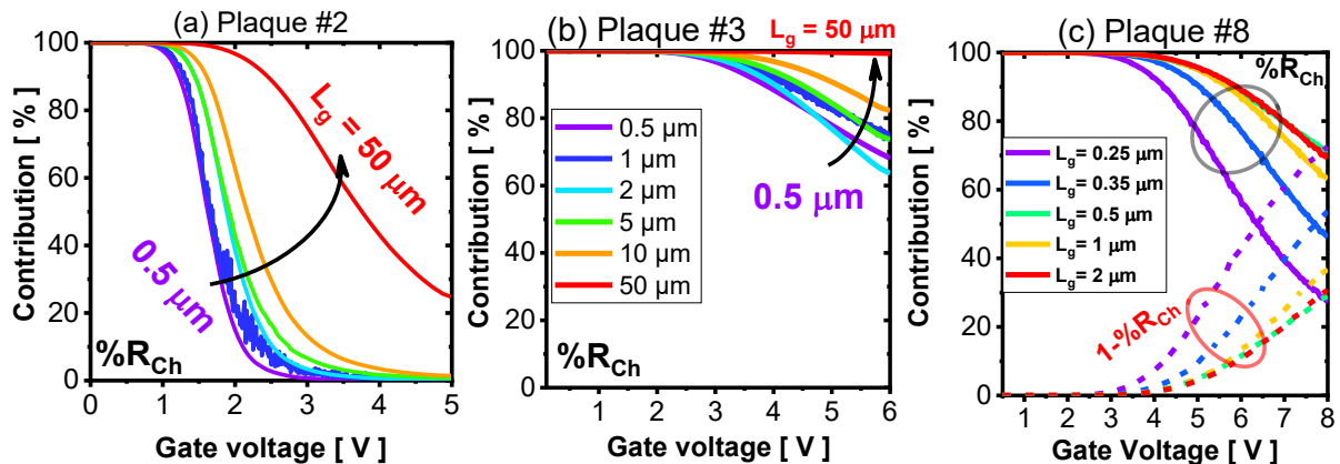
Figure 24: Evolution de la contribution de la variabilité du canal sur la variabilité globale pour les plaques (a) #2, (b) #3 et (c) #9.
