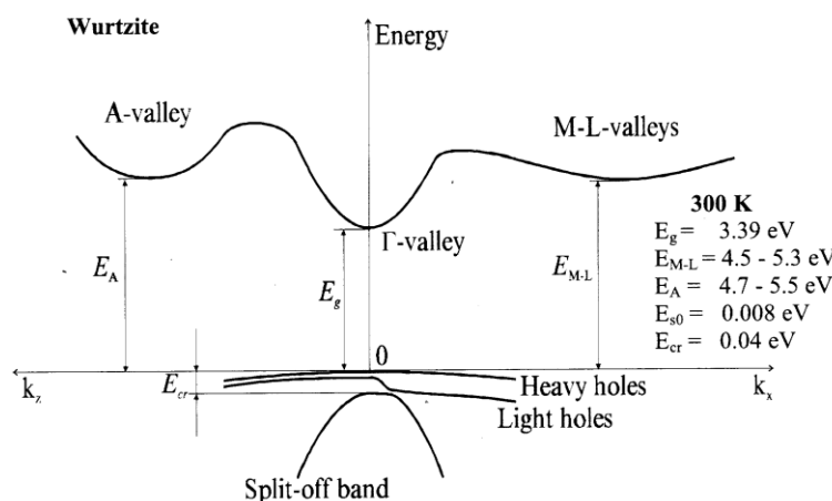
Figure 2 : Diagramme de bande de la structure wurtzite du GaN [2].
