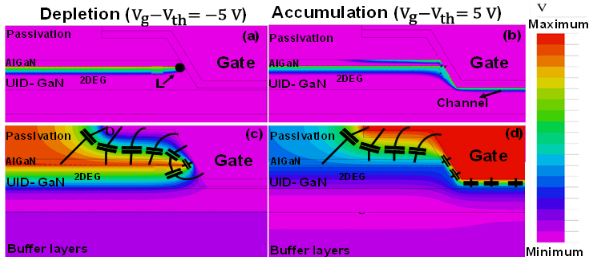
Figure 8: Carte du dispositif GaN générée par le simulateur qui illustre pour deux régimes de fonctionnement (a) et (b) le profil de charge d'électron et (c) et (d) l'évolution du profil de potentiel dans la structure.
