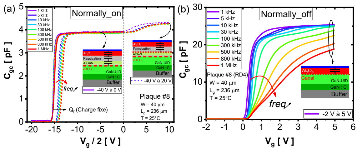
Figure 11: Courbes expérimentales de capacité en fonction de la tension de grille mesurées pour deux dispositifs MIS-HEMT GaN (a) sans et (b) avec gravure locale (Plaquette #8, RD4).
