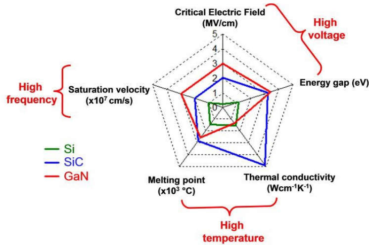
Figure 13: Avantage du GaN par rapport aux autres matériaux Si et SiC [26].
