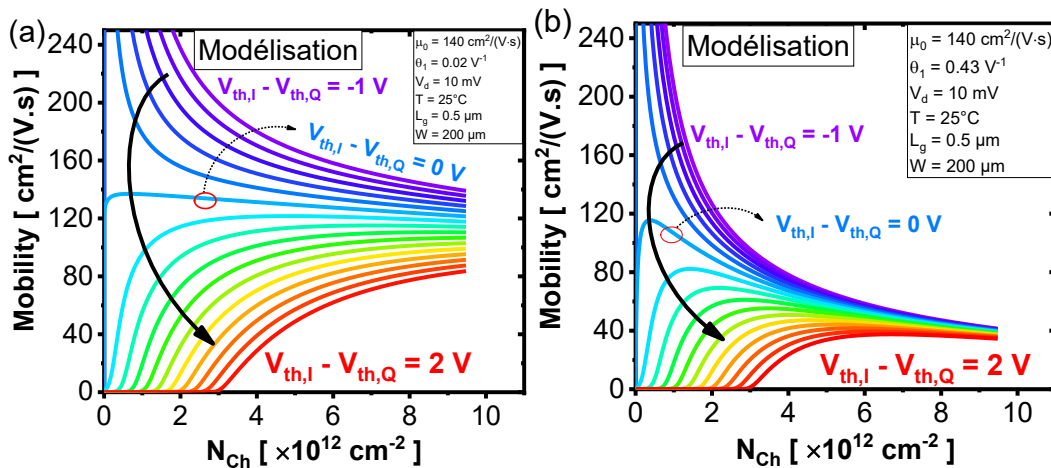
Figure 24: Impact de la différence entre V_{th,I} et V_{th,Q} sur l'évolution de la mobilité (modélisation) obtenue par la méthode CV-split (a) sans et (b) avec effet de résistance d'accès source/drain.
