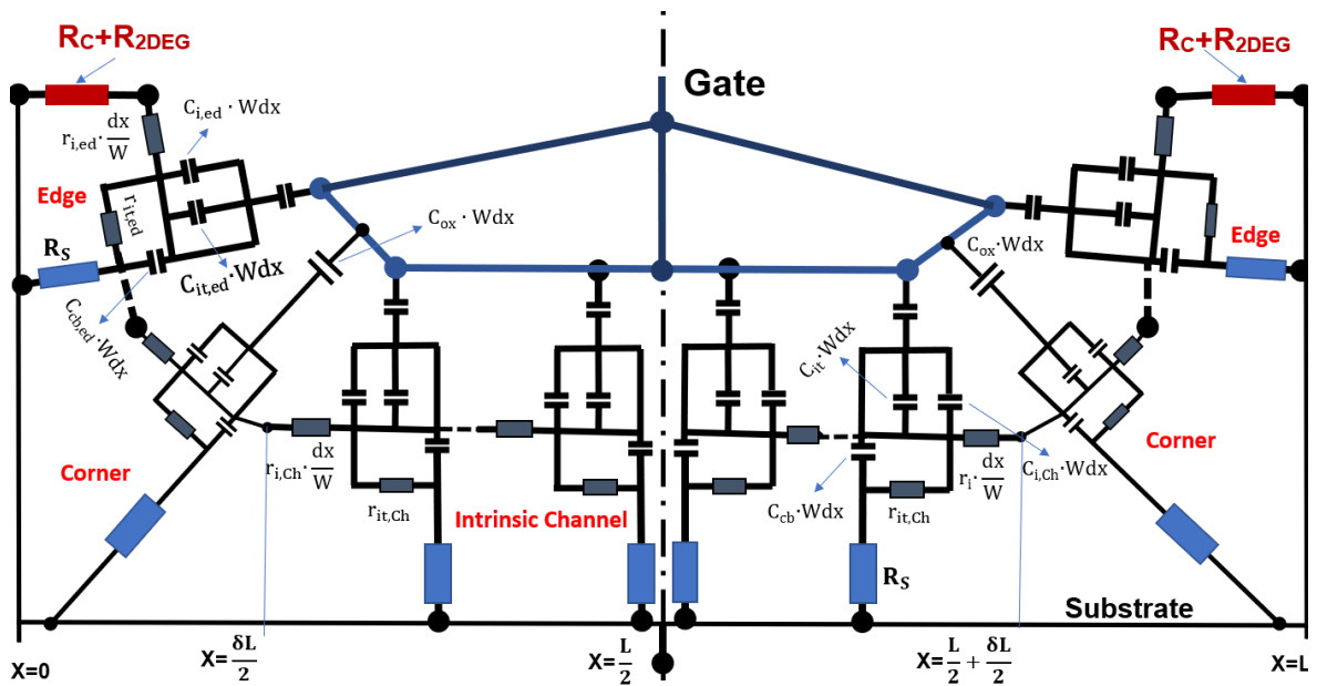
Figure 14: Circuit équivalent petit signal AC de la ligne de transmission du canal de conduction du dispositif MIS-HEMT GaN à grille encastrée.
