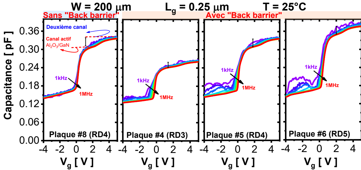
Figure 13: Courbes expérimentales de capacité en fonction de la tension de grille de dispositifs MIS-HEMT GaN mesurées pour différentes profondeurs de gravure.
