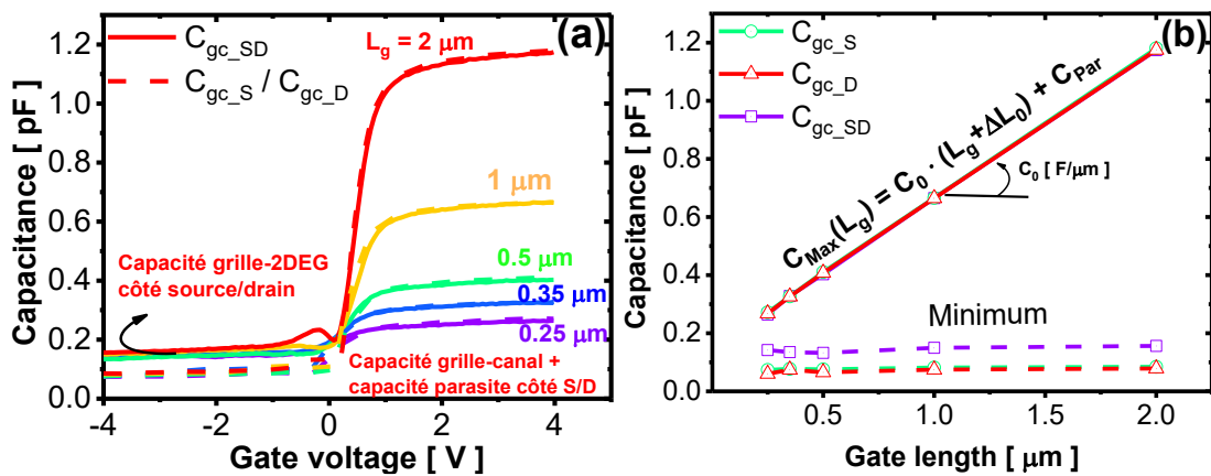
Figure 2: Evolution pour différentes configurations de mesure de la capacité C_{gc} (a) en fonction de la tension de grille V_g et (b) à V_g=4\text{V} en fonction de L_g des dispositifs GaN HEMT à gravure moins profonde ( L_{GS} = L_{GD} = 2 \mu\text{m} , L_{FPg,S} = L_{FPg,D} = 0.25 \mu\text{m} , W=200\mu\text{m} , f=10\text{kHz} et T=25^\circ\text{C} ).
