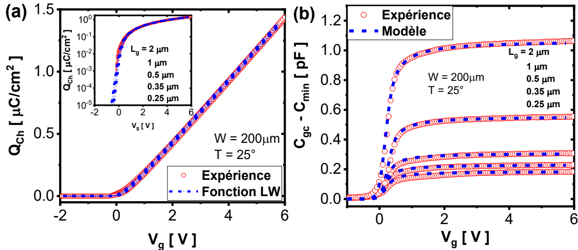
Figure 19: Comparaison pour différentes longueurs de grille de la plaque #8 (expérimentale (symbole) et modèle de Lambert (traits pointillés)), de l'évolution des caractéristiques (a) Q_{gc}(V_g) et (b) C_{gc}(V_g) .
