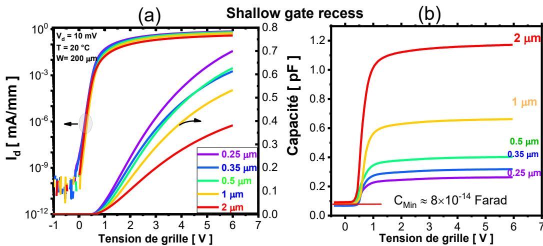
Figure 14: Caractéristique (a) I_d(V_g) et (b) C_{gc}(V_g) des dispositifs MIS-HEMT avec grille encastree de la plaque #4.
