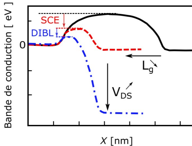
Figure 22: Effet de canal court SCE et de DIBL sur la barrière de potentiel.
