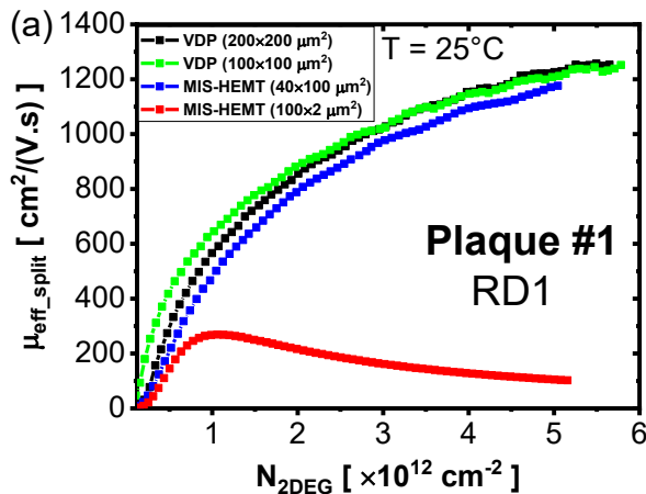
Figure 11: Evolution de la mobilité split-CV en fonction du nombre de porteur libre pour (a) la plaque #1 (RD1) et (b) la plaque #2 (RD2).
