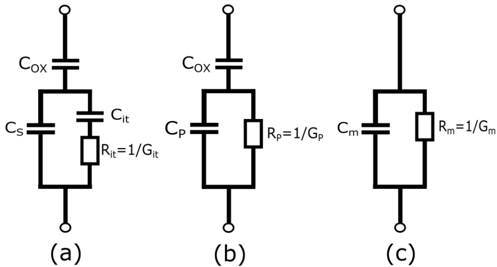
Figure 5: Schéma du circuit électrique équivalent d'un empilement MOS polarisée en régime de déplétion pour un niveau de piège donné où la résistance série est négligeable ; (a) circuit avec pièges à l'interface de constante de temps \tau_{it} = R_{it}C_{it} , (b) circuit simplifié de (a) et (c) circuit mesuré.
