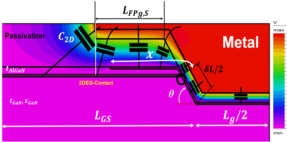
Figure 10: Carte du potentiel dans la structure simplifiée générée par le simulateur 2D FlexPDE montrant le couplage parasite au-dessus du 2DEG.
