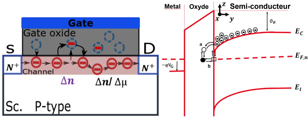
Figure 7: Structure MOSFET (gauche) et diagramme d'énergie montrant les transitions des électrons par effet tunnel entre la bande de conduction et des pièges localisés dans l'oxyde de grille, le processus (a) correspond au tunnel direct et (b) pour un effet tunnel indirect via des pièges d'interface (droite).
