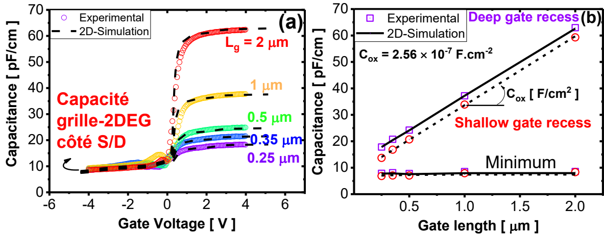
Figure 7: Comparaison entre expérience et simulation de la variation de capacité C_{gc} : (a) en fonction de la tension de grille pour des dispositifs de la plaques #5 et (b) capacité maximales et minimales en fonction de la longueur de grille pour les plaques #4 et #5.
