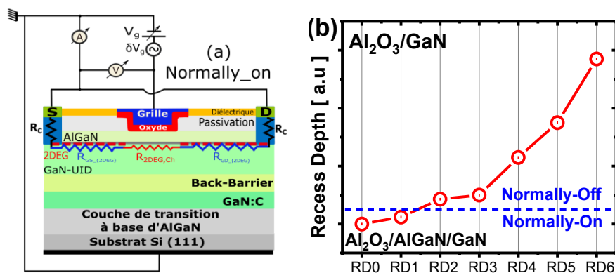
Figure 2: (a) Schéma de mesure de la capacité grille-canal et (b) Illustration de la profondeur de gravure en fonction des symboles.
