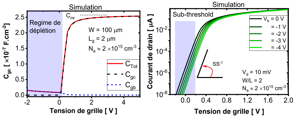
Figure 19: Courbes obtenus par simulation analytique du transistor 1D de la figure 18 en fonction de la tension de grille, (a) de la capacité et (b) du courant de drain.
