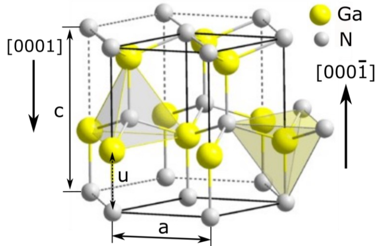
Figure 1 : Structure cristalline wurtzite du GaN [1].
