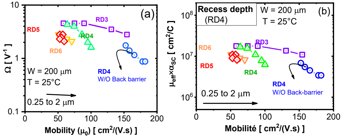
Figure 31: Evolution en fonction de la mobilité du canal intrinsèque \mu_{ch} , (a) du coefficient de mobilité corrélée et (b) du produit du coefficient d'interaction de Coulombienne \alpha_{sc} et la mobilité \mu_{eff} .
