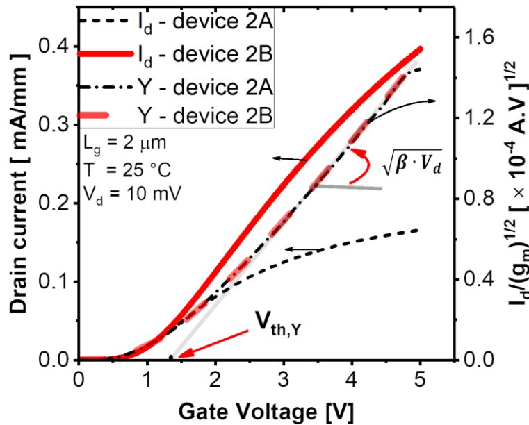
Figure 5: Application de la fonction Y ( I_d/\sqrt{g_m} ) sur des technologies GaN MIS-HEMT pour deux dispositifs A et B sur la plaque #2 ayant différents niveaux de résistances d'accès.
