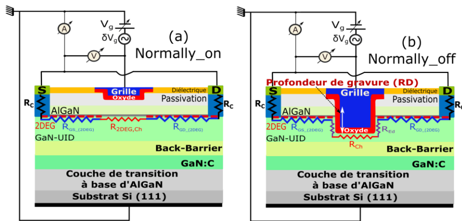
Figure 10: Schéma de montage électrique de la mesure de capacité grille-canal C_{gc} de deux dispositifs (a) normally-on sans gravure de la couche de passivation et (b) normally-off avec gravure locale complète de l'empilement passivation/AlGaN (RD4).
