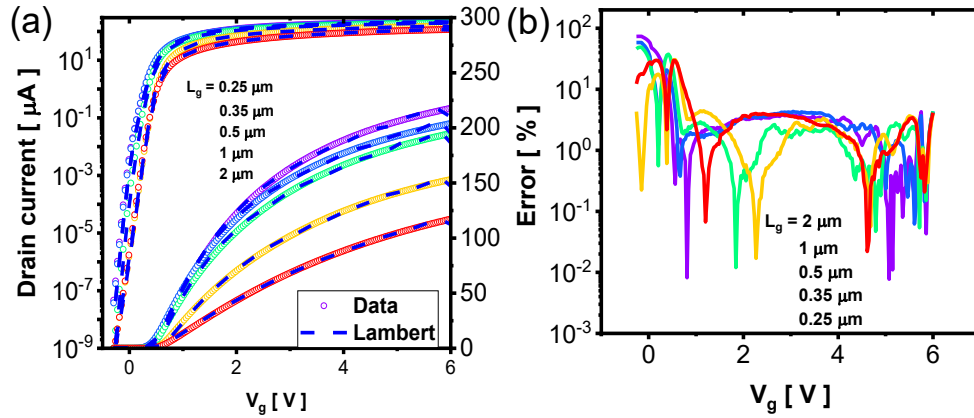
Figure 20: Comparaison pour différentes longueurs de grille de la plaque #8 (expérimentale (symbole) et modélisation (traits pointillés)), de l'évolution des caractéristiques (a) I_d(V_g) et (b) l'erreur en fonction de V_g .
