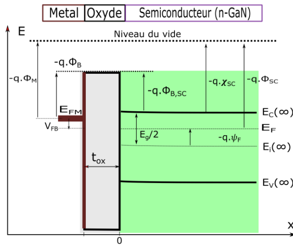
Figure 1: Diagramme de bandes d'une structure MOS idéale en condition de bandes plates V_g = V_{FB} ( \Phi_M \neq \Phi_{SC} ), semiconducteur de type n (cas du GaN).
