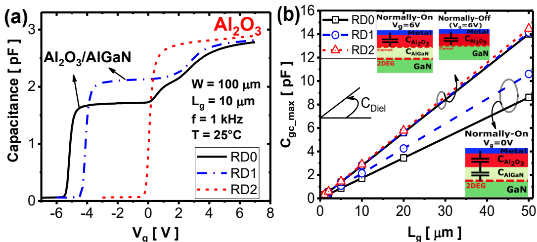
Figure 3: Évolutions : a) en fonction de la tension de grille V_g , de la capacité grille-canal et (b) en fonction de la longueur de grille L_g , de la capacité à V_g=0\text{V} et V_g=6\text{V} pour les dispositifs « normally on » (RD0 et RD1) et V_g=6\text{V} pour les dispositifs « normally-off » (RD2).
