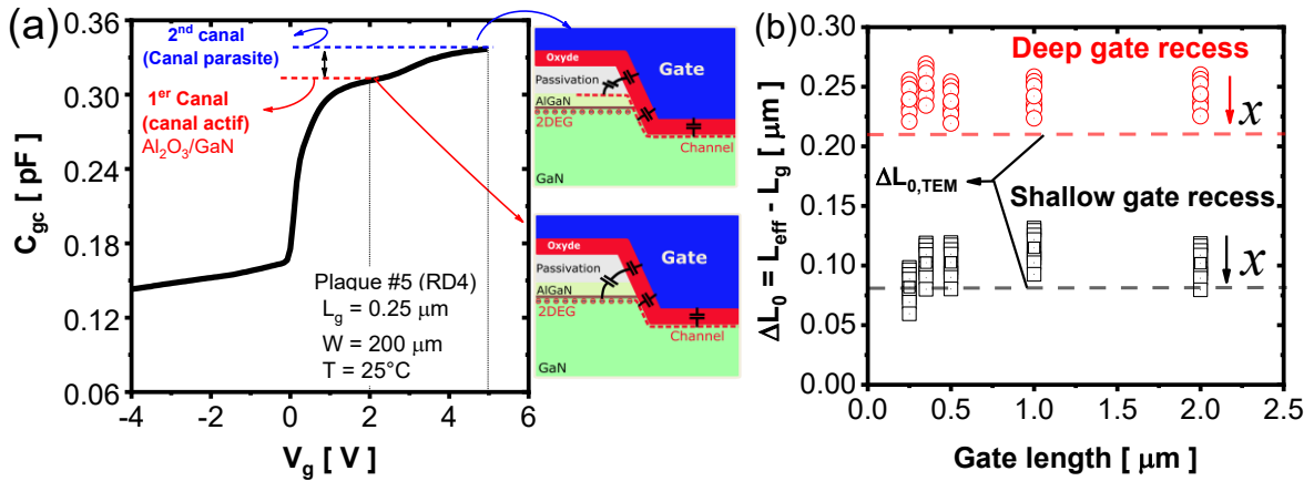
Figure 13: (a) Mise en évidence expérimentale de la formation d'un 2 nd canal sur la caractéristique C_{gc}(V_g) et (b) \Delta L_0 = L_{eff} - L_g en fonction de L_g pour différentes valeurs de capacités parasite qui correspondent à différentes longueurs d'extension x , analyse faite sur les plaques #4 et #5.
