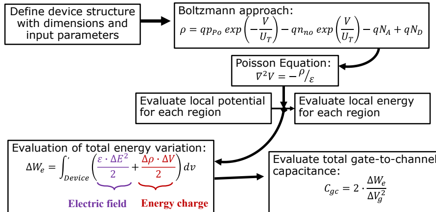
Figure 5: Schéma de principe de la simulation du couplage grille-canal C_{gc} .
