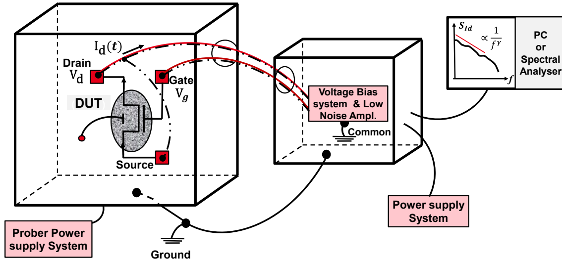
Figure 9: Schéma de principe du système de mesure de bruit basse fréquence utilisé.
