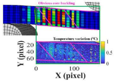
(c) Point B: Dis.=6.2 mm, F=1721 N.
