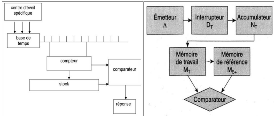
Figure 2. Modèles de l'horloge interne. A gauche, le modèle original de Treisman (1963). A droite le modèle de Gibbon, Church & Meck (1984) illustrant la présence d'un comparateur et montrant les relations avec la mémoire de travail et la mémoire de référence
