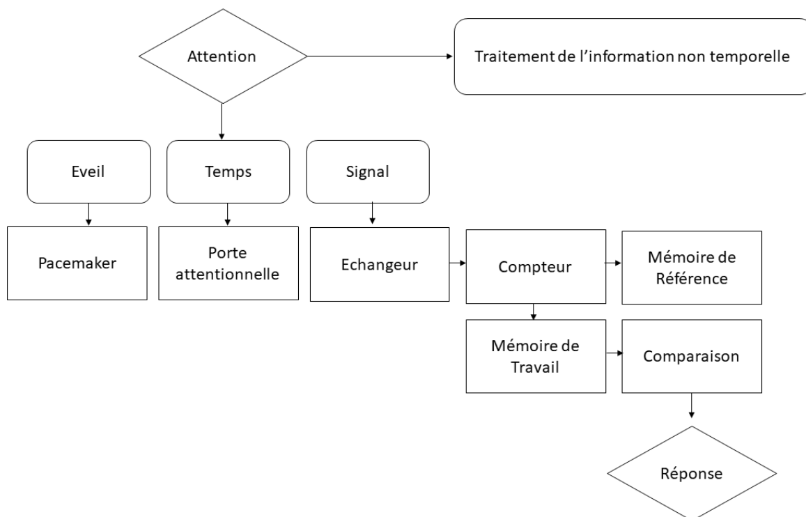
Figure 3. Modèle de la porte attentionnelle (Block & Zakay, 1996)
