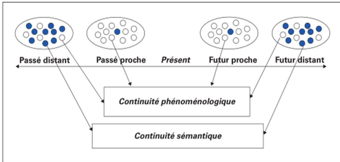
Figure 5. Modèle TEDIFT (La Corte & Piolino, 2016)
