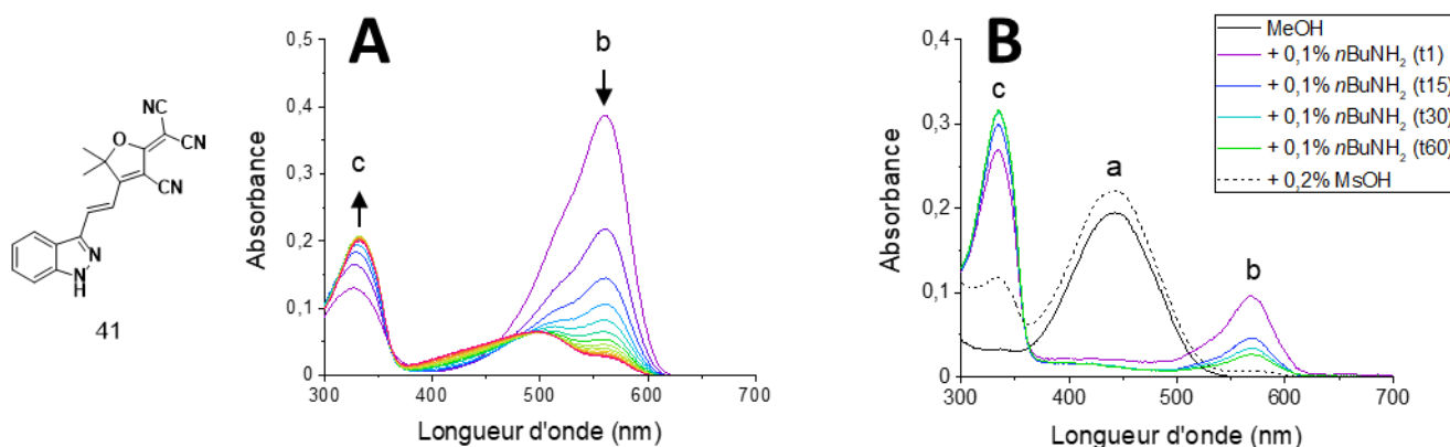
Figure 62 : A) Stabilité du composé avec l'accepteur TCF 41 en milieux aqueux basique ; B) Evolution de son spectre d'absorption après ajout de base puis d'acide dans le méthanol.
