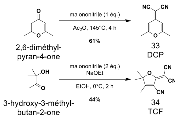
Schéma 22 : Conditions réactionnelles pour la synthèse des accepteurs de type polynitrile.
