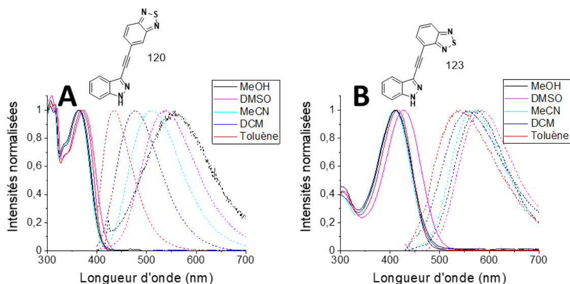
Figure 95 : A) & B) Spectres d'absorption (traits pleins) et d'émission (traits pointillés) dans différents solvants des composés de structure D-alcyne-A, où D est un 1H-indazole 120 et 123 , respectivement.
