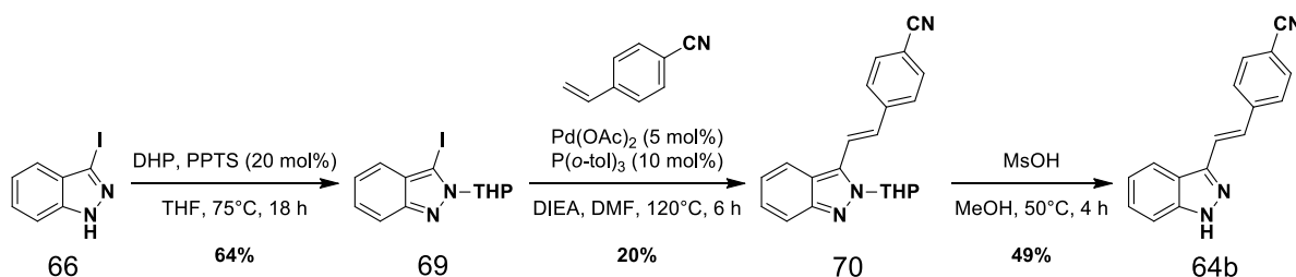
Schéma 41 : Synthèse de la sonde 64b par couplage de Heck sur un indazole protégé en position 2.
