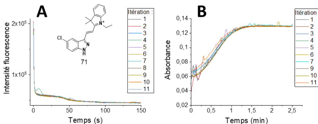
Figure 64 : Cinétiques de : A) la disparition de fluorescence de 71 dans le DMSO acide à 550 nm ( \lambda_{exc} = 450 nm, à 20°C) ; B) retour de l'absorption de 71 à 450 nm (à 50°C).
