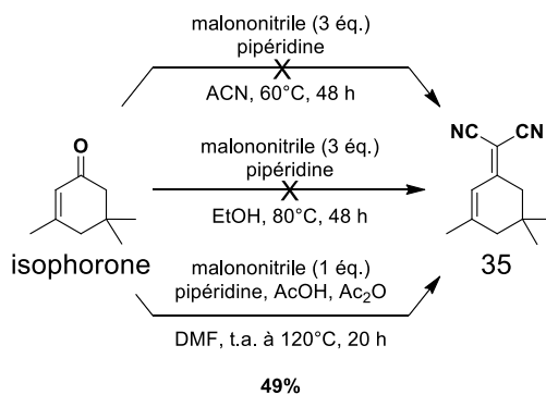
Schéma 23 : Conditions réactionnelles pour la synthèse de l'accepteur polynitrile 35 .
