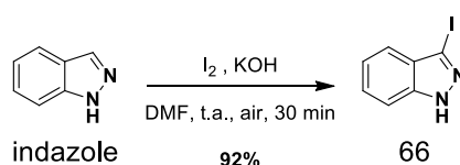
Schéma 39 : Synthèse du partenaire indazole pour la réaction de Heck.
