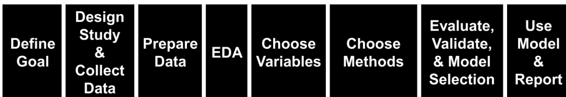
FIGURE 2.4: Etapes du processus de modélisation statistique (Shmueli, 2010)
