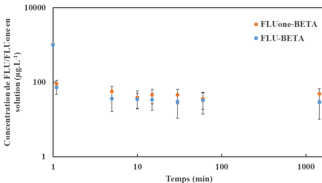
Figure IV-8. Cinétiques de sorption pour le FLU et la FLUone sur la zéolithe BETA, C_{FLU(0)} = 1\ 000\ \mu\text{g}\cdot\text{L}^{-1} et C_{FLUone(0)} = 1\ 000\ \mu\text{g}\cdot\text{L}^{-1}
