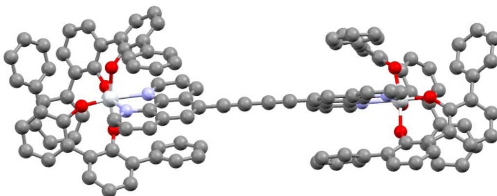
Figure 44 : Modèles moléculaires de a) \Delta,\Delta - [\text{Ti}_2(\mathbf{38})_4(\mathbf{49})] et b) \Lambda,\Lambda - [\text{Ti}_2(\mathbf{38})_4(\mathbf{49})] obtenus par calculs DFT dans le dichlorométhane (seul un conformère est représenté pour chaque stéréoisomère). Les atomes de titane sont représentés en blanc, les atomes de carbone en gris, les atomes d'oxygène en rouge et les atomes d'azote en violet. Les atomes d'hydrogène sont omis par souci de clarté.
