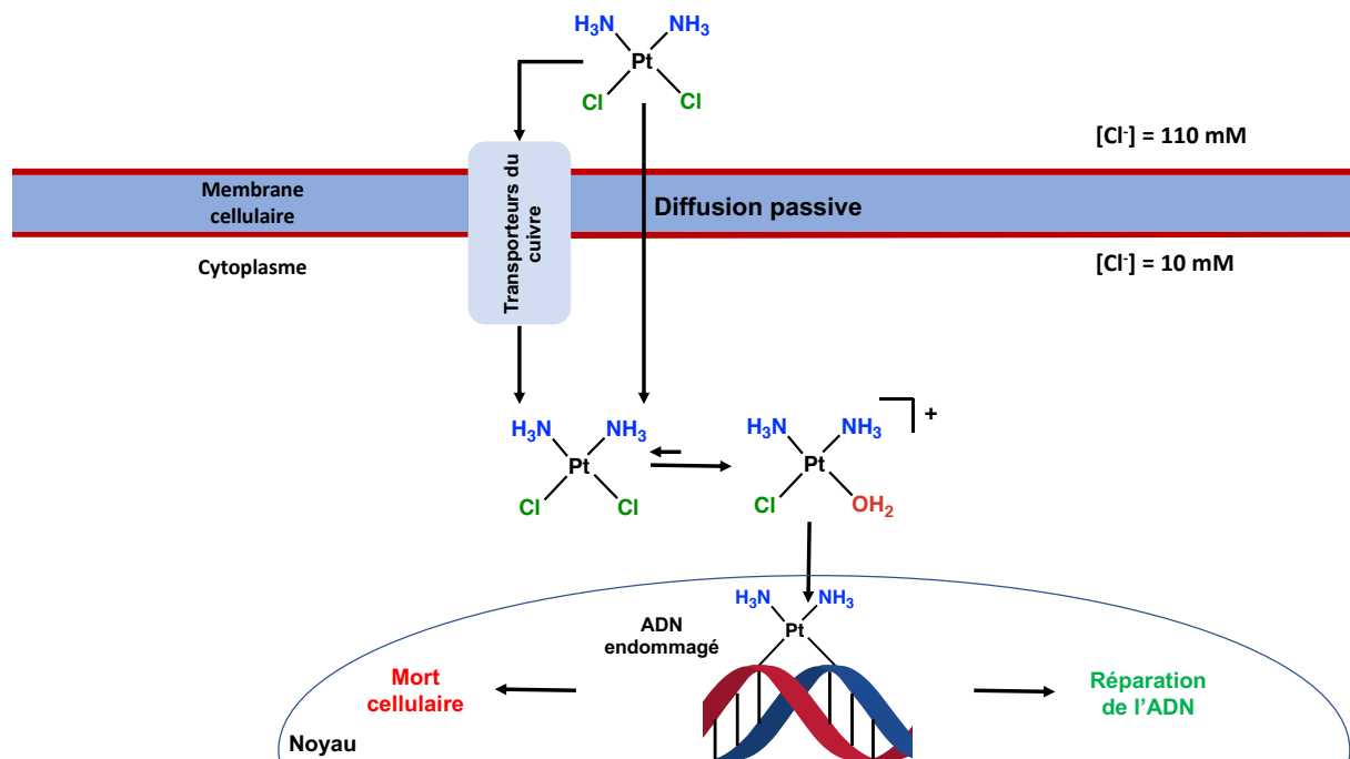
Figure 68 : Mode d'action du cisplatine. Après pénétration dans le noyau cellulaire, l'adduit crée par coordination à l'ADN est soit réparé par les protéines chargées de la réparation de l'ADN lors de la réplication cellulaire, ou bien, si la réparation n'est pas possible, provoque la mort cellulaire.
