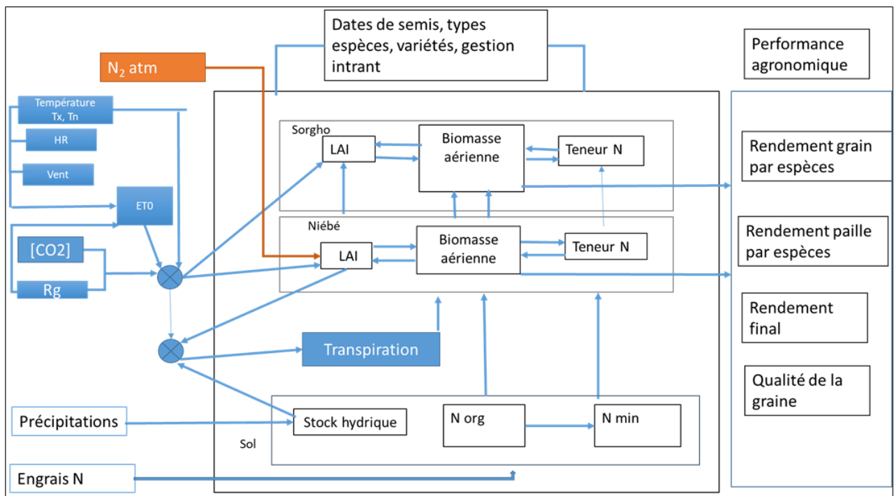
Figure 1 : Schéma conceptuel du fonctionnement de l'association sorgho-niébé. N 2 atm = azote atmosphérique, Tx = température maximale, tn = température minimale, Rg = rayonnement global, ETO = évapotranspiration de référence, N = azote.
