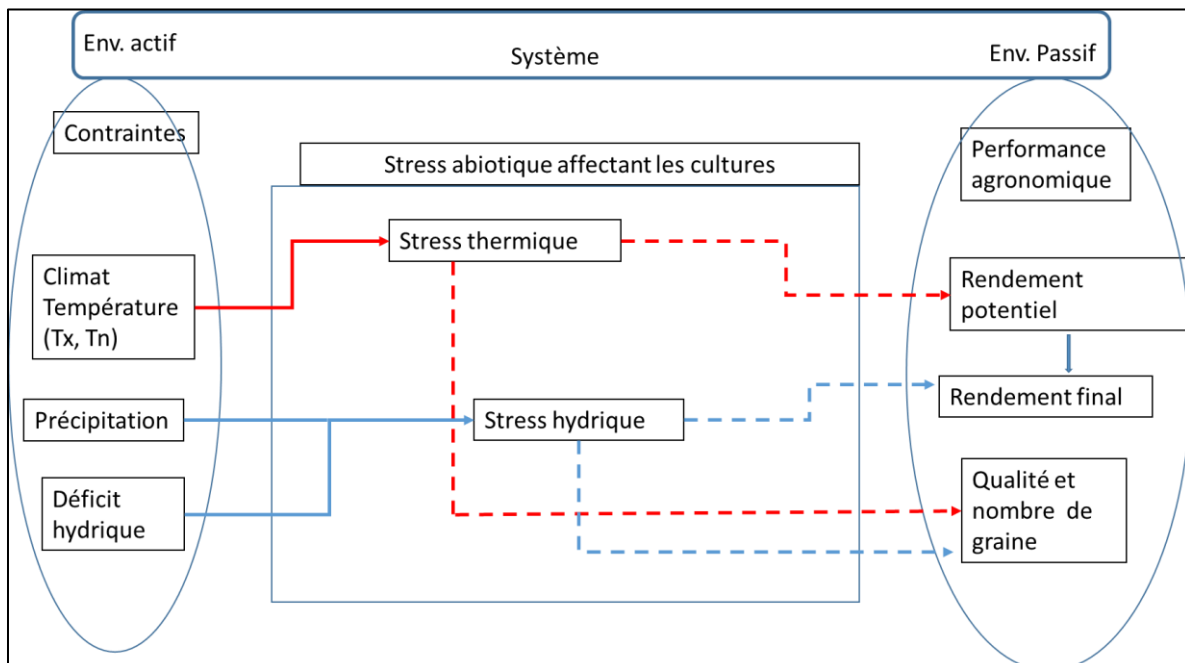
Figure2 : Schéma conceptuel du stress induits à l'élaboration de la biomasse. Tx = température maximale, tn = température minimale, Rg = rayonnement global, Env. actif = environnement actif, Env. passif = Environnement passif.
